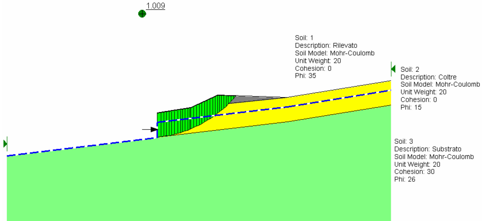
Figura 6.3- Analisi limite per la valutazione dell'azione che stabilizza il cuneo di monte con FS=1.0 nelle condizioni iniziali
