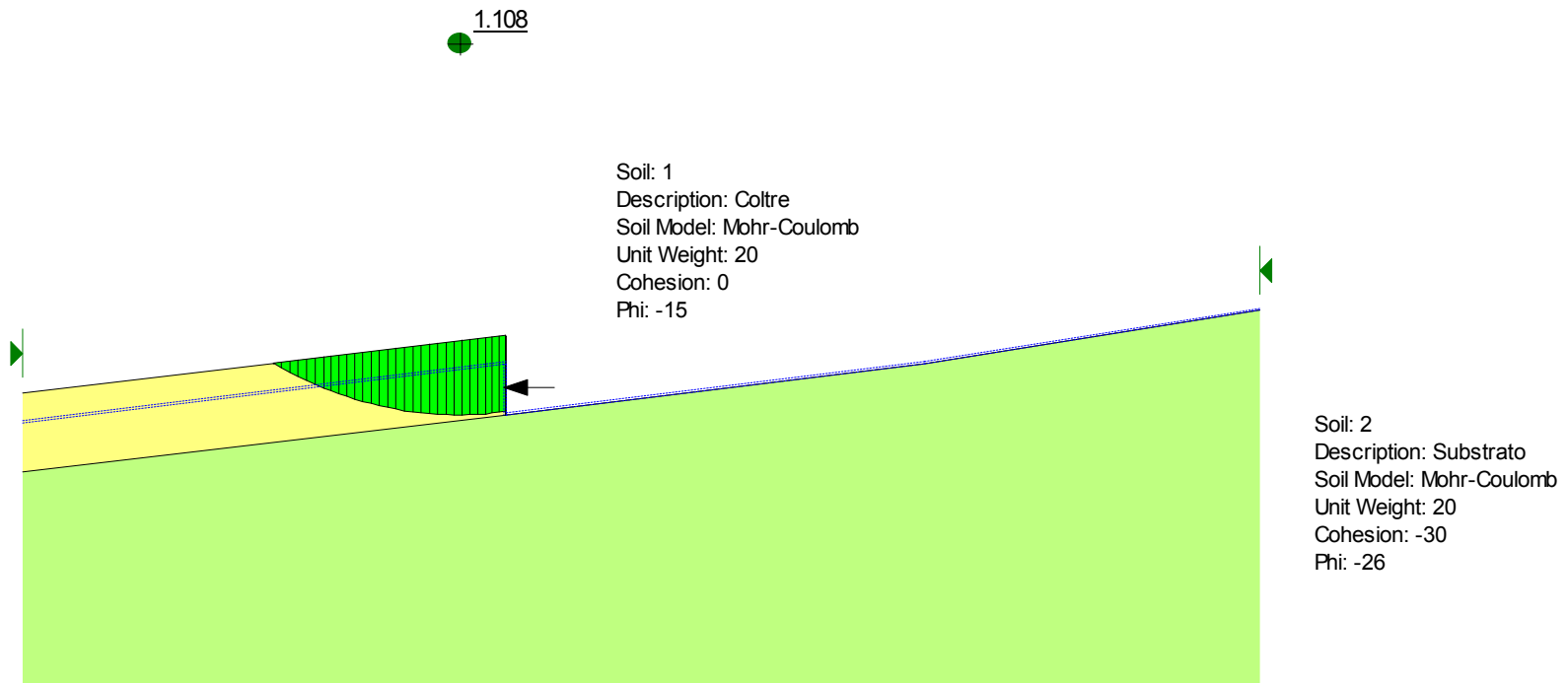
Figura 6.7- Analisi limite per la valutazione dell'azione che instabilizza il cuneo di valle con FS=1.1 nelle condizioni finali
