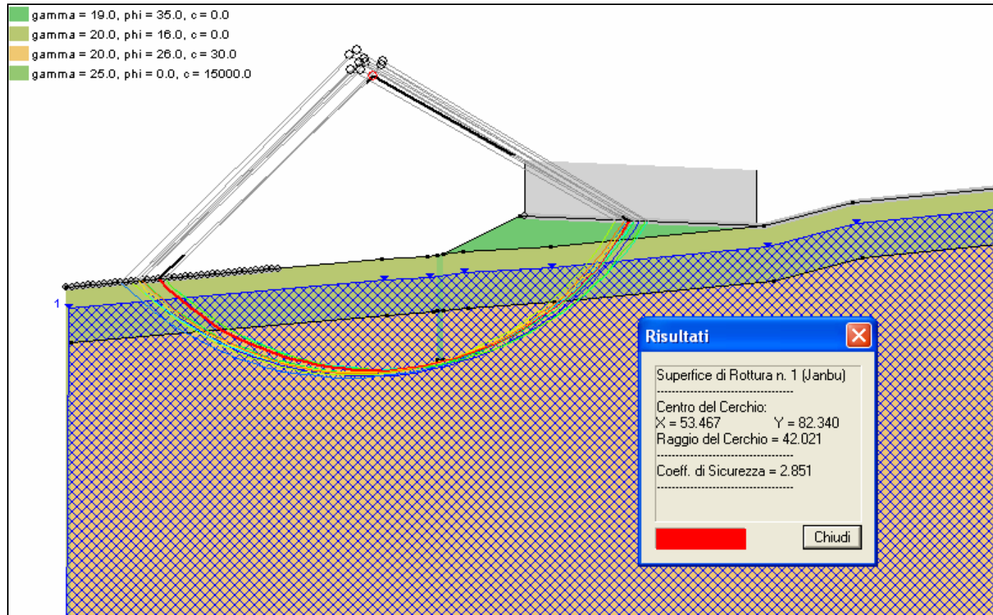
Figura 7.1- Analisi di stabilità globale nel caso statico ed individuazione della superficie di scorrimento avente Fs minimo
