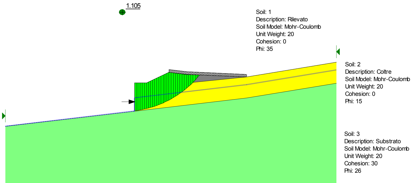
Figura 6.6- Analisi limite per la valutazione dell'azione che stabilizza il cuneo di monte con FS=1.1 nelle condizioni finali
