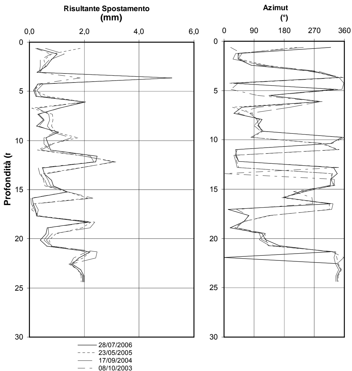
Figura 3.2 Grafici delle letture inclinometro I103
