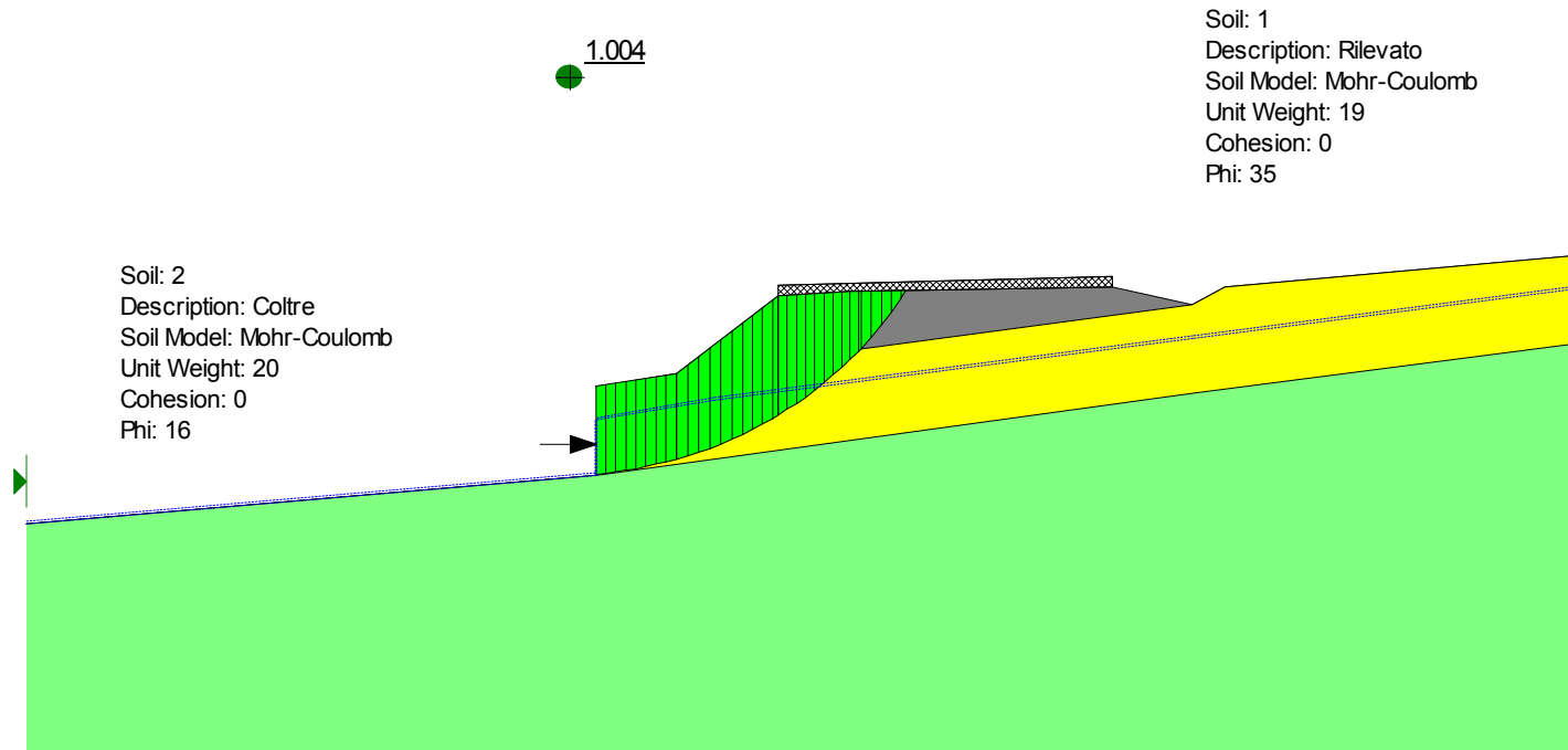
Figura 6.3- Analisi limite per la valutazione dell'azione che stabilizza il cuneo di monte con FS=1.0 nelle condizioni iniziali
