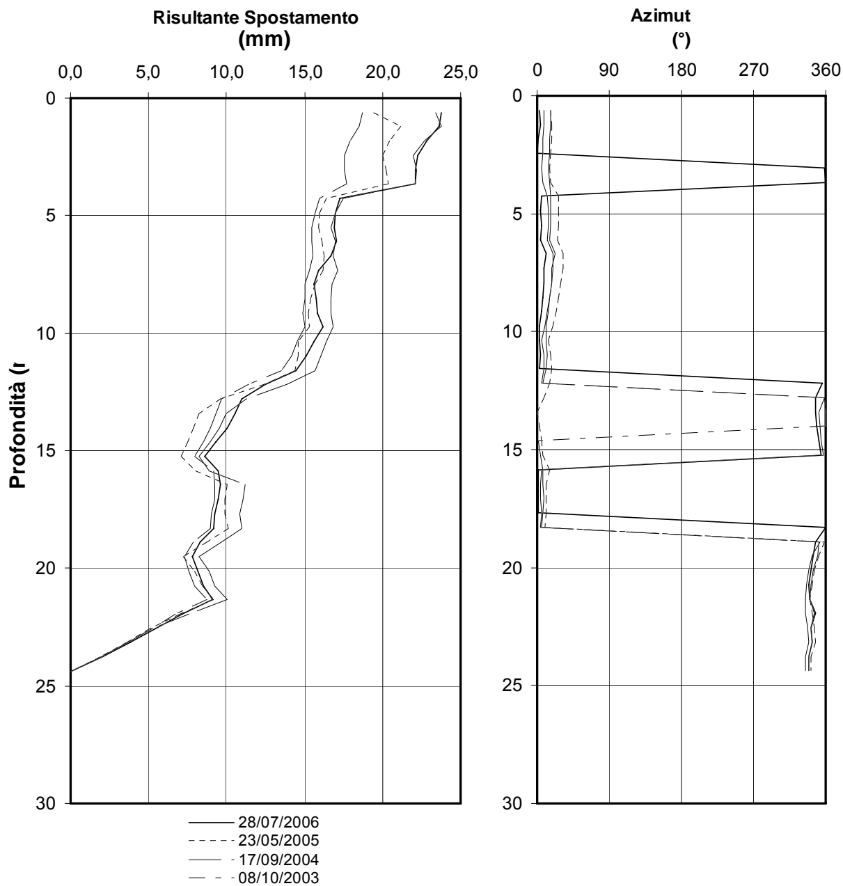
Figura 3.1 Grafici delle letture inclinometro I103
