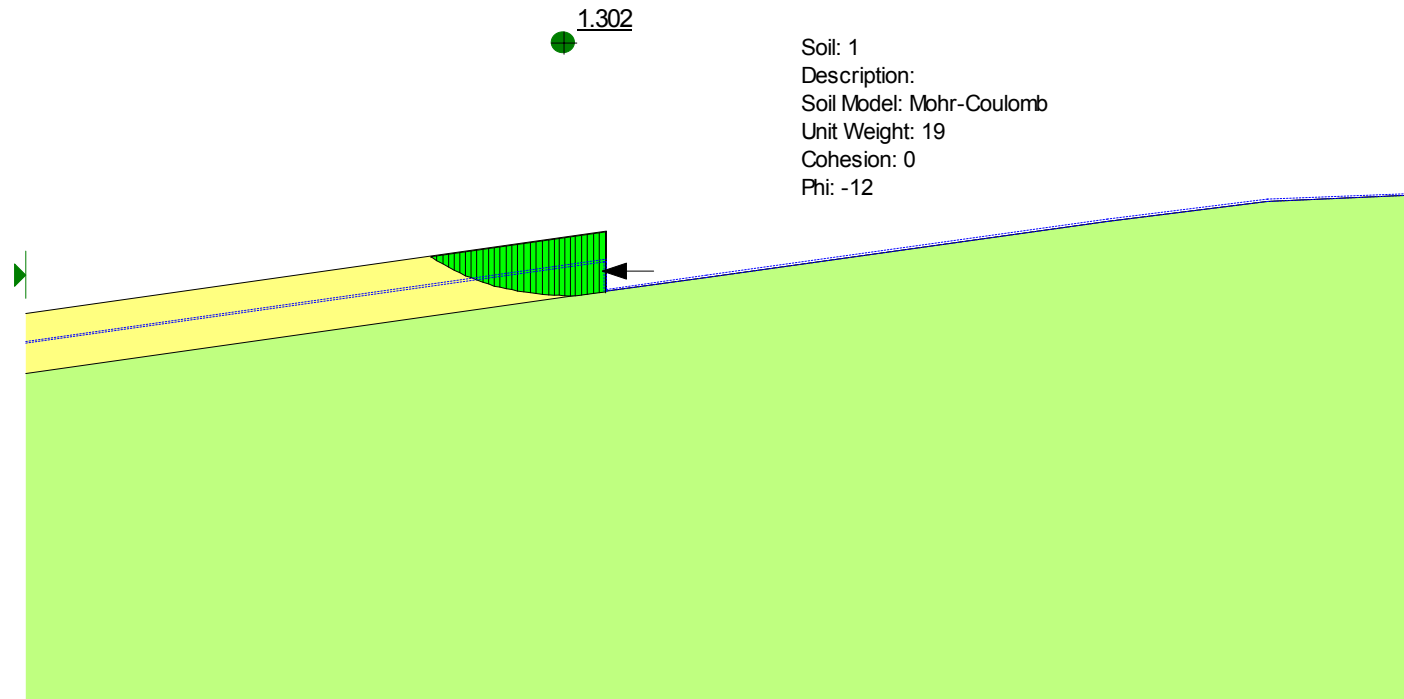
Figura 6.9- Analisi limite per la valutazione dell'azione che instabilizza il cuneo di valle con FS=1.3 nelle condizioni finali
