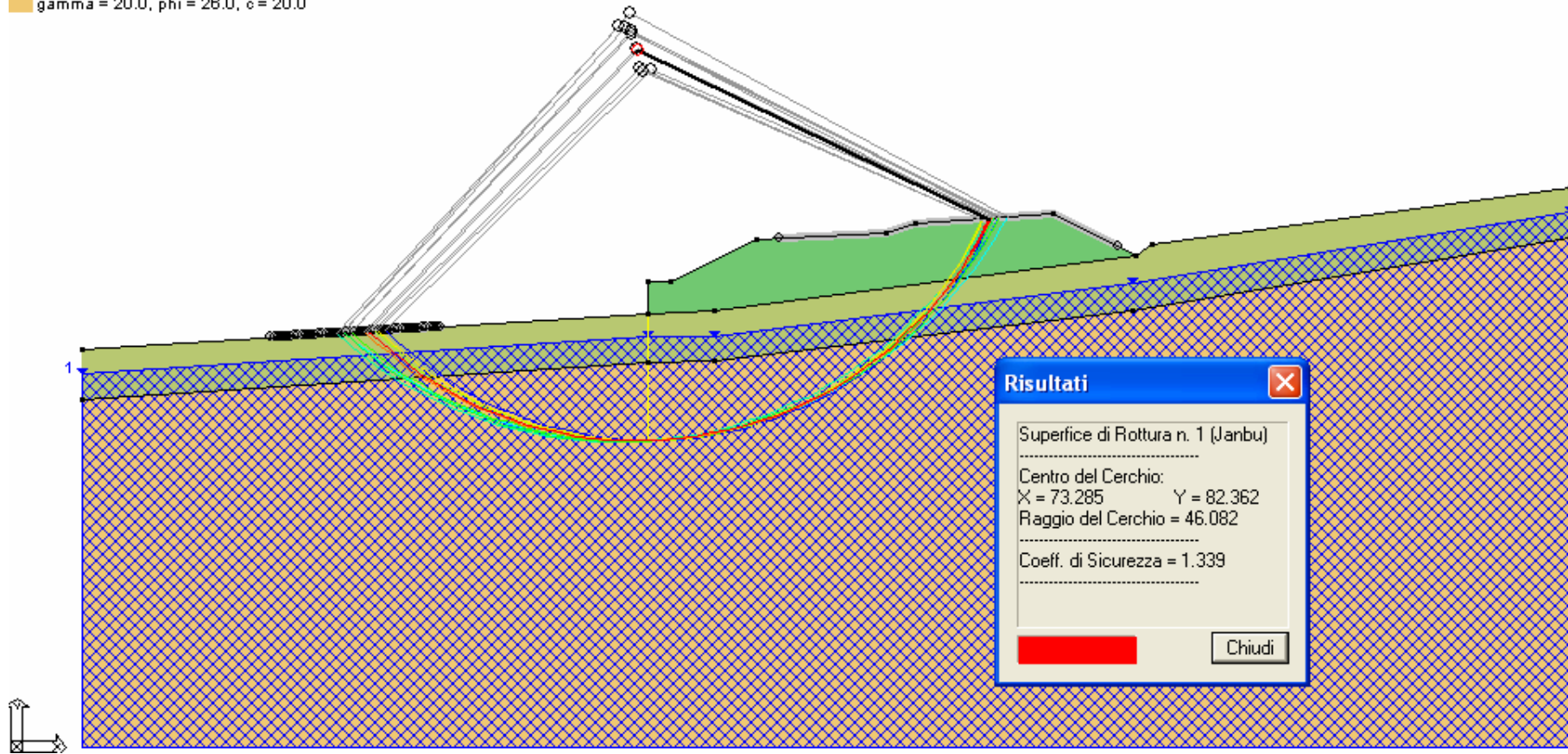
Figura 7.2- Analisi di stabilità globale nel caso sismico ed individuazione della superficie di scorrimento avente F_s minimo
