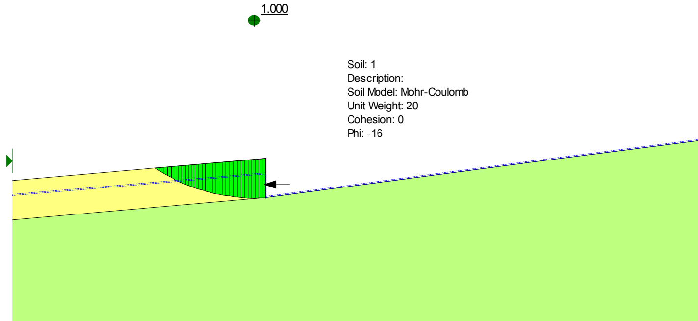
Figura 6.4- Analisi limite per la valutazione dell'azione che instabilizza il cuneo di valle con FS = 1.0 nelle condizioni iniziali
