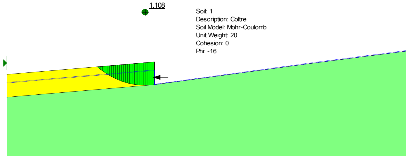
Figura 6.7- Analisi limite per la valutazione dell'azione che instabilizza il cuneo di valle con FS=1.1 nelle condizioni finali
