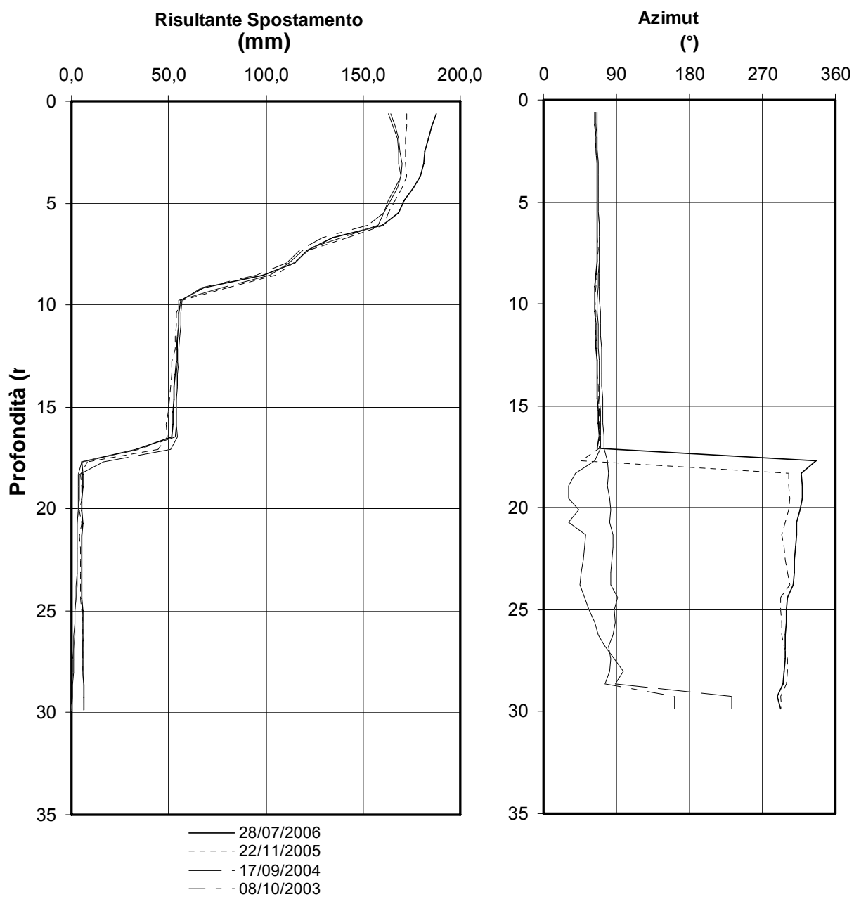
Figura 3.1 Grafici delle letture inclinometro I9
