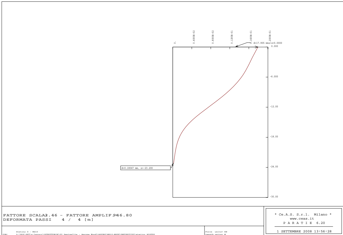
Figura 6.11- Programma PARATIE – Spostamenti in fase di esercizio
