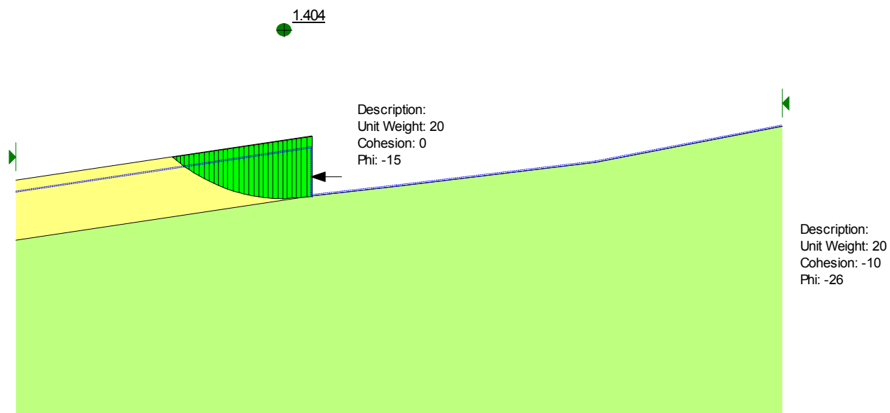
Figura 6.9- Analisi limite per la valutazione dell'azione che instabilizza il cuneo di valle con FS=1.4 nelle condizioni finali
