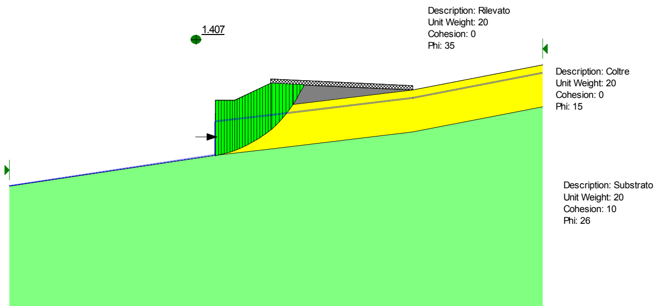
Figura 6.8- Analisi limite per la valutazione dell'azione che stabilizza il cuneo di monte con FS=1.4 nelle condizioni finali
