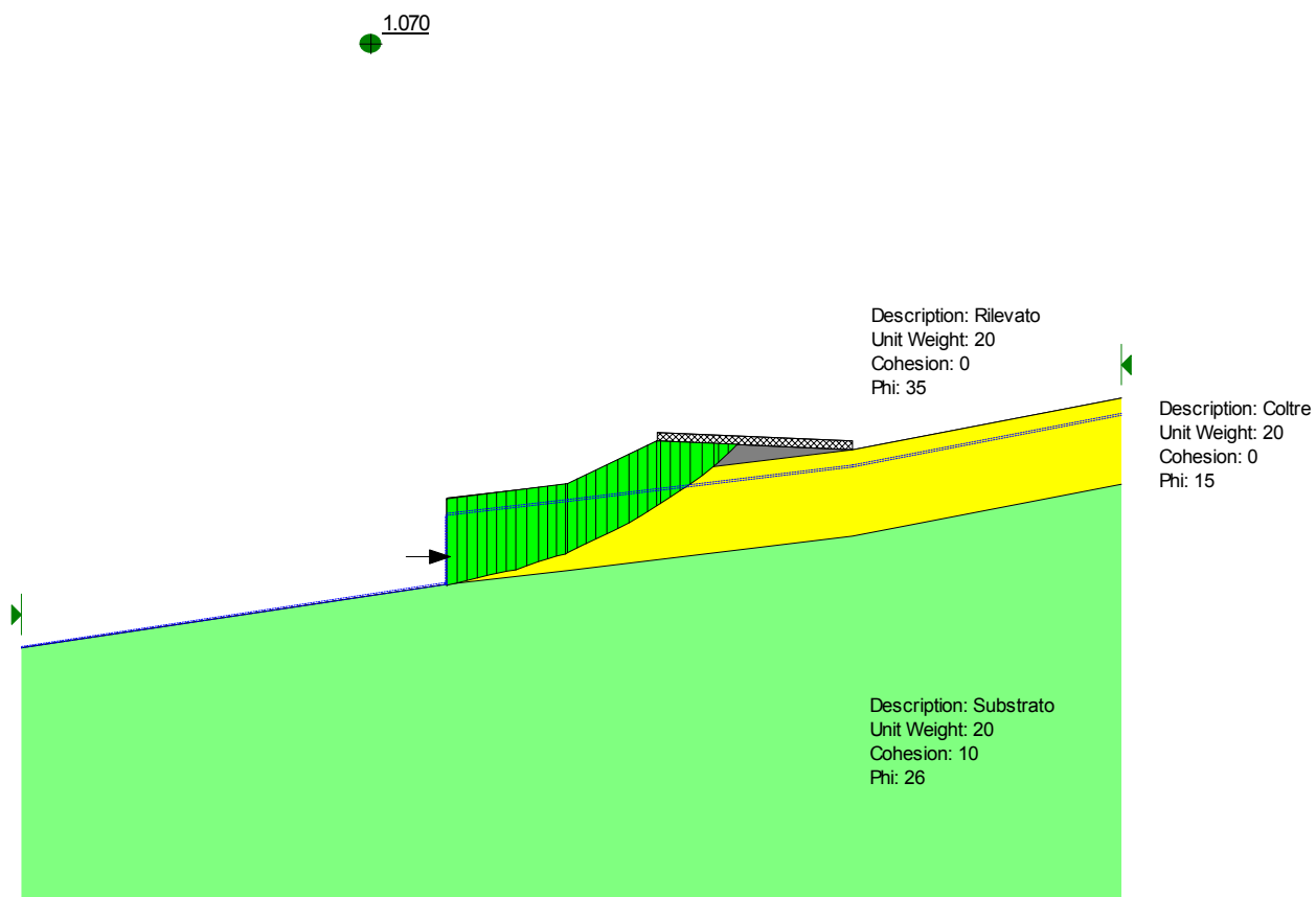
Figura 6.3- Analisi limite per la valutazione dell'azione che stabilizza il cuneo di monte con FS=1.0 nelle condizioni iniziali
