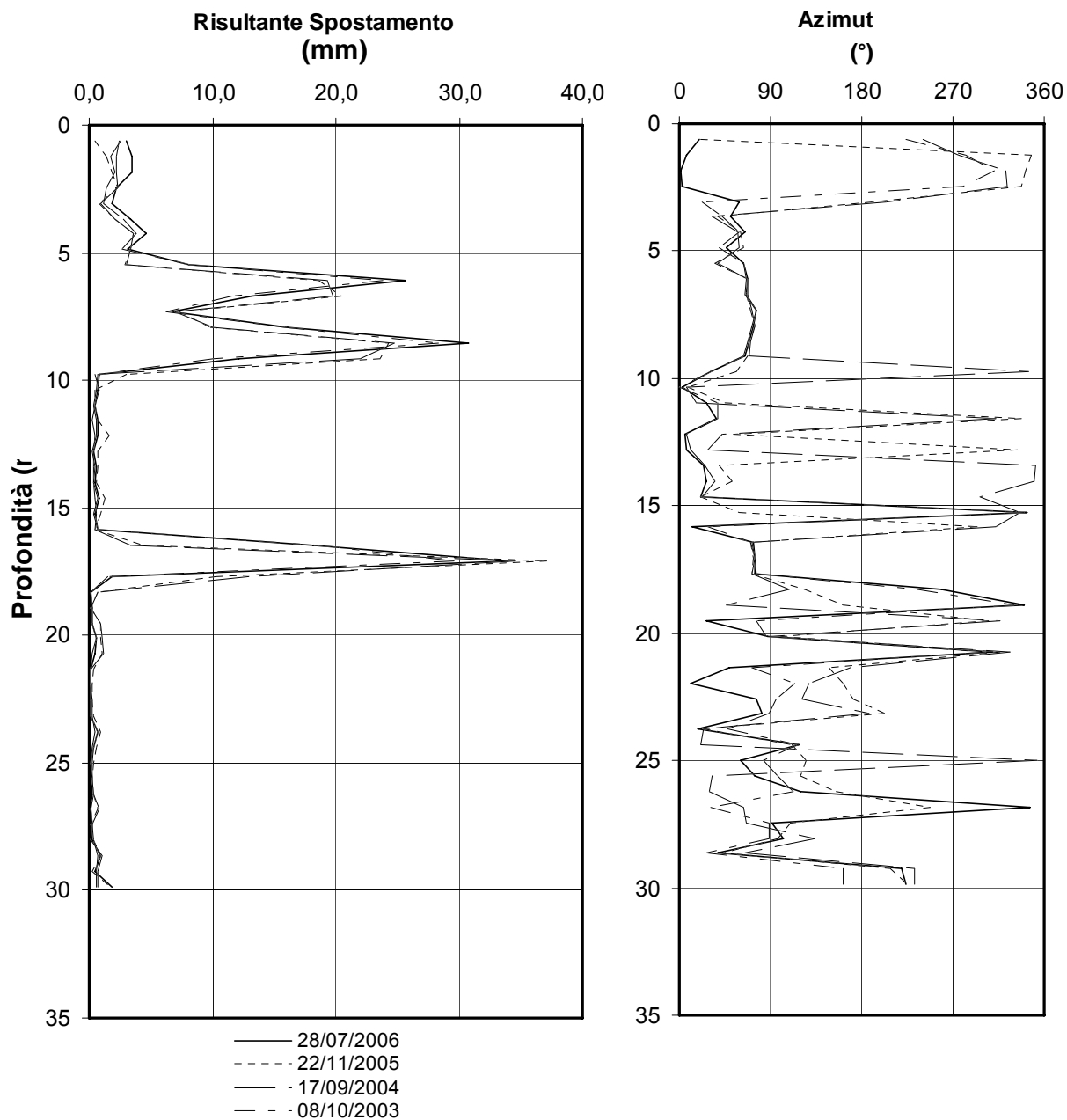
Figura 3.2 Grafici delle letture inclinometro I9
