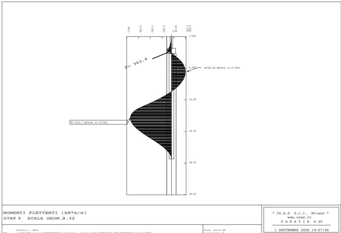
Figura 6.20- Programma PARATIE – Fase SLU Sisma – Momento flettente
