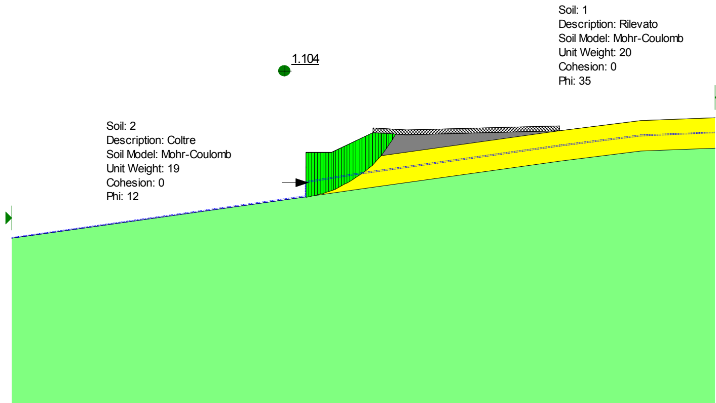
Figura 6.6- Analisi limite per la valutazione dell'azione che stabilizza il cuneo di monte con FS=1.1 nelle condizioni finali
