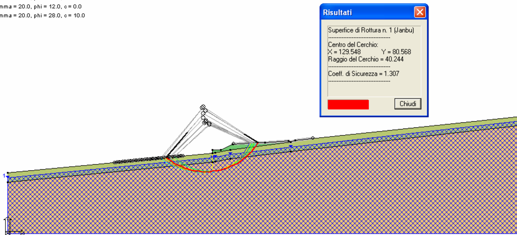
Figura 7.2- Analisi di stabilità globale nel caso sismico ed individuazione della superficie di scorrimento avente F_s minimo
