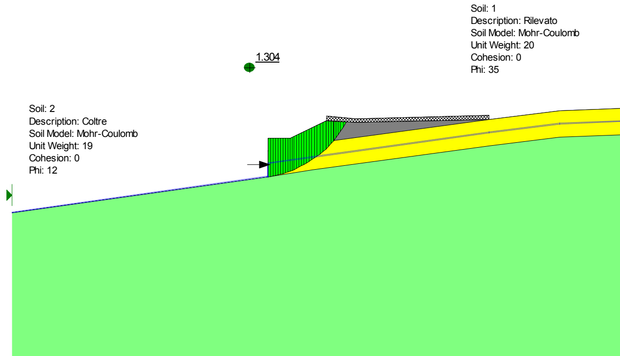
Figura 6.8- Analisi limite per la valutazione dell'azione che stabilizza il cuneo di monte con FS=1.3 nelle condizioni finali
