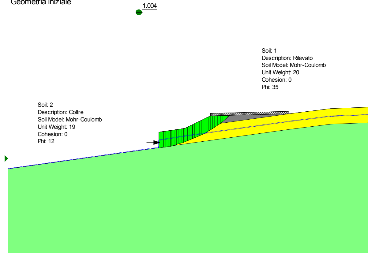
Figura 6.3- Analisi limite per la valutazione dell'azione che stabilizza il cuneo di monte con FS=1.0 nelle condizioni iniziali
