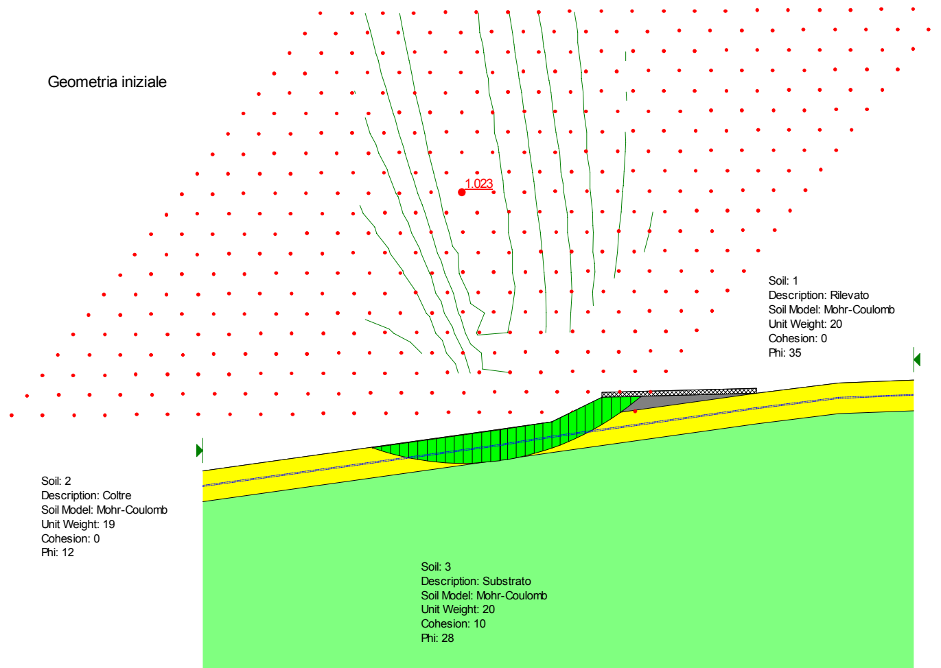
Figura 6.2- Analisi limite nelle condizioni iniziali per la definizione della superficie di rottura critica
