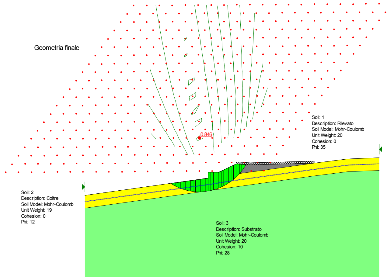
Figura 6.5- Analisi limite nelle condizioni finali per la definizione della superficie di rottura critica
