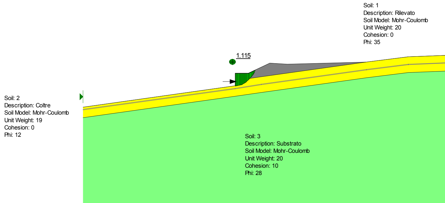
Figura 6.10 - Analisi limite per la valutazione dell'azione sismica con FS=1.1 nelle condizioni finali
