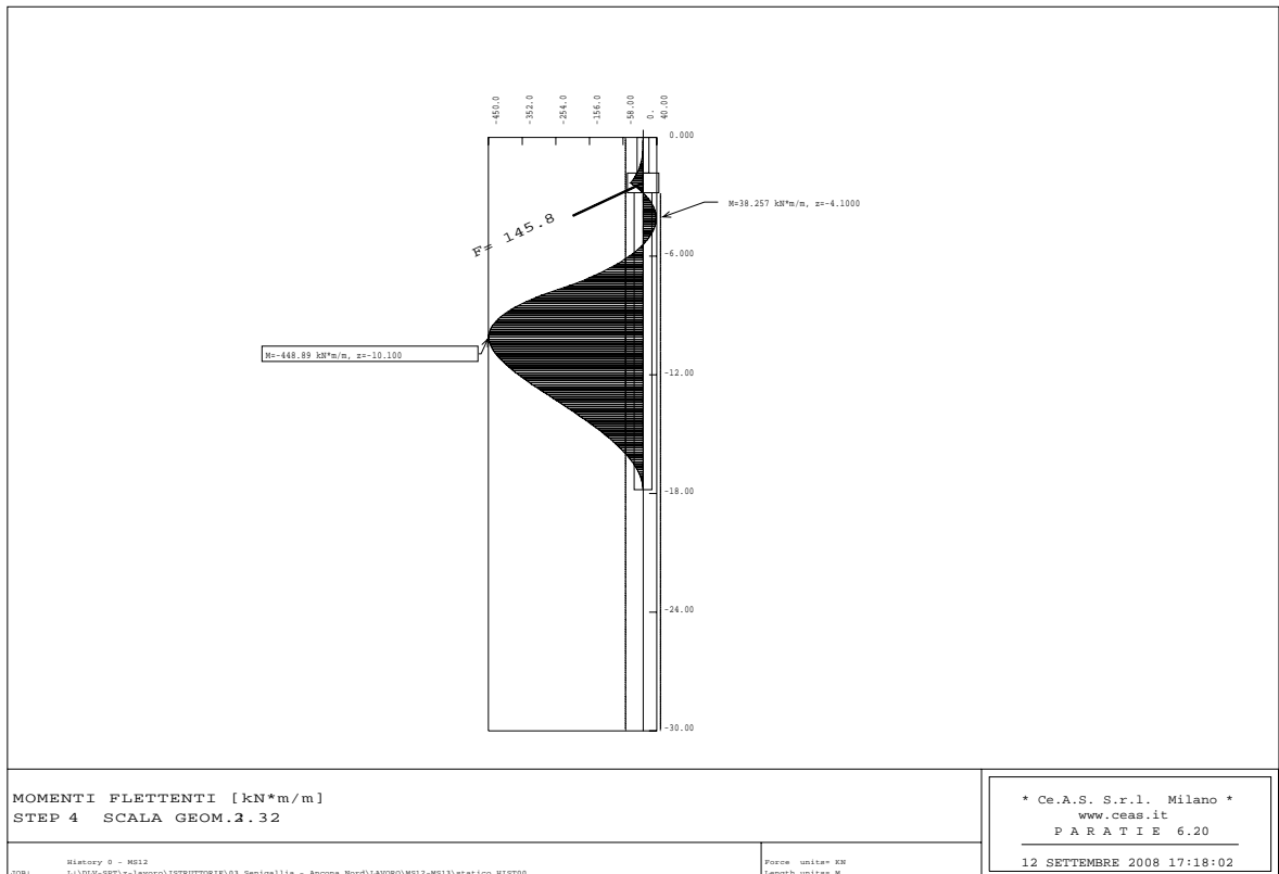
Figura 6.17 - Programma PARATIE – Fase di esercizio – Momento flettente
