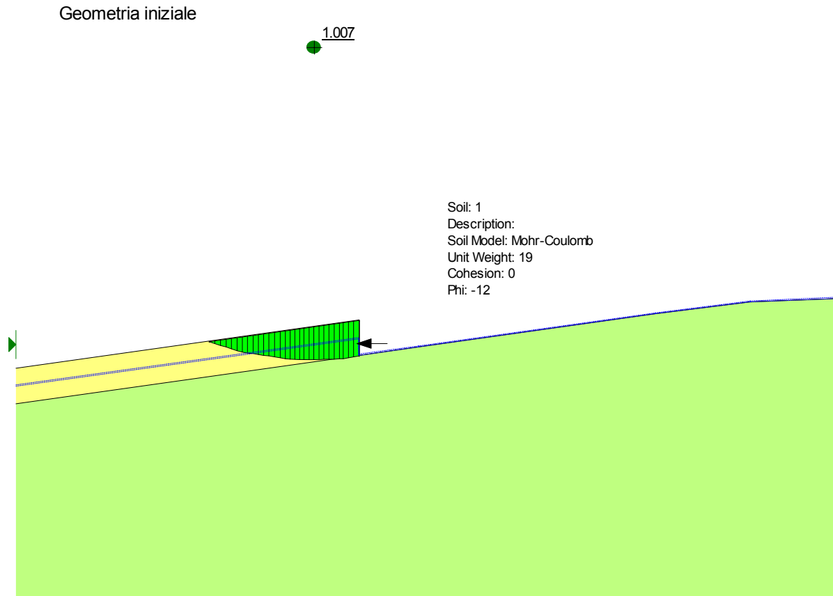
Figura 6.4- Analisi limite per la valutazione dell'azione che instabilizza il cuneo di valle con FS = 1.0 nelle condizioni iniziali
