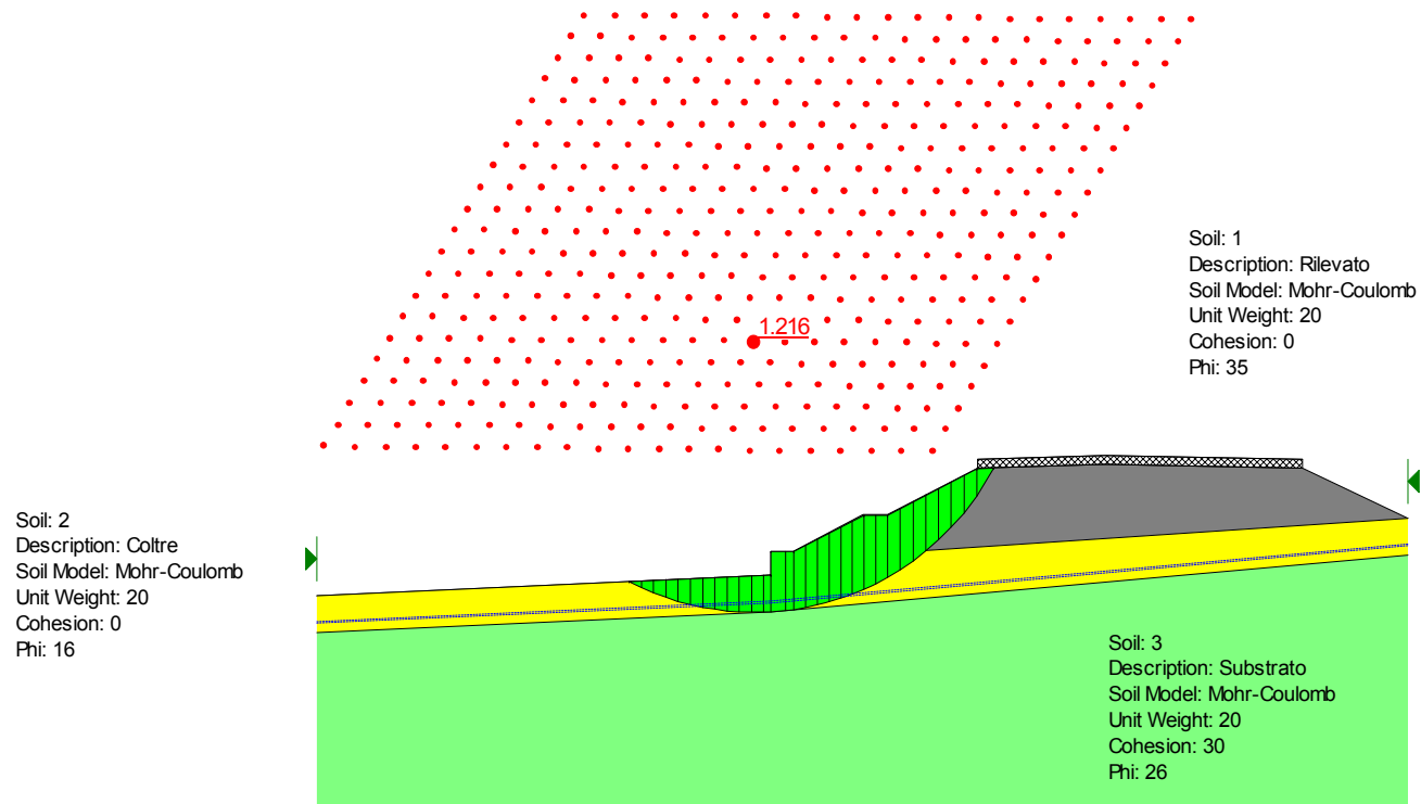
Figura 6.3- Analisi limite nelle condizioni finali per la definizione della superficie di rottura critica
