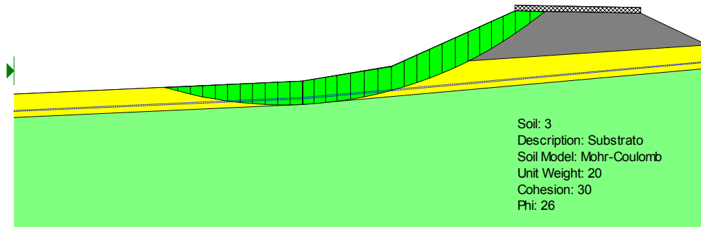
Figura 6.2- Analisi limite nelle condizioni iniziali per la definizione della superficie di rottura critica
