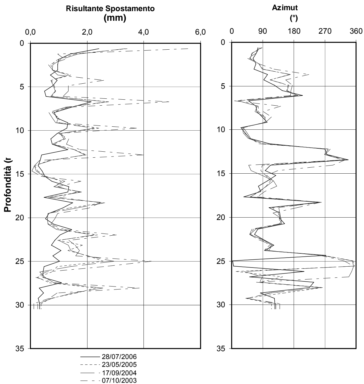
Figura 3.2 Grafici delle letture inclinometro I111
