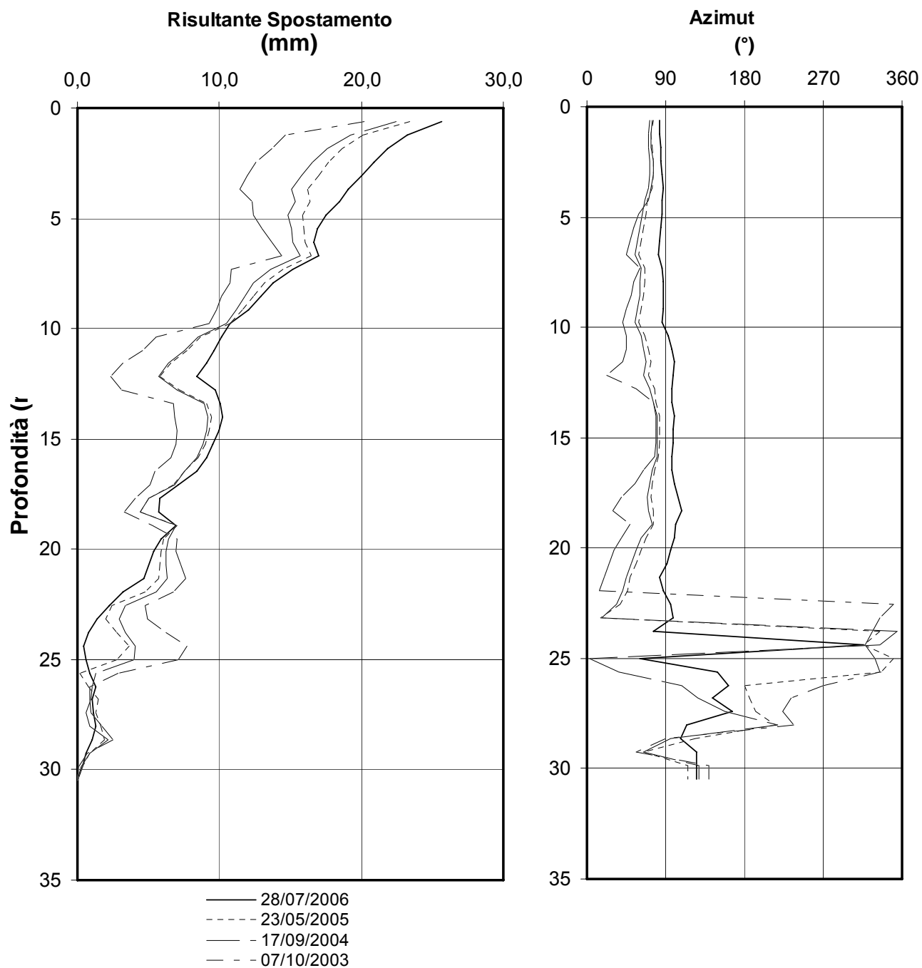
Figura 3.1 Grafici delle letture inclinometro I111
