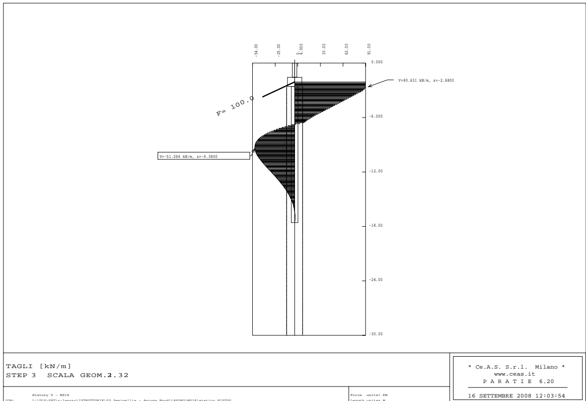
Figura 6.16 - Programma PARATIE – Fasi costruttive – Taglio
