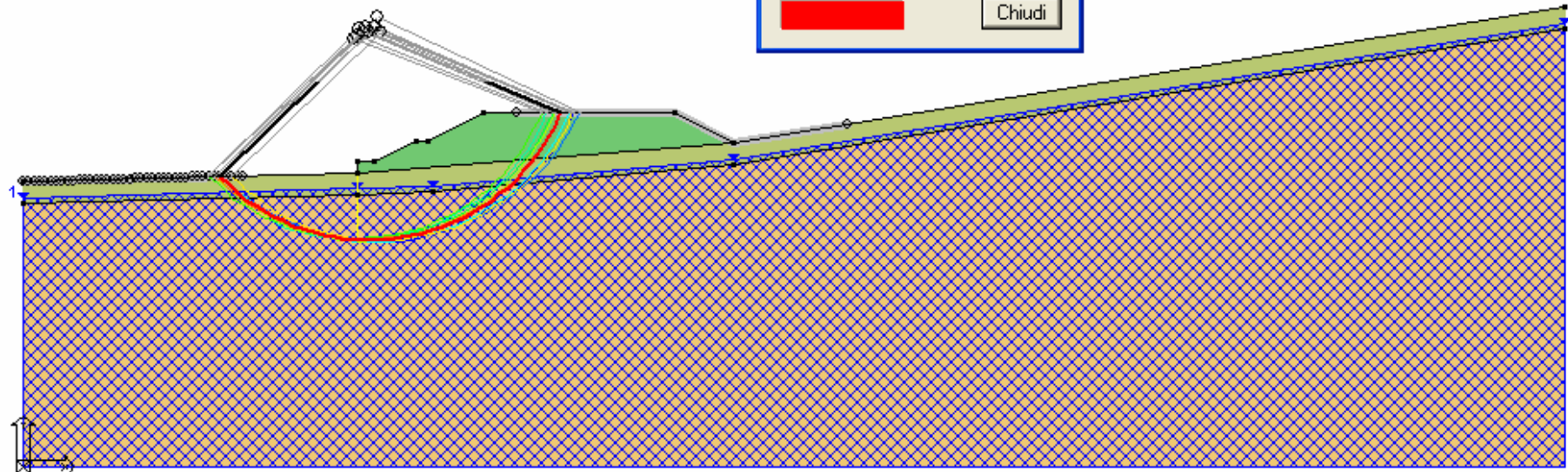
Figura 7.2- Analisi di stabilità globale nel caso sismico ed individuazione della superficie di scorrimento avente Fs minimo
