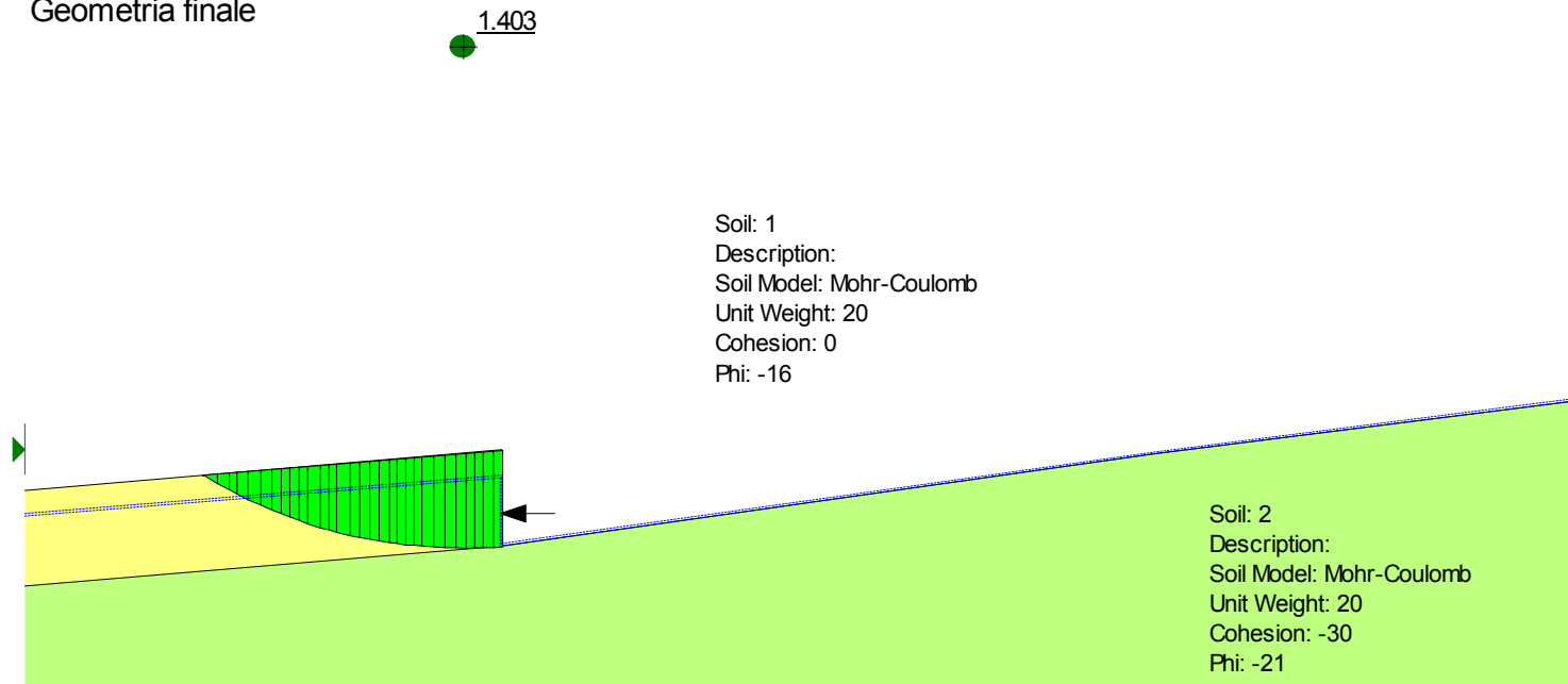
Figura 6.9- Analisi limite per la valutazione dell'azione che instabilizza il cuneo di valle con FS=1.4 nelle condizioni finali
