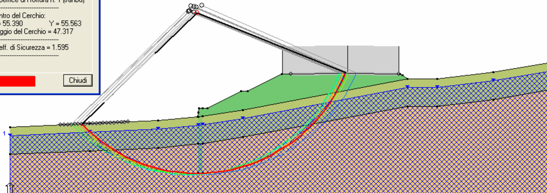
Figura 7.1- Analisi di stabilità globale nel caso statico ed individuazione della superficie di scorrimento avente Fs minimo
