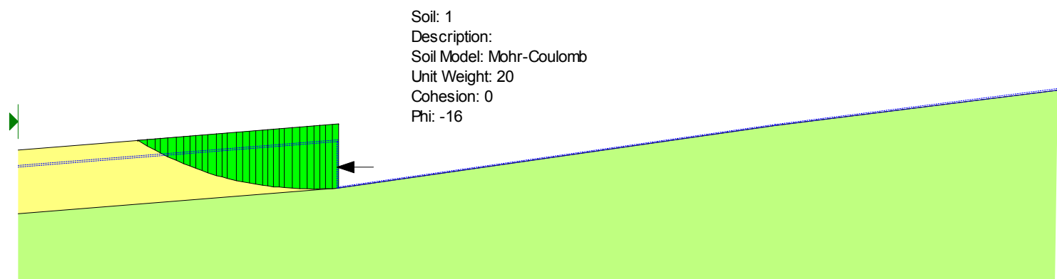
Figura 6.7- Analisi limite per la valutazione dell'azione che instabilizza il cuneo di valle con FS=1.1 nelle condizioni finali
