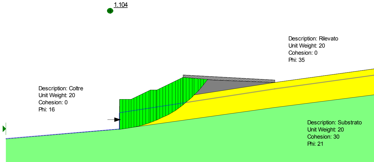
Figura 6.6- Analisi limite per la valutazione dell'azione che stabilizza il cuneo di monte con FS=1.1 nelle condizioni finali
