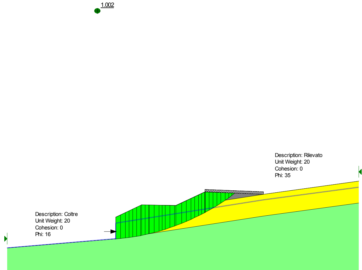
Figura 6.3- Analisi limite per la valutazione dell'azione che stabilizza il cuneo di monte con FS=1.0 nelle condizioni iniziali
