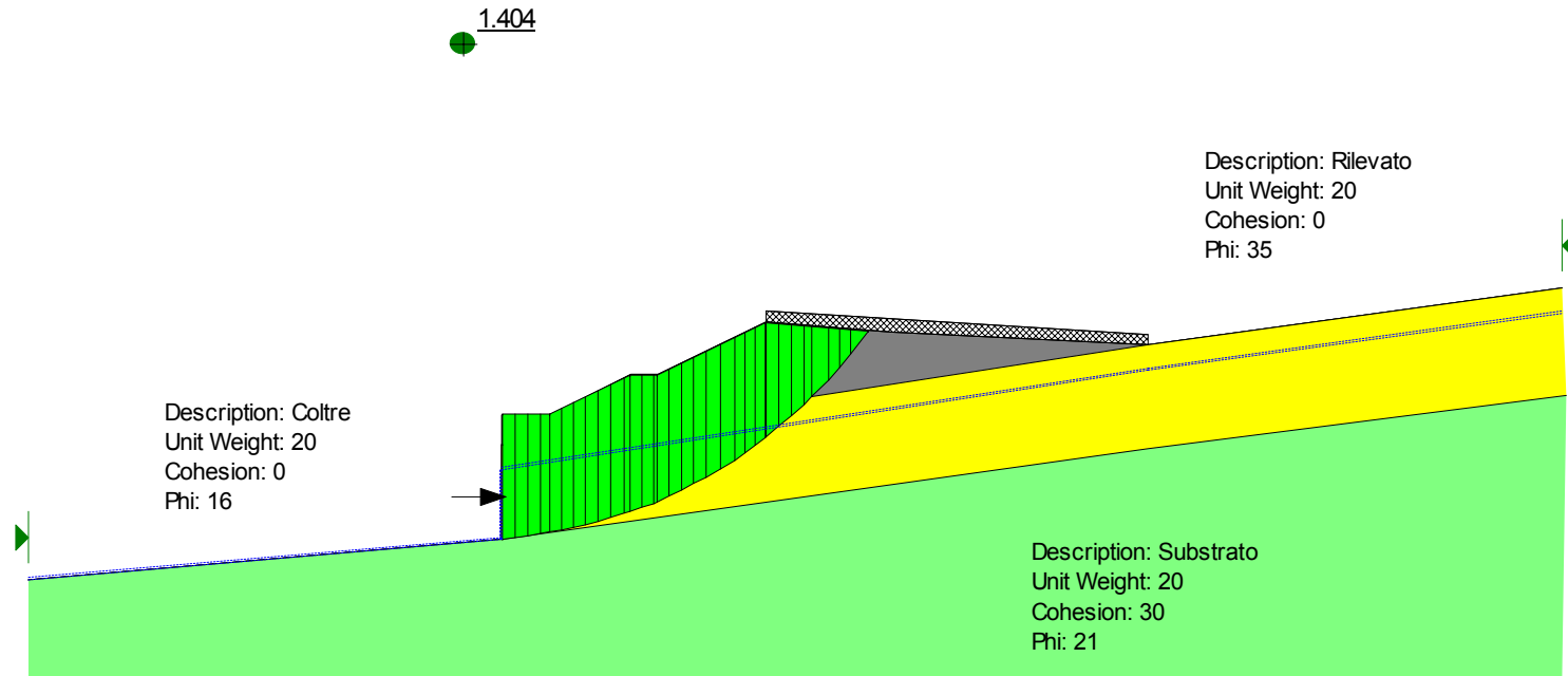
Figura 6.8- Analisi limite per la valutazione dell'azione che stabilizza il cuneo di monte con FS=1.4 nelle condizioni finali
