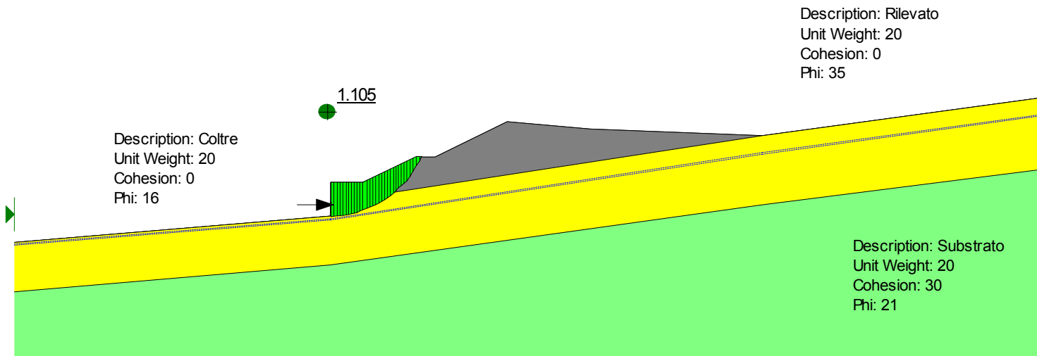
Figura 6.10 - Analisi limite per la valutazione dell'azione sismica con FS=1.1 nelle condizioni finali
