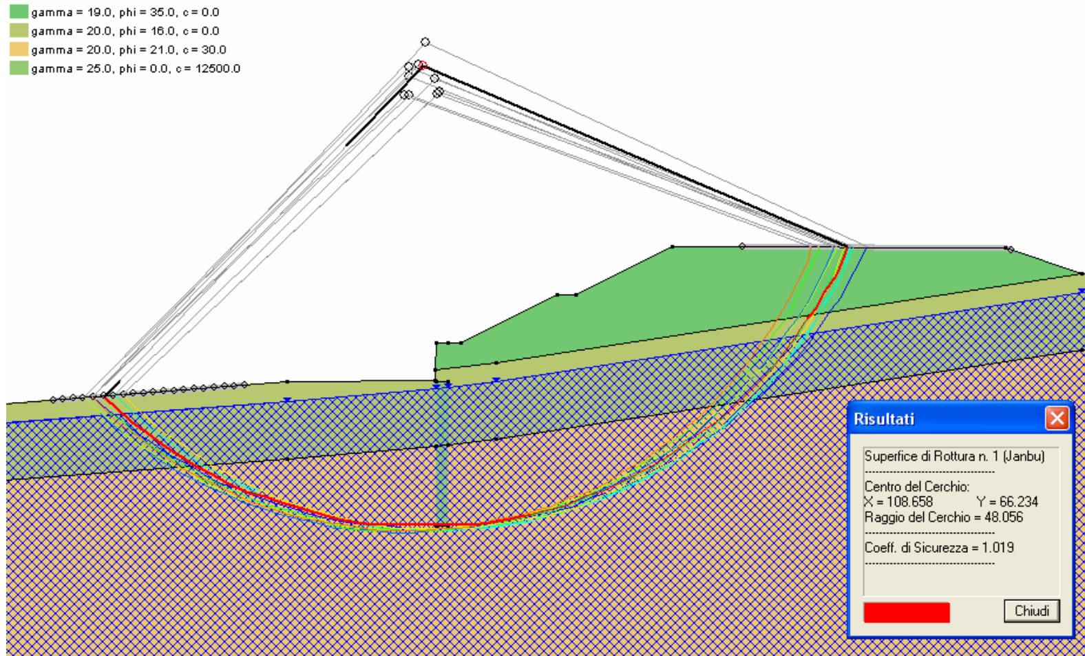
Figura 7.2- Analisi di stabilità globale nel caso sismico ed individuazione della superficie di scorrimento avente Fs minimo
