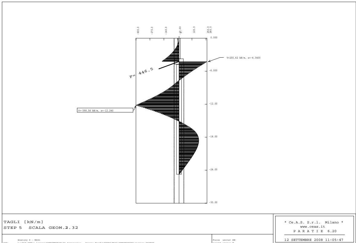
Figura 6.19 - Programma PARATIE – Fase SLU FS NEW – Taglio
