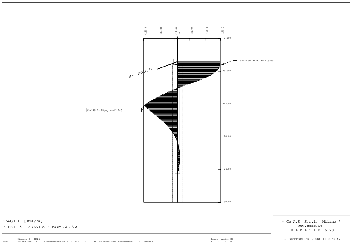
Figura 6.15 - Programma PARATIE – Fasi costruttive – Taglio
