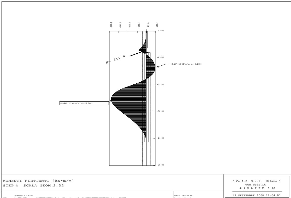
Figura 6.16 - Programma PARATIE – Fase di esercizio – Momento flettente
