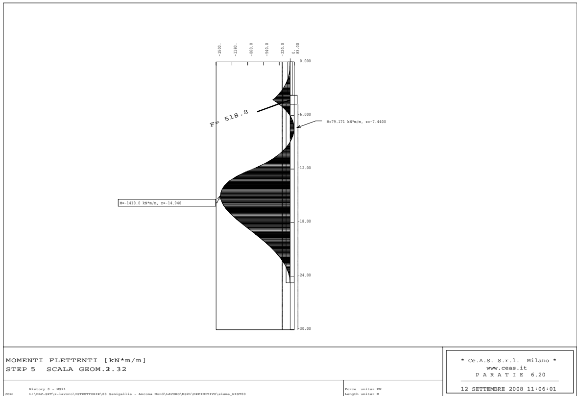
Figura 6.20 - Programma PARATIE – Fase SLU Sisma – Momento flettente
