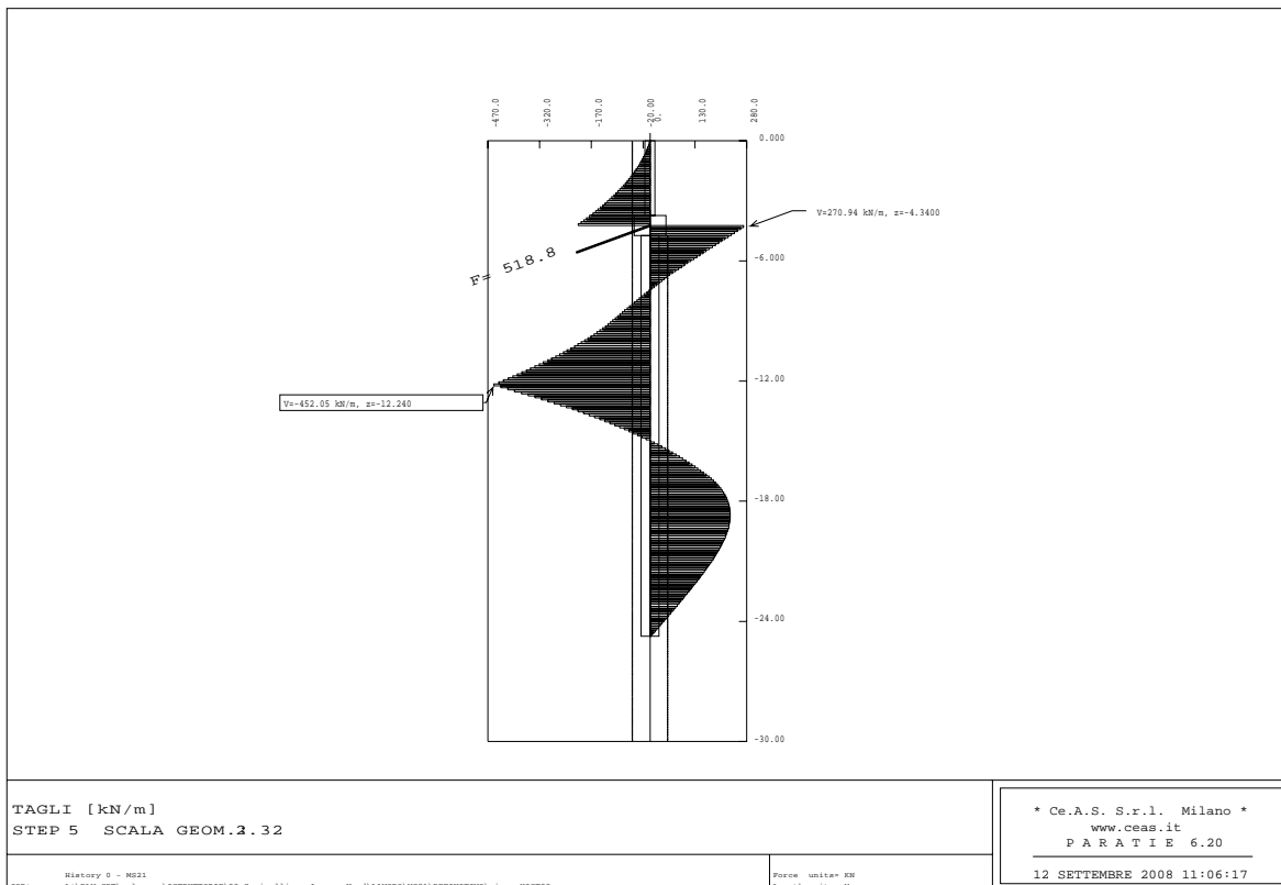
Figura 6.21 - Programma PARATIE – Fase SLU Sisma – Taglio
