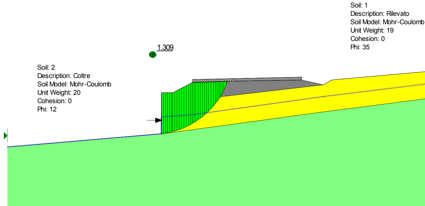
Figura 6.8- Analisi limite per la valutazione dell'azione che stabilizza il cuneo di monte con FS=1.3 nelle condizioni finali
