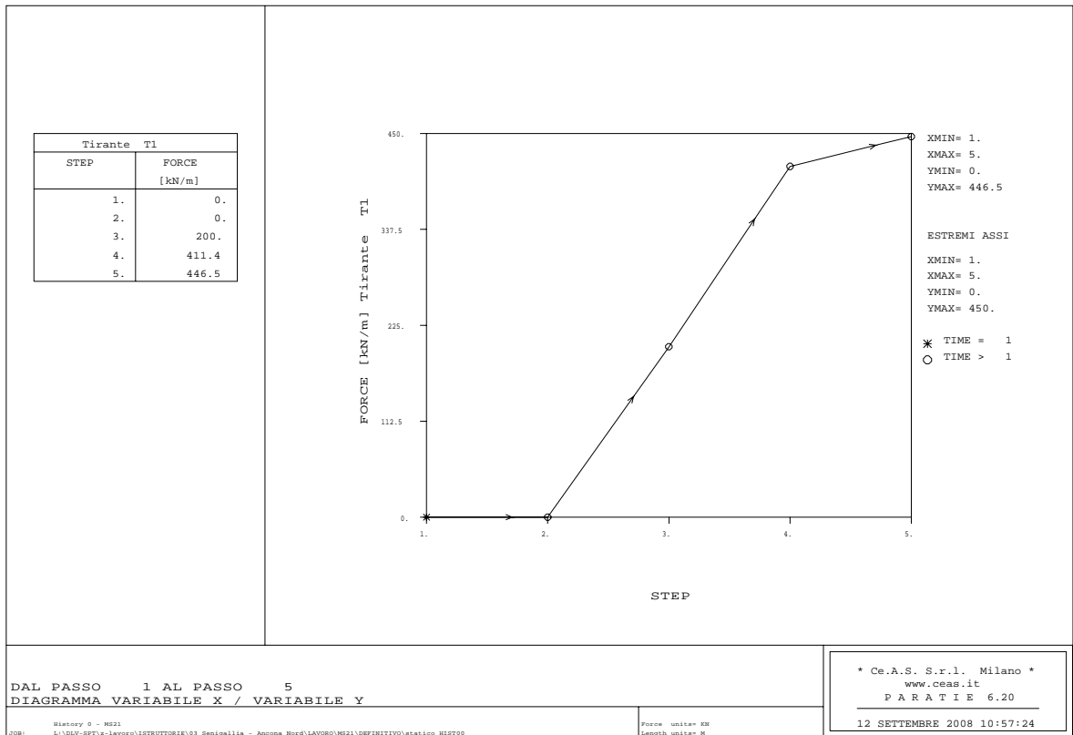
Figura 6.12 - Programma PARATIE – Tiro nel tirante – Caso statico
