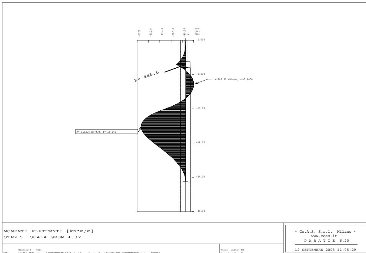
Figura 6.18 - Programma PARATIE – Fase SLU FS NEW – Momento flettente
