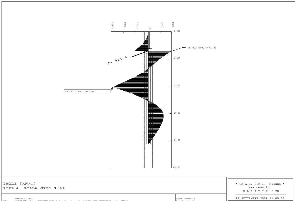
Figura 6.17 - Programma PARATIE – Fase di esercizio - Taglio
