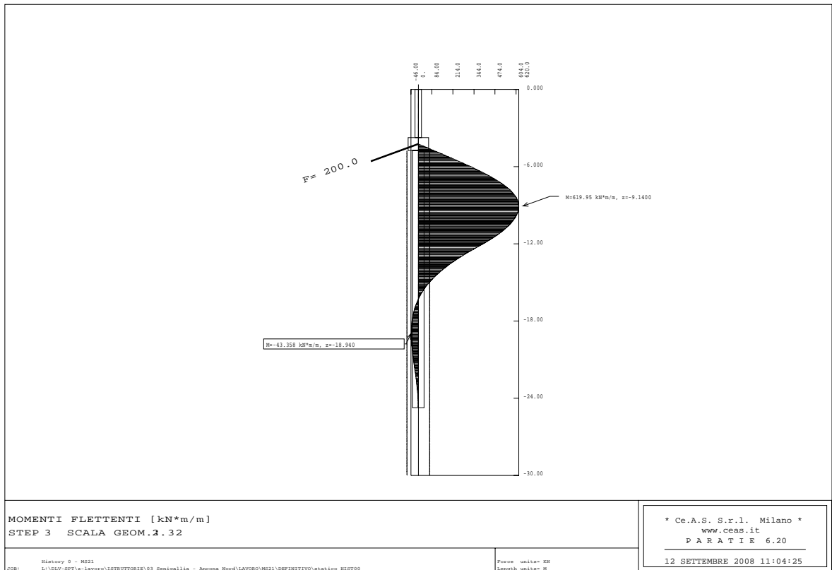
Figura 6.14 - Programma PARATIE – Fasi costruttive – Momento flettente
