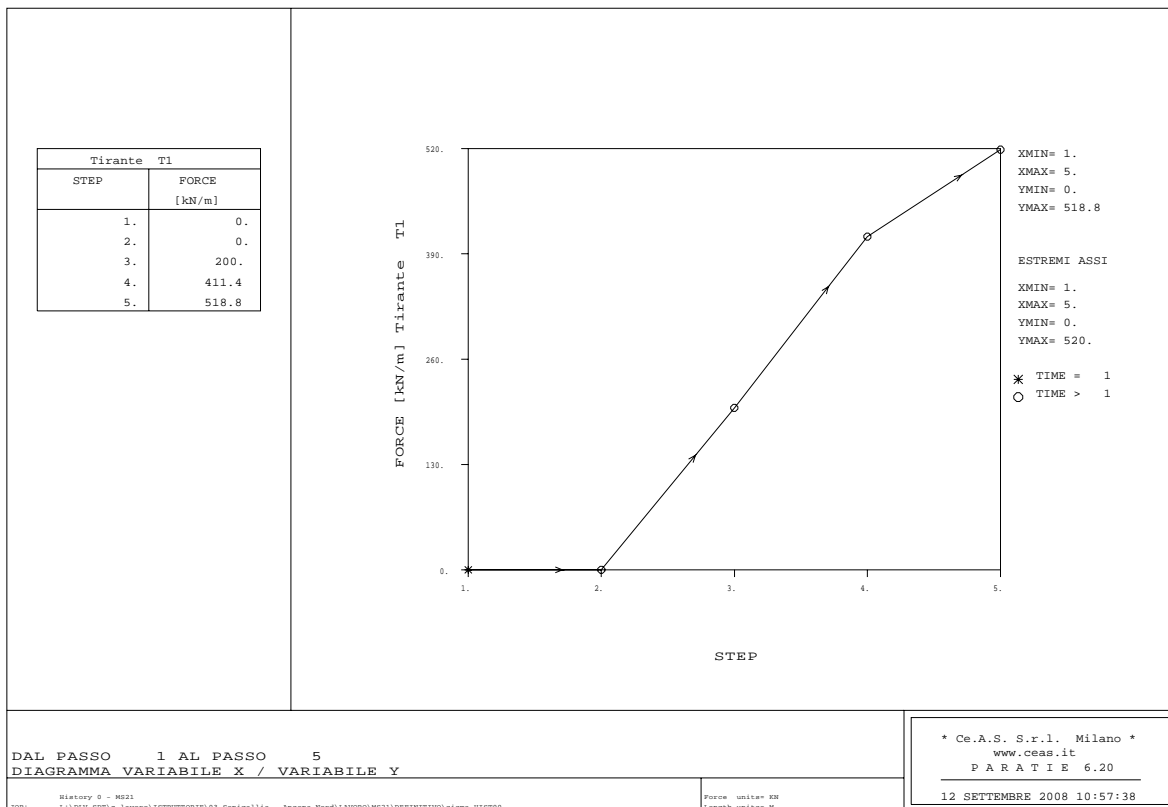
Figura 6.13 - Programma PARATIE – Tiro nel tirante – Caso sismico
