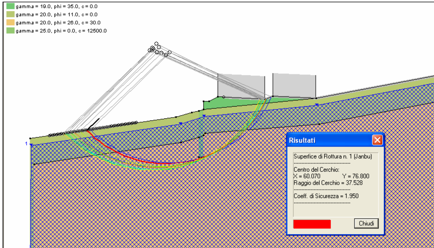
Figura 7.1- Analisi di stabilità globale nel caso statico ed individuazione della superficie di scorrimento avente Fs minimo
