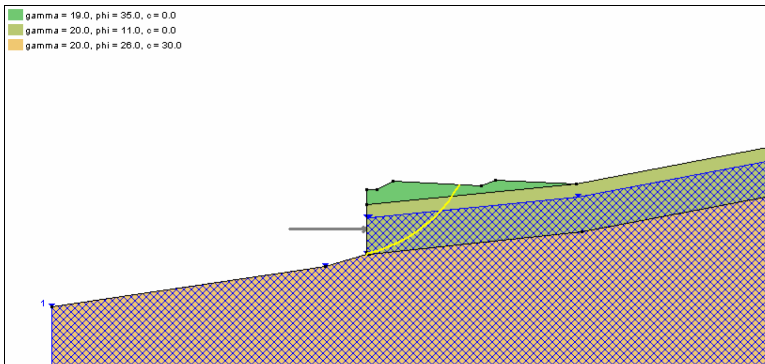
Figura 6.4- Analisi limite per la valutazione dell'azione che stabilizza il cuneo di monte in presenza del rilevato in progetto
