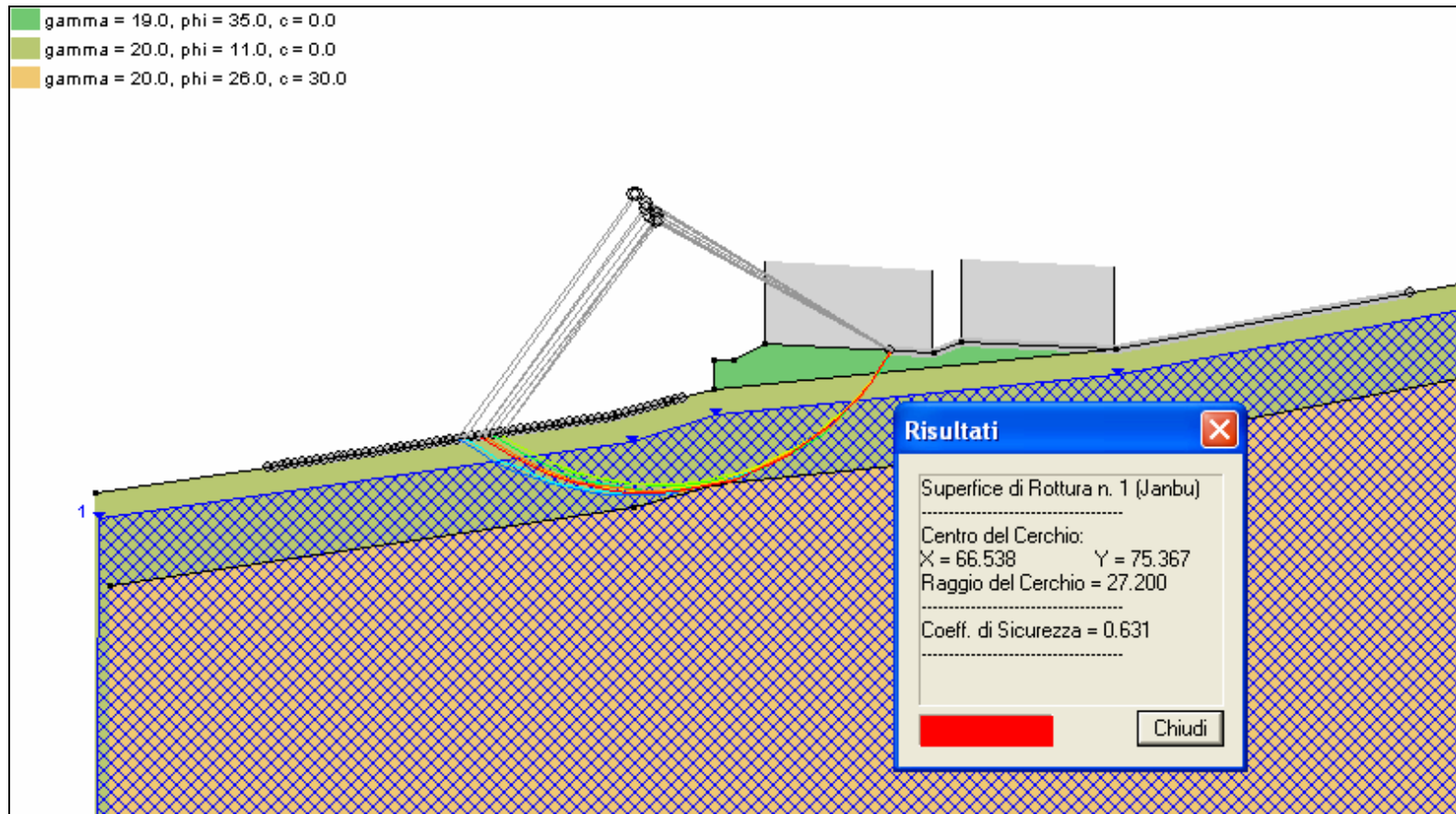
Figura 6.2- Analisi limite in condizione finale di progetto per la definizione della superficie di rottura critica
