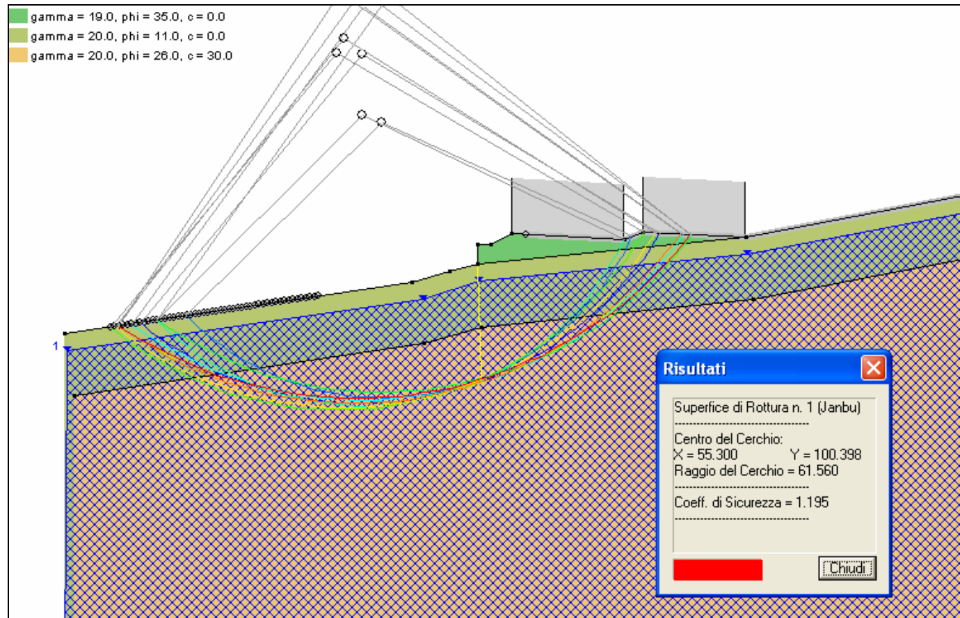
Figura 7.2- Analisi di stabilità globale nel caso sismico ed individuazione della superficie di scorrimento avente F_s minimo
