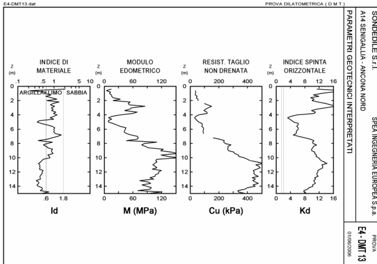
Figura 3.2 – Interpretazione dei parametri geotecnici dalle letture del dilatometro E4-DMT13
