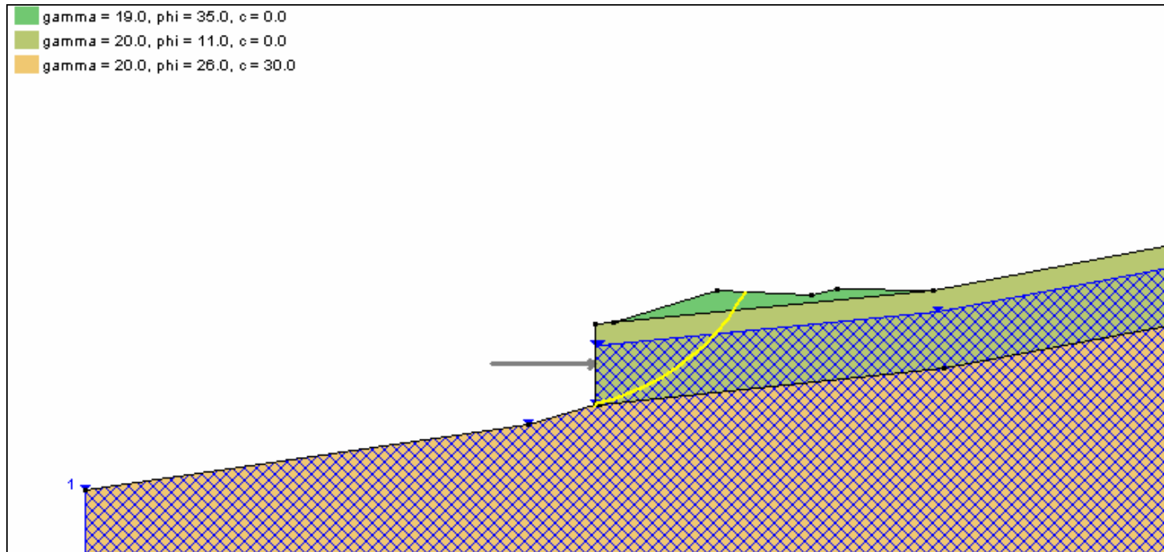
Figura 6.3- Analisi limite per la valutazione dell'azione che stabilizza il cuneo di monte con F_s=1,0 , nelle condizioni attuali (precedenti l'allargamento autostradale)
