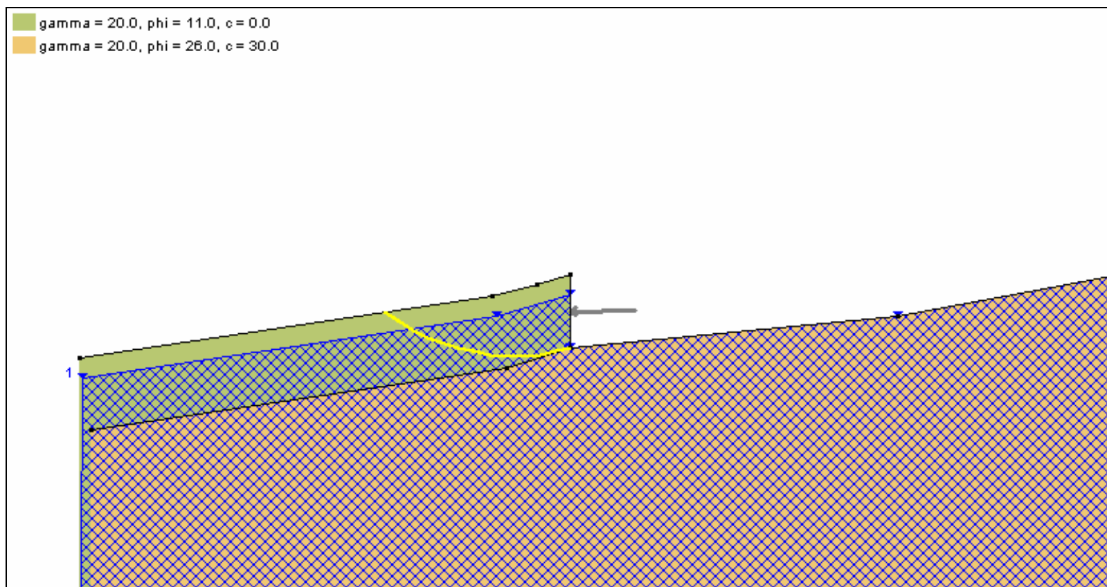
Figura 6.5- Analisi limite per la valutazione dell'azione che instabilizza il cuneo di valle
