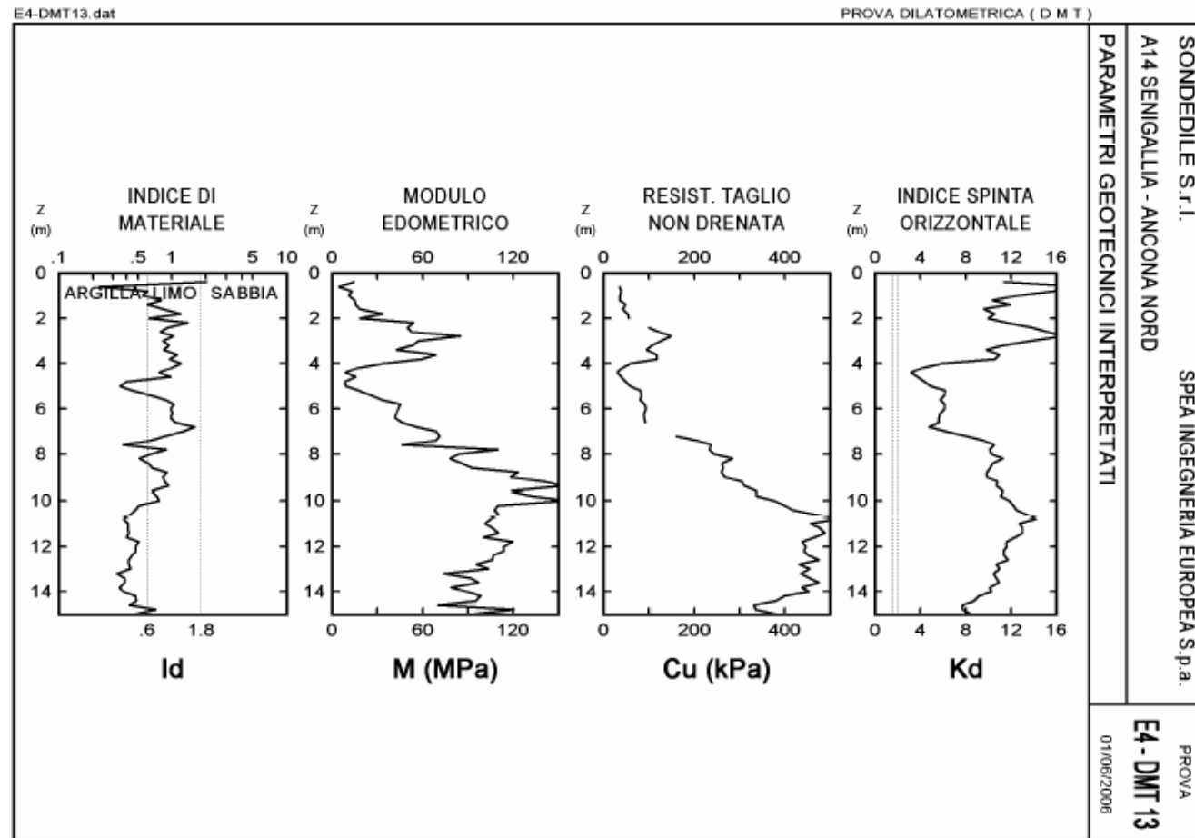
Figura 3.1 – Interpretazione dei parametri geotecnici dalle letture del dilatometro E4-DMT13
