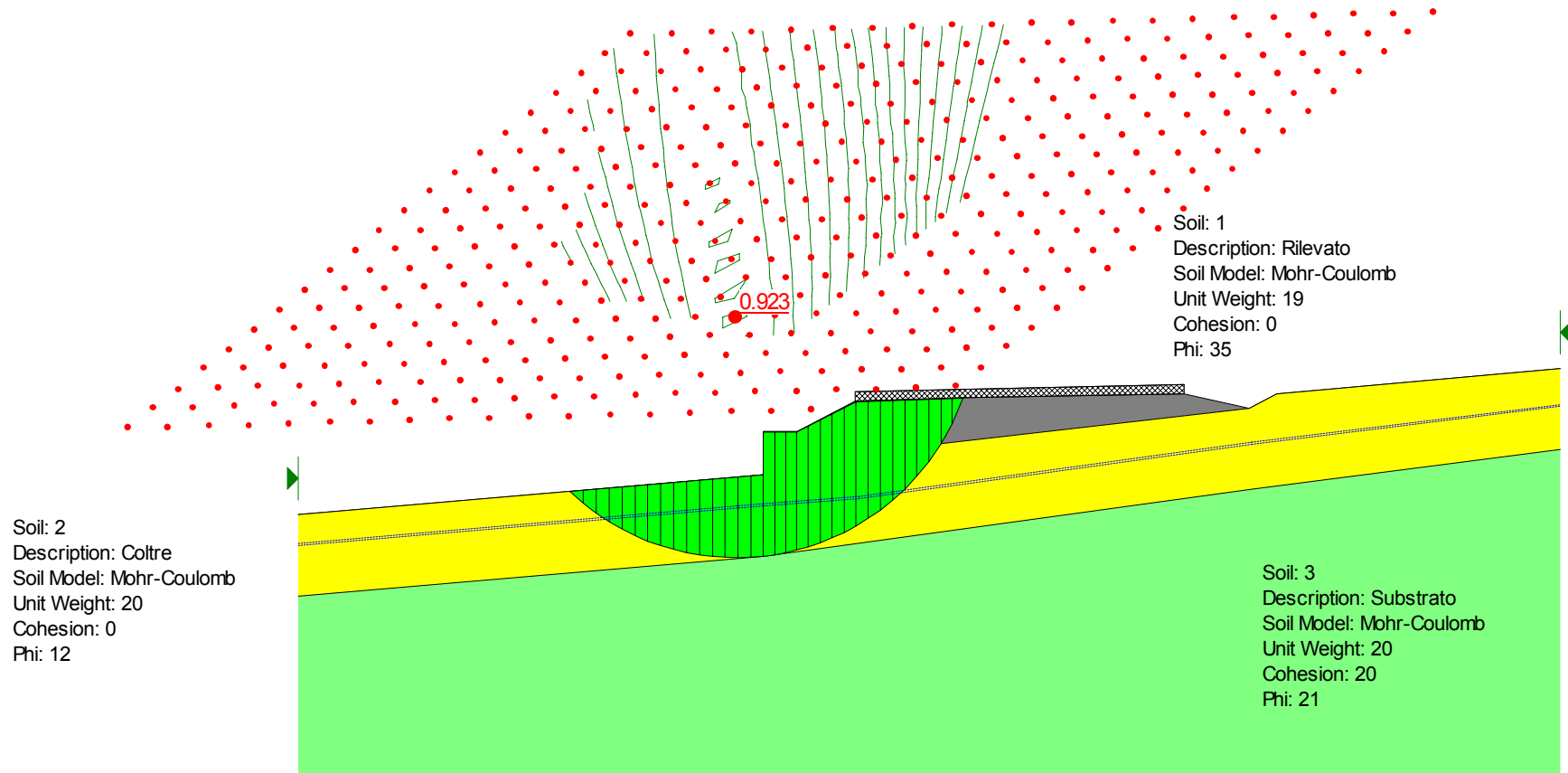
Figura 6.5- Analisi limite nelle condizioni finali per la definizione della superficie di rottura critica
