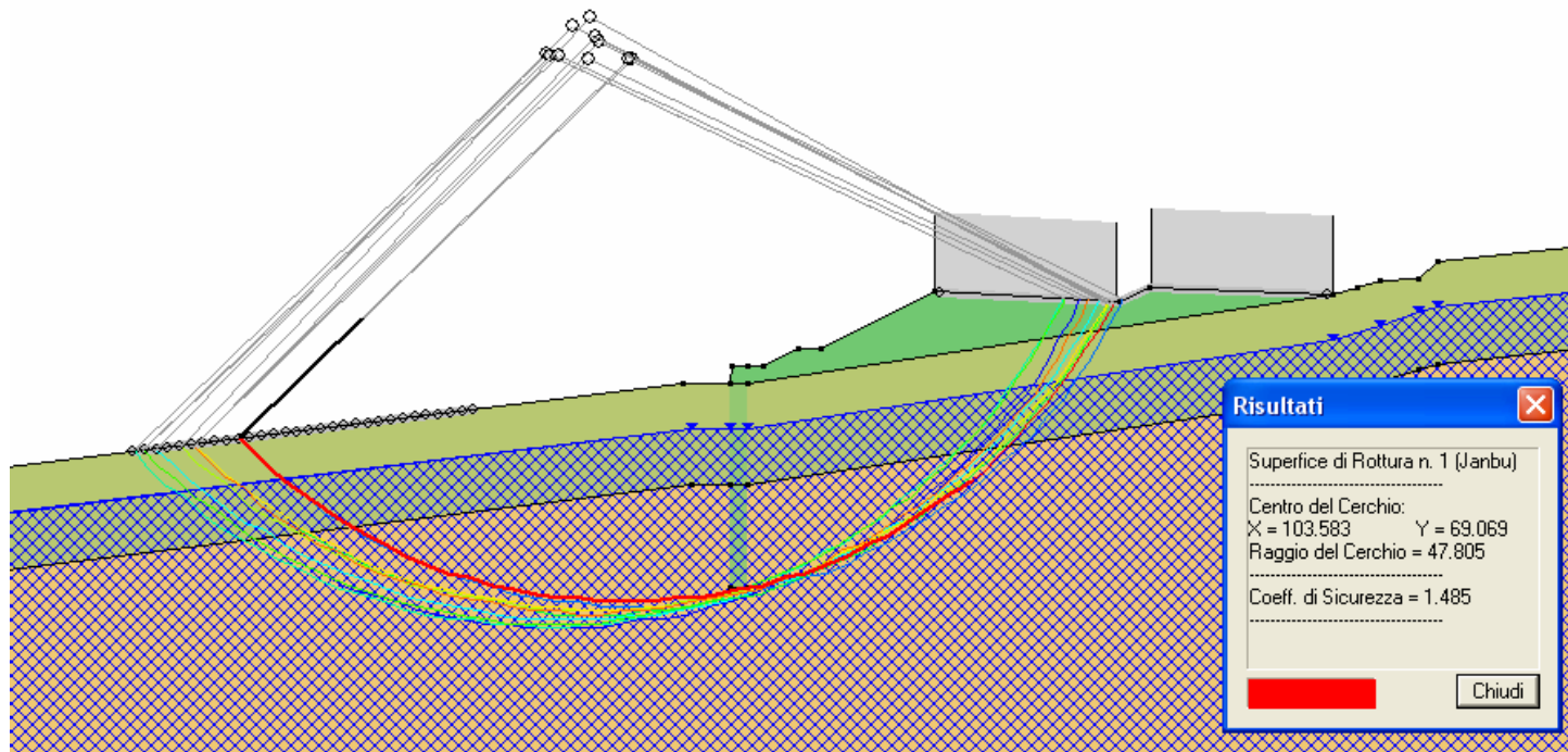
Figura 7.1- Analisi di stabilità globale nel caso statico ed individuazione della superficie di scorrimento avente Fs minimo
