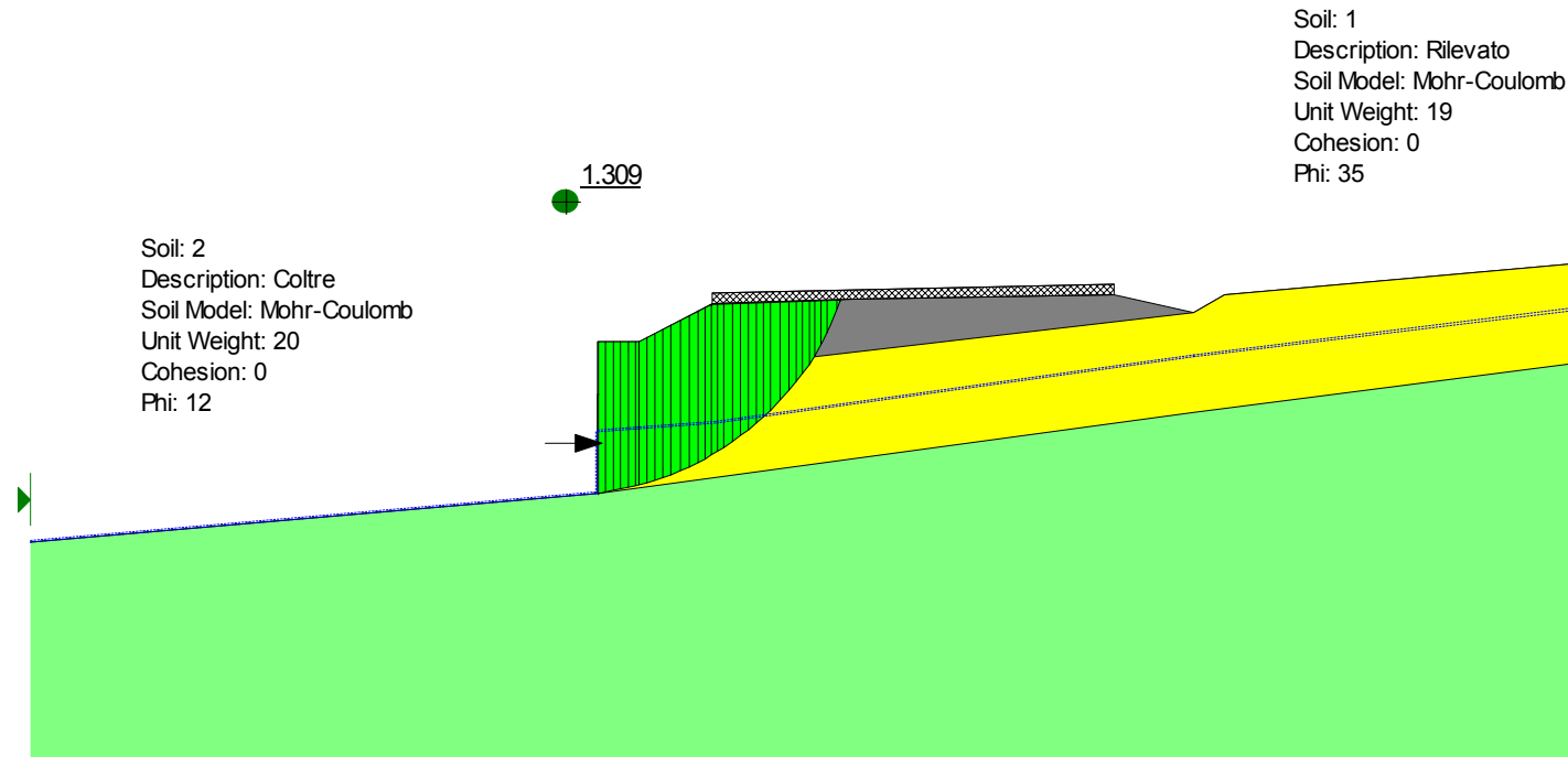
Figura 6.8- Analisi limite per la valutazione dell'azione che stabilizza il cuneo di monte con FS=1.3 nelle condizioni finali
