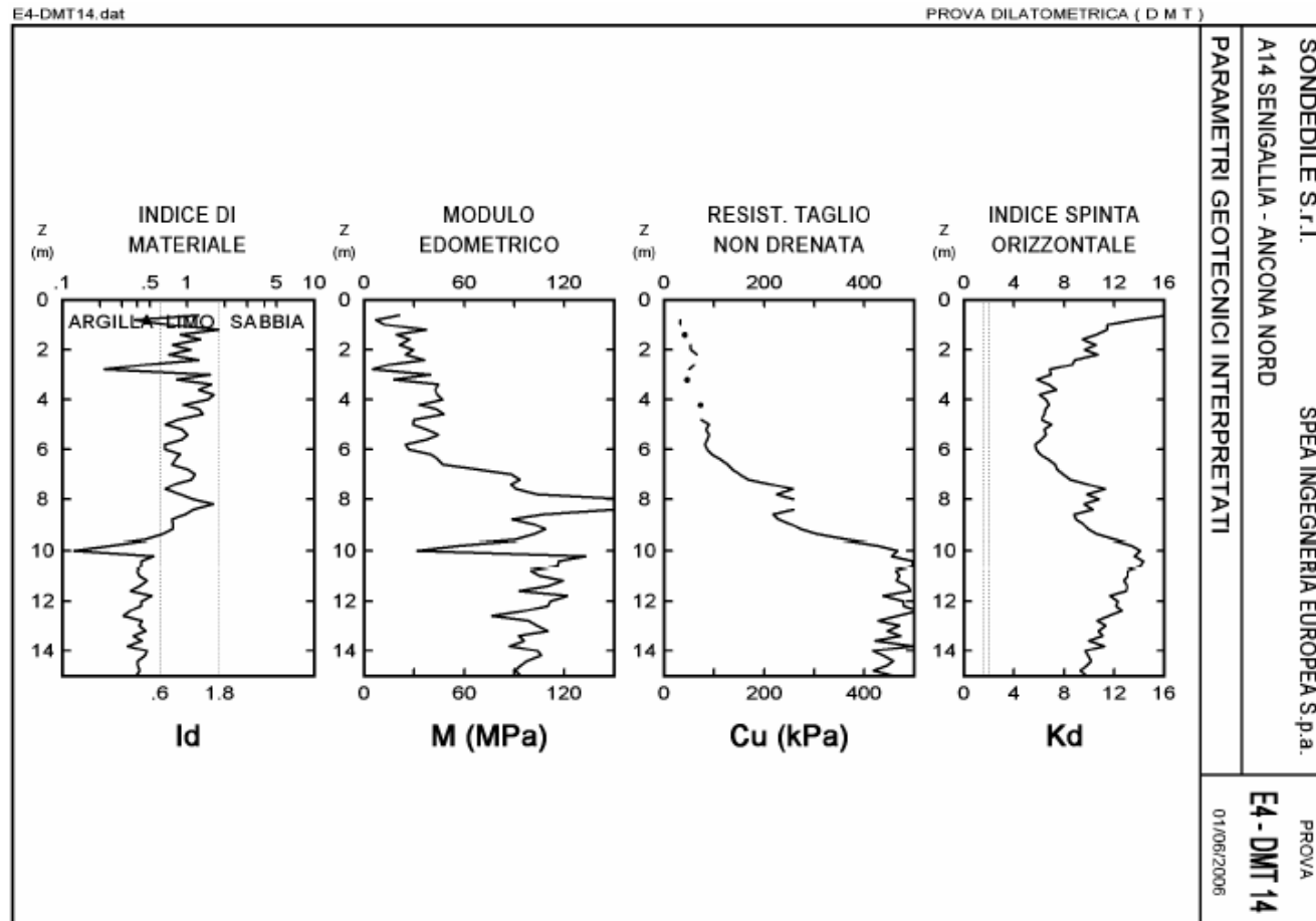
Figura 3.2 – Interpretazione dei parametri geotecnici dalle letture del dilatometro E4-DMT14
