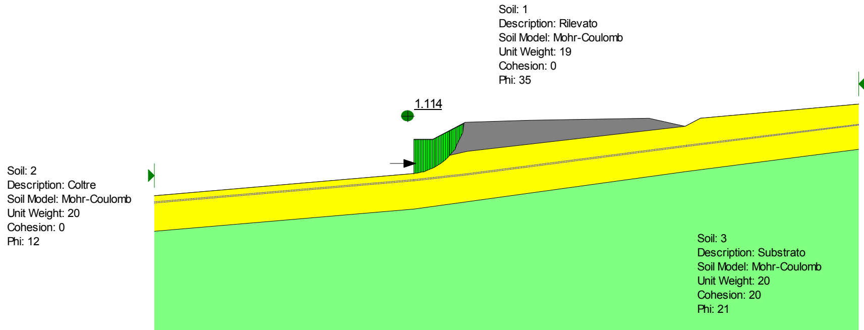
Figura 6.10 - Analisi limite per la valutazione dell'azione sismica con FS=1.1 nelle condizioni finali
