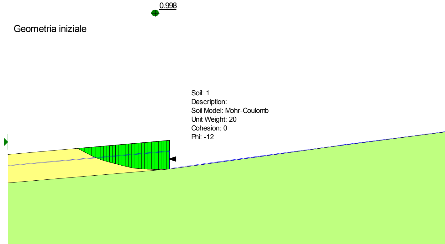
Figura 6.4- Analisi limite per la valutazione dell'azione che instabilizza il cuneo di valle con FS = 1.0 nelle condizioni iniziali
