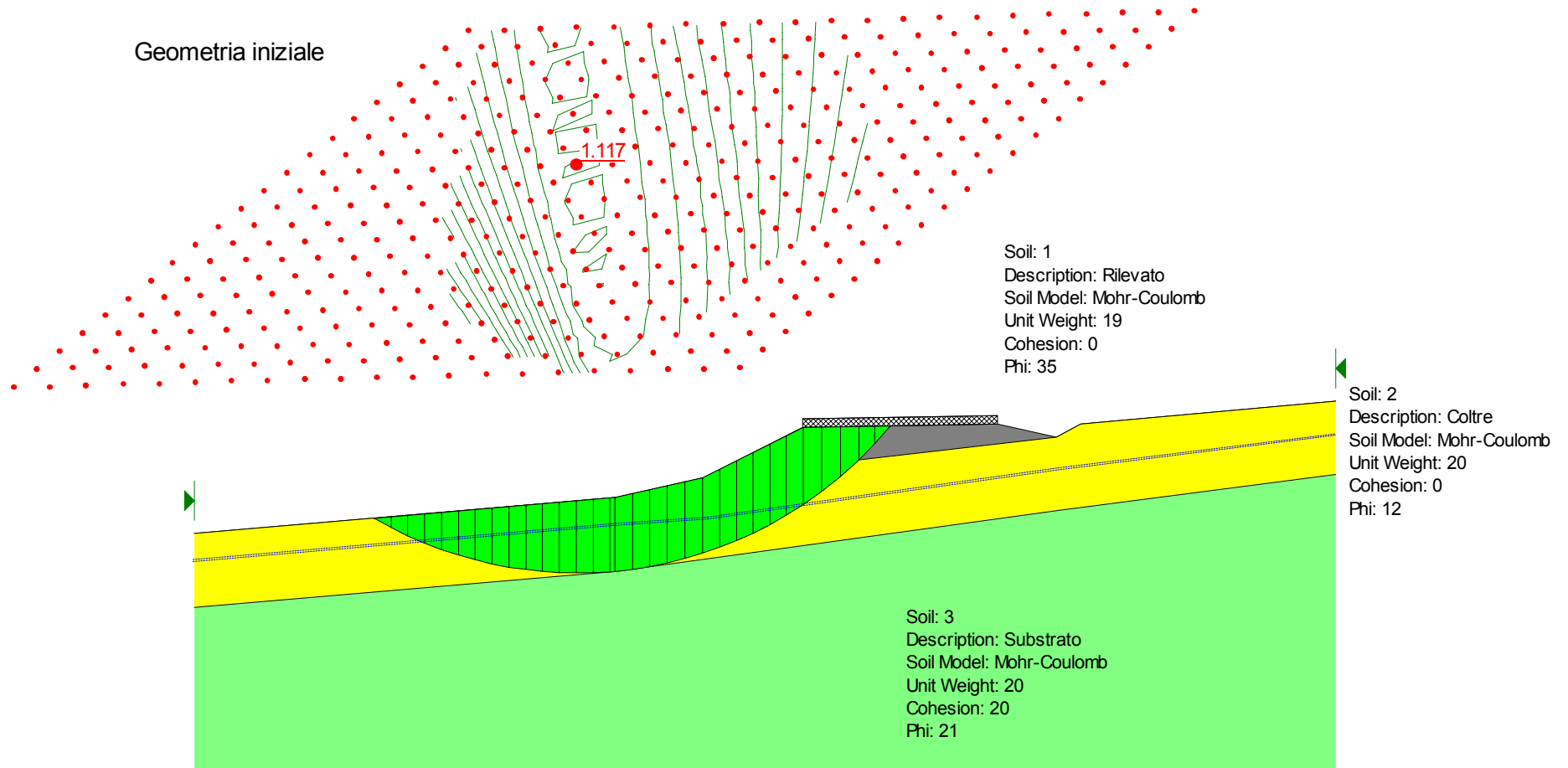
Figura 6.2- Analisi limite nelle condizioni iniziali per la definizione della superficie di rottura critica
