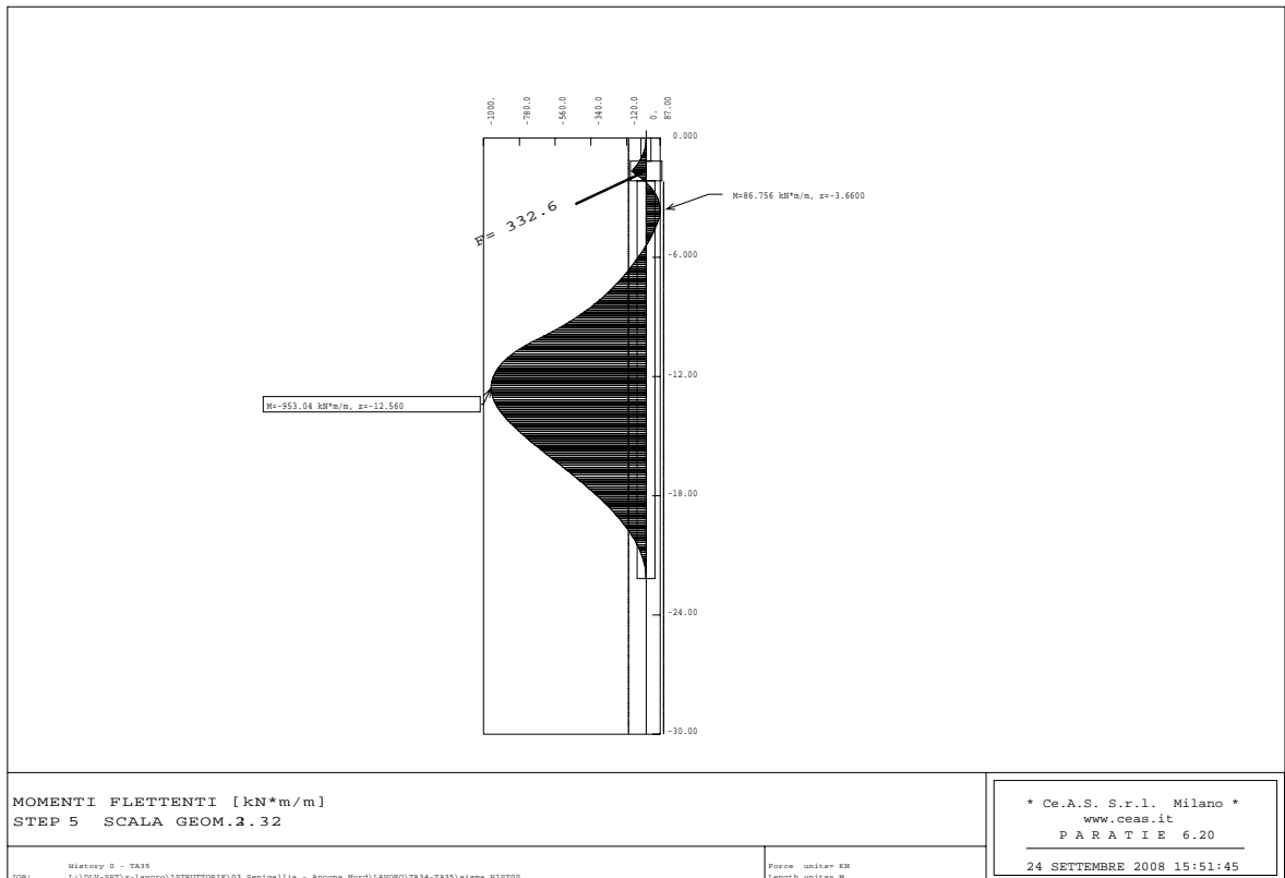
Figura 6.21 - Programma PARATIE – Fase SLU Sisma – Momento flettente
