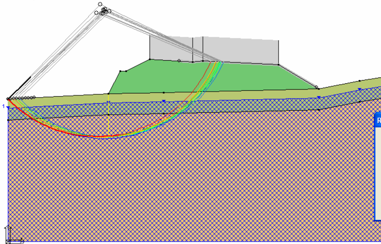
Figura 7.1, nella quale si rappresenta la superficie avente coefficiente di sicurezza minimo pari a 2,103. La verifica risulta dunque soddisfatta.
