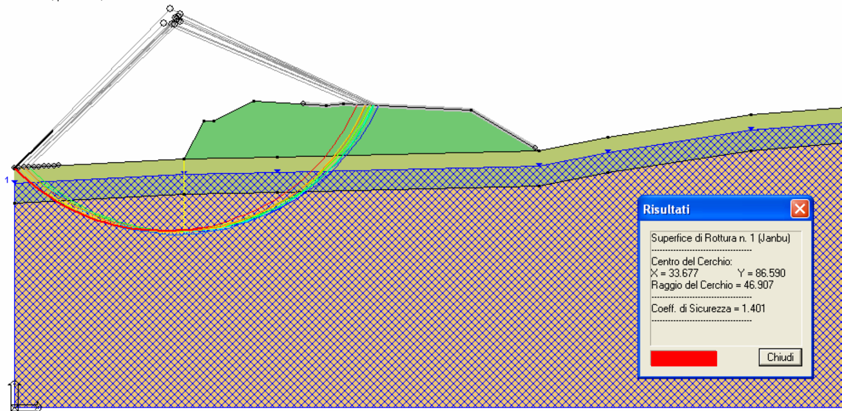
Figura 7.2- Analisi di stabilità globale nel ca sismico ed individuazione della superficie di scorrimento avente F_s minimo
