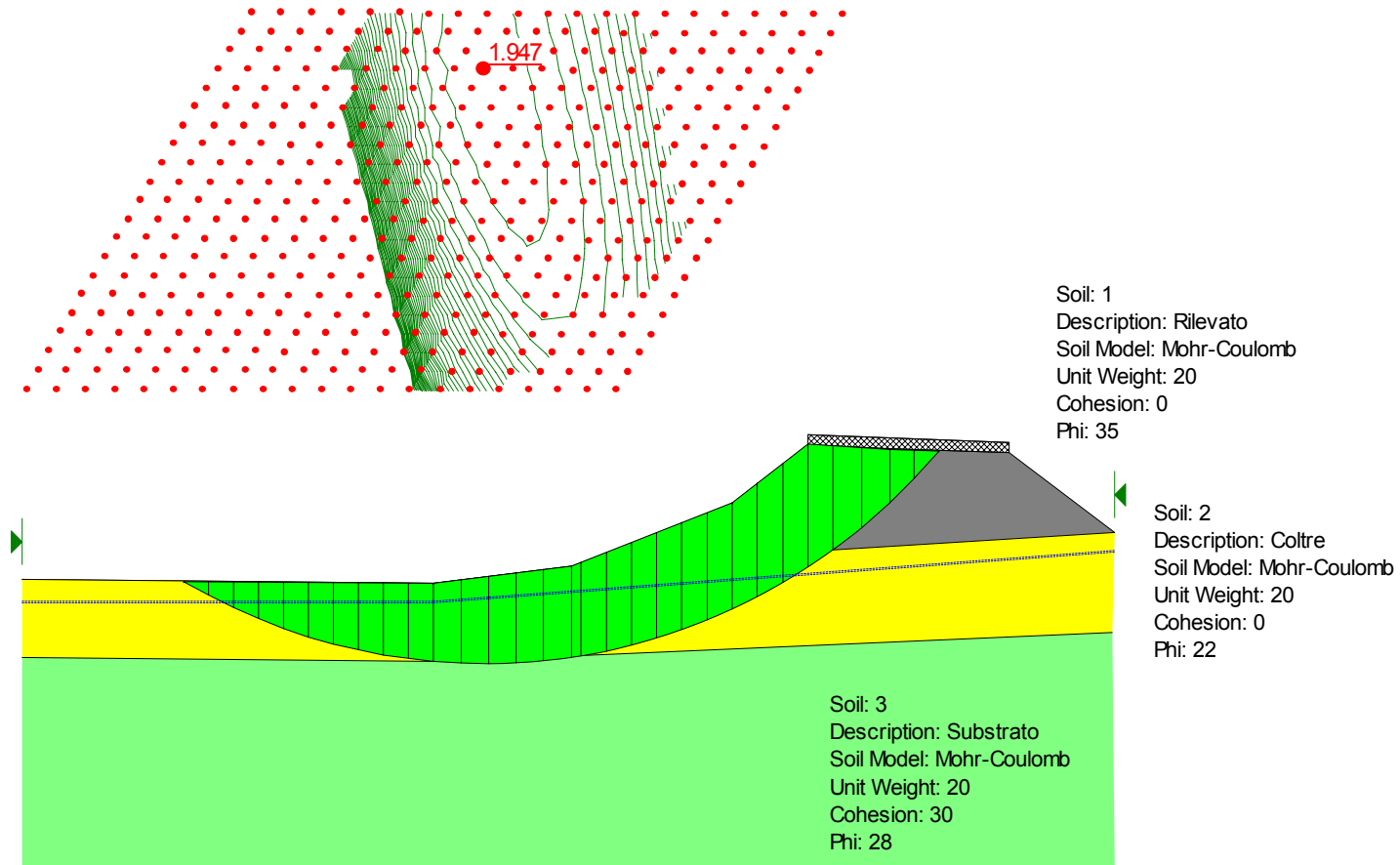
Figura 6.2- Analisi limite nelle condizioni iniziali per la definizione della superficie di rottura critica
