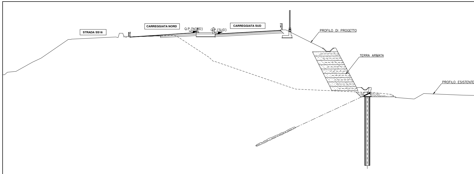
Figura 6.1- Sezione di calcolo
