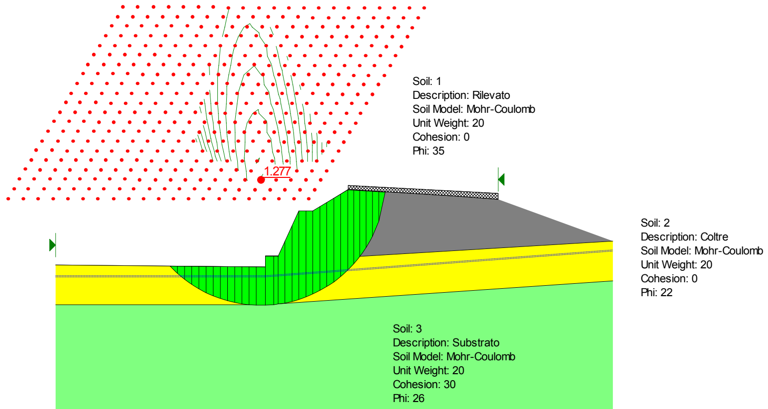
Figura 6.5- Analisi limite nelle condizioni finali per la definizione della superficie di rottura critica
