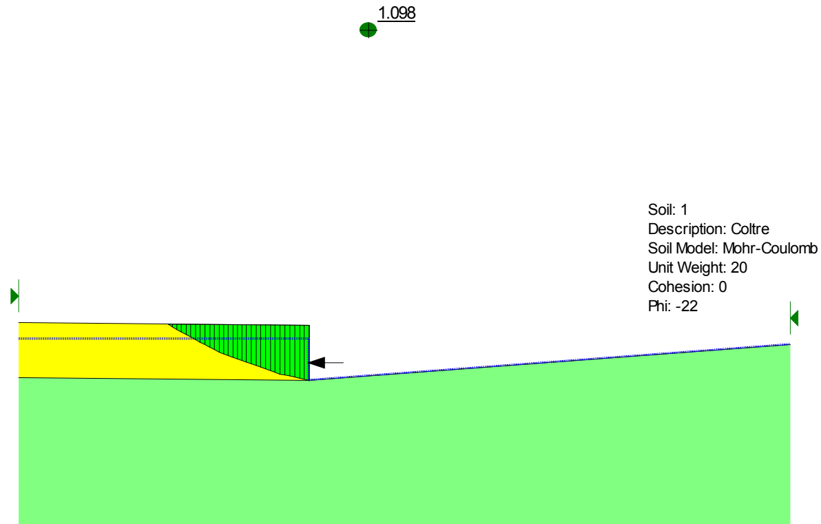
Figura 6.4- Analisi limite per la valutazione dell'azione che instabilizza il cuneo di valle con FS = 1.0 nelle condizioni iniziali
