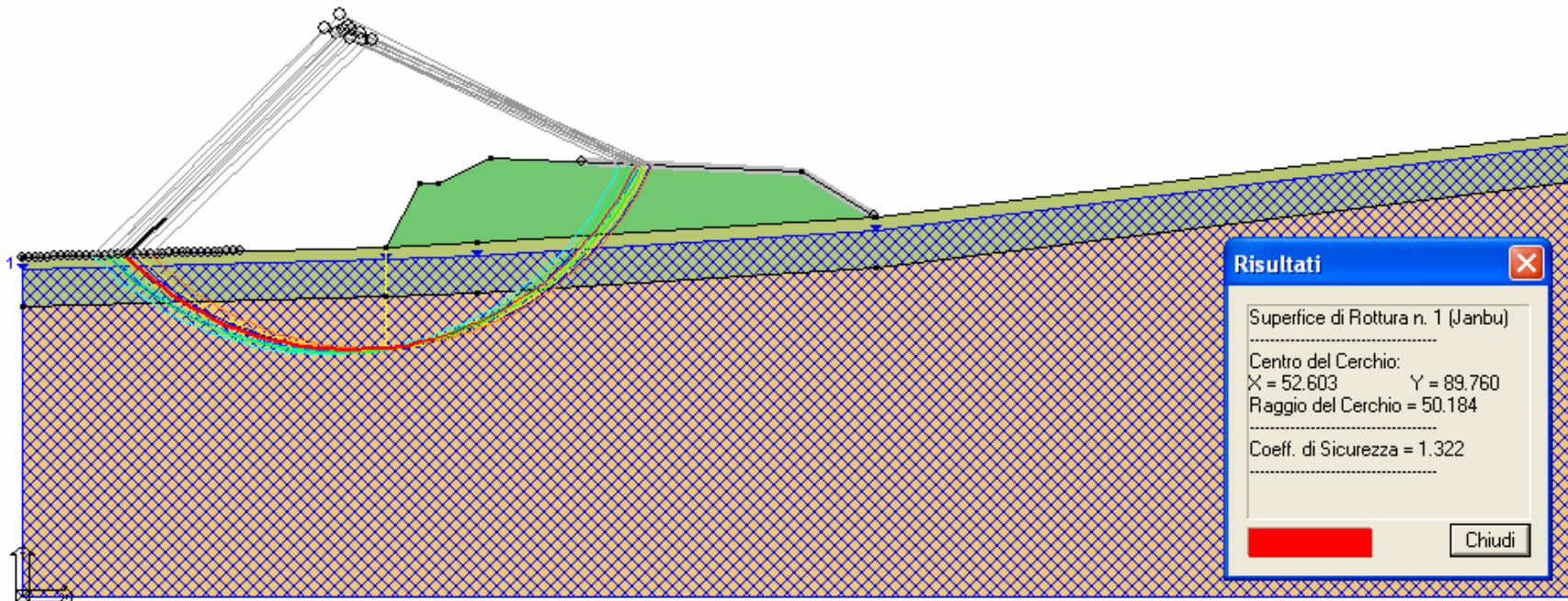
Figura 7.2- Analisi di stabilità globale nel ca sismico ed individuazione della superficie di scorrimento avente Fs minimo
