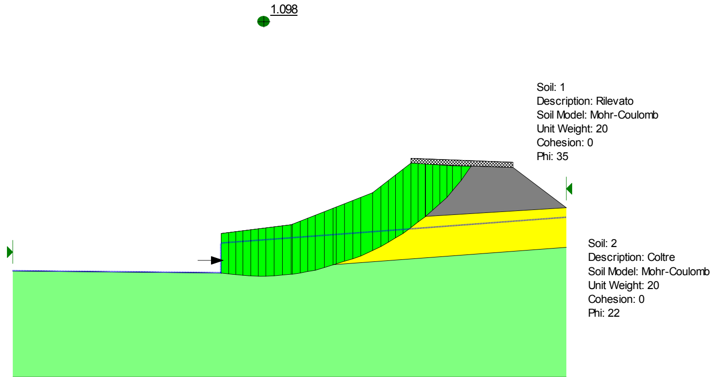
Figura 6.3- Analisi limite per la valutazione dell'azione che stabilizza il cuneo di monte con FS=1.0 nelle condizioni iniziali
