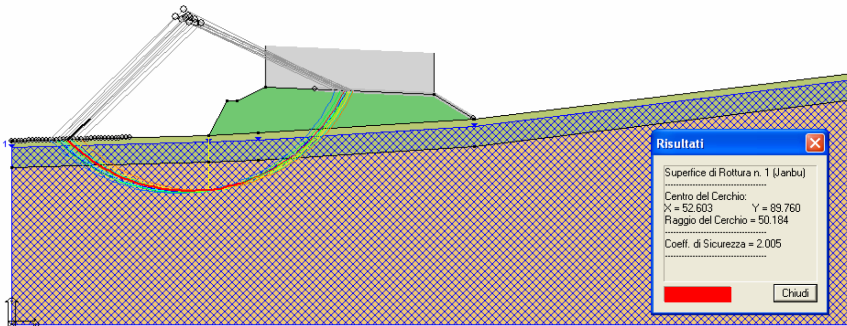
Figura 7.1- Analisi di stabilità globale nel caso statico ed individuazione della superficie di scorrimento avente Fs minimo
