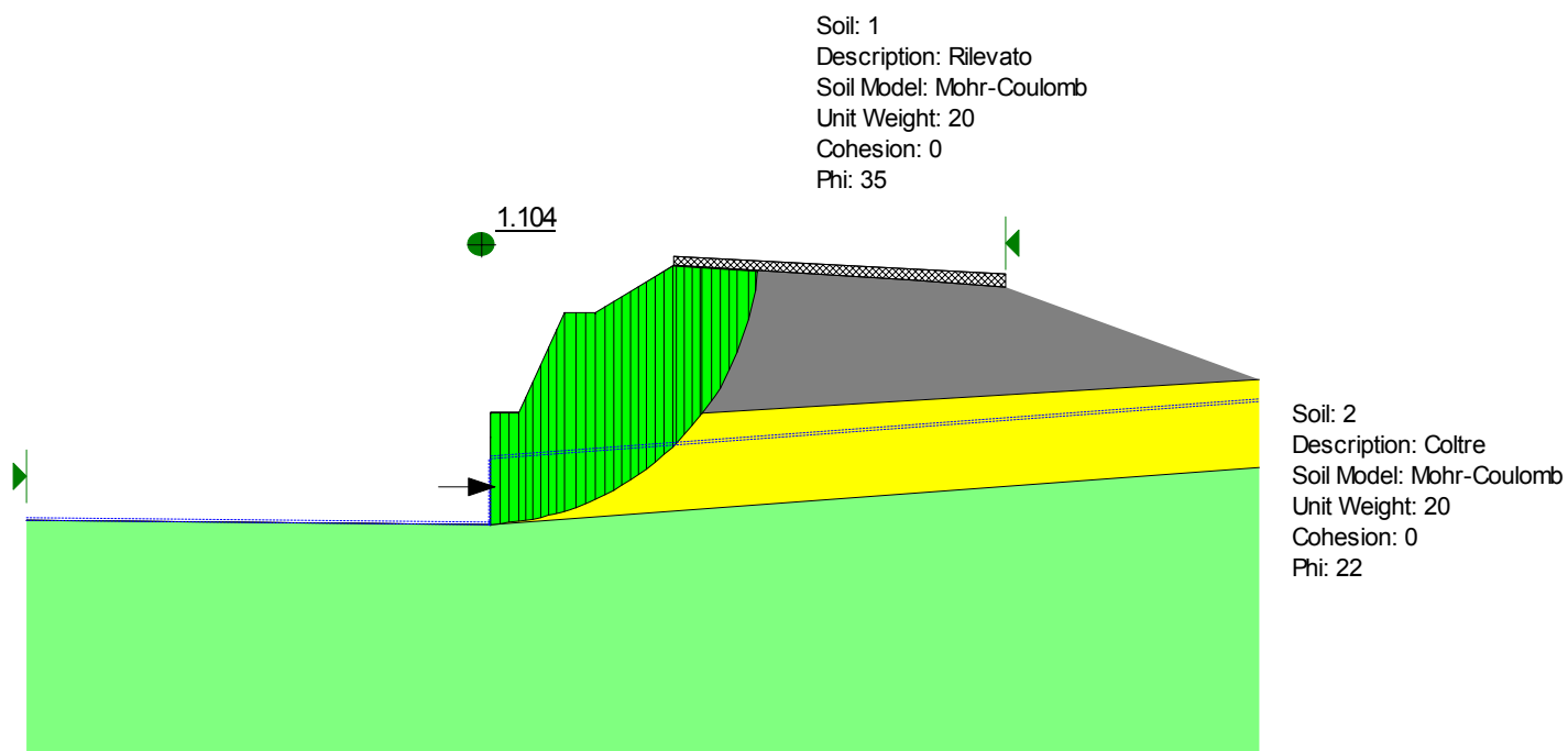
Figura 6.6- Analisi limite per la valutazione dell'azione che stabilizza il cuneo di monte con FS=1.1 nelle condizioni finali
