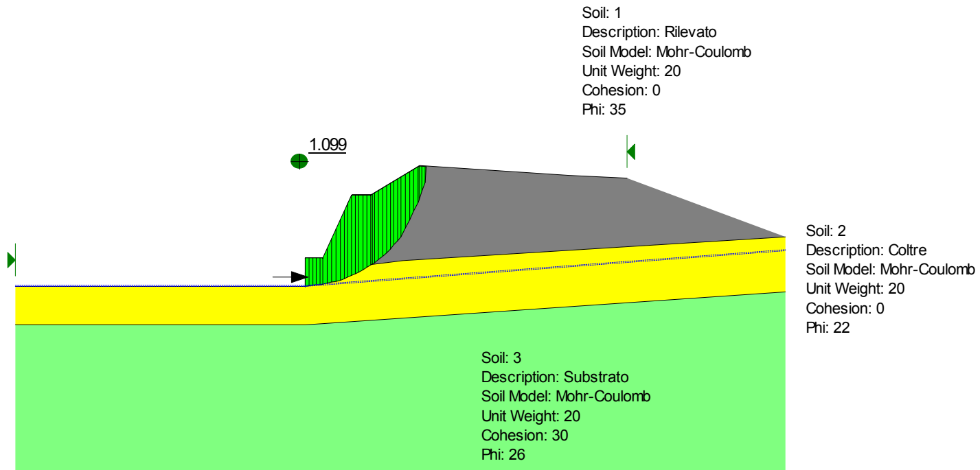
Figura 6.10 - Analisi limite per la valutazione dell'azione sismica con FS=1.1 nelle condizioni finali
