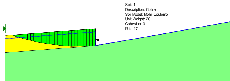
Figura 6.4- Analisi limite per la valutazione dell'azione che instabilizza il cuneo di valle con FS = 1.0 nelle condizioni iniziali
