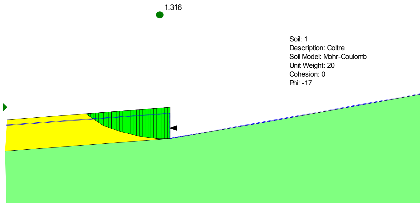
Figura 6.9- Analisi limite per la valutazione dell'azione che instabilizza il cuneo di valle con FS=1.3 nelle condizioni finali
