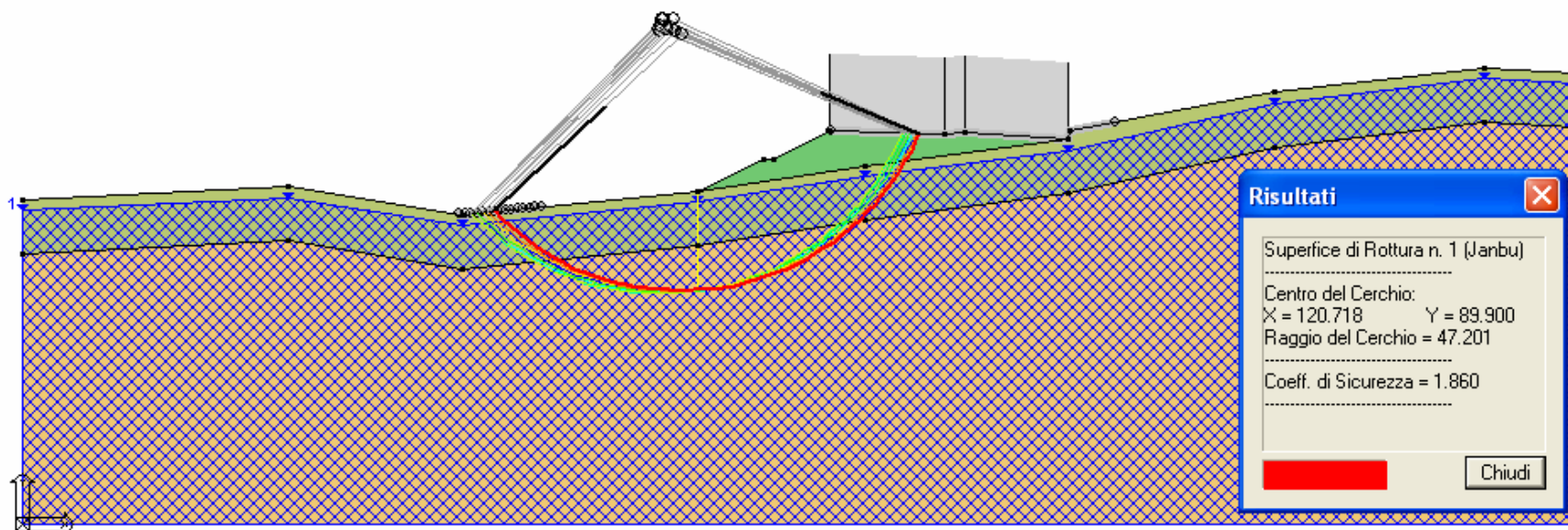
Figura 7.1- Analisi di stabilità globale nel caso statico ed individuazione della superficie di scorrimento avente Fs minimo
