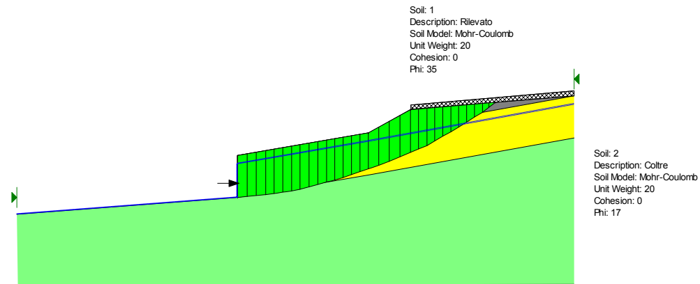
Figura 6.3- Analisi limite per la valutazione dell'azione che stabilizza il cuneo di monte con FS=1.0 nelle condizioni iniziali
