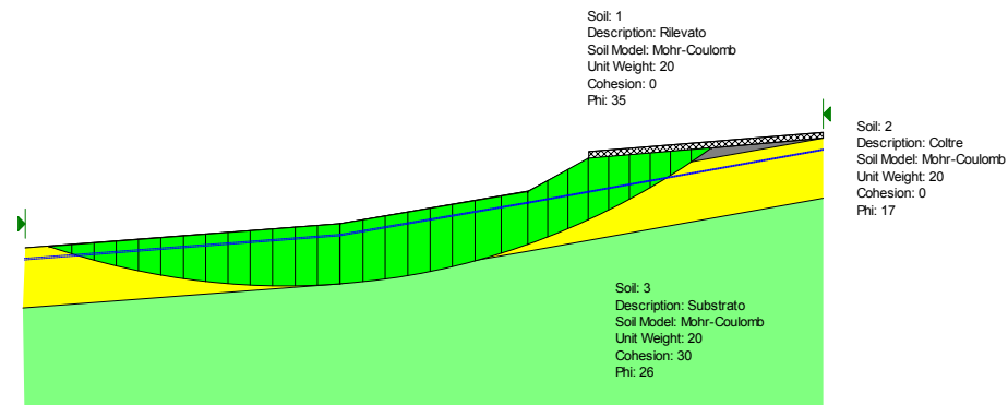
Figura 6.2- Analisi limite nelle condizioni iniziali per la definizione della superficie di rottura critica
