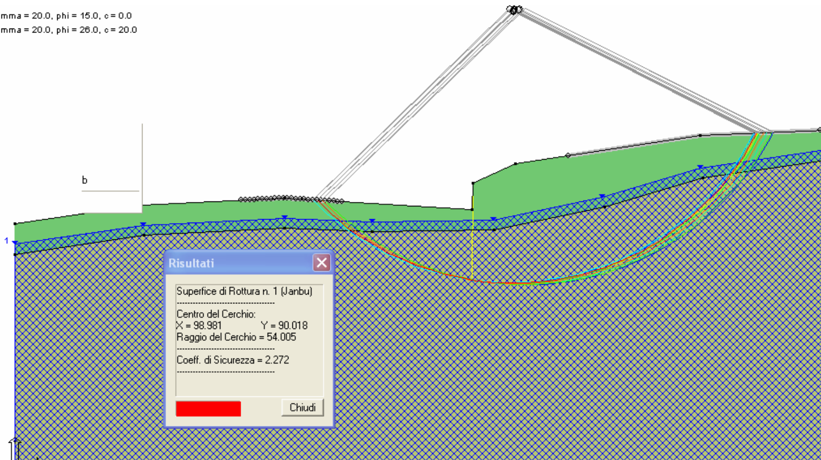
Figura 7.1- Analisi di stabilità globale nel caso statico ed individuazione della superficie di scorrimento avente F_s minimo
