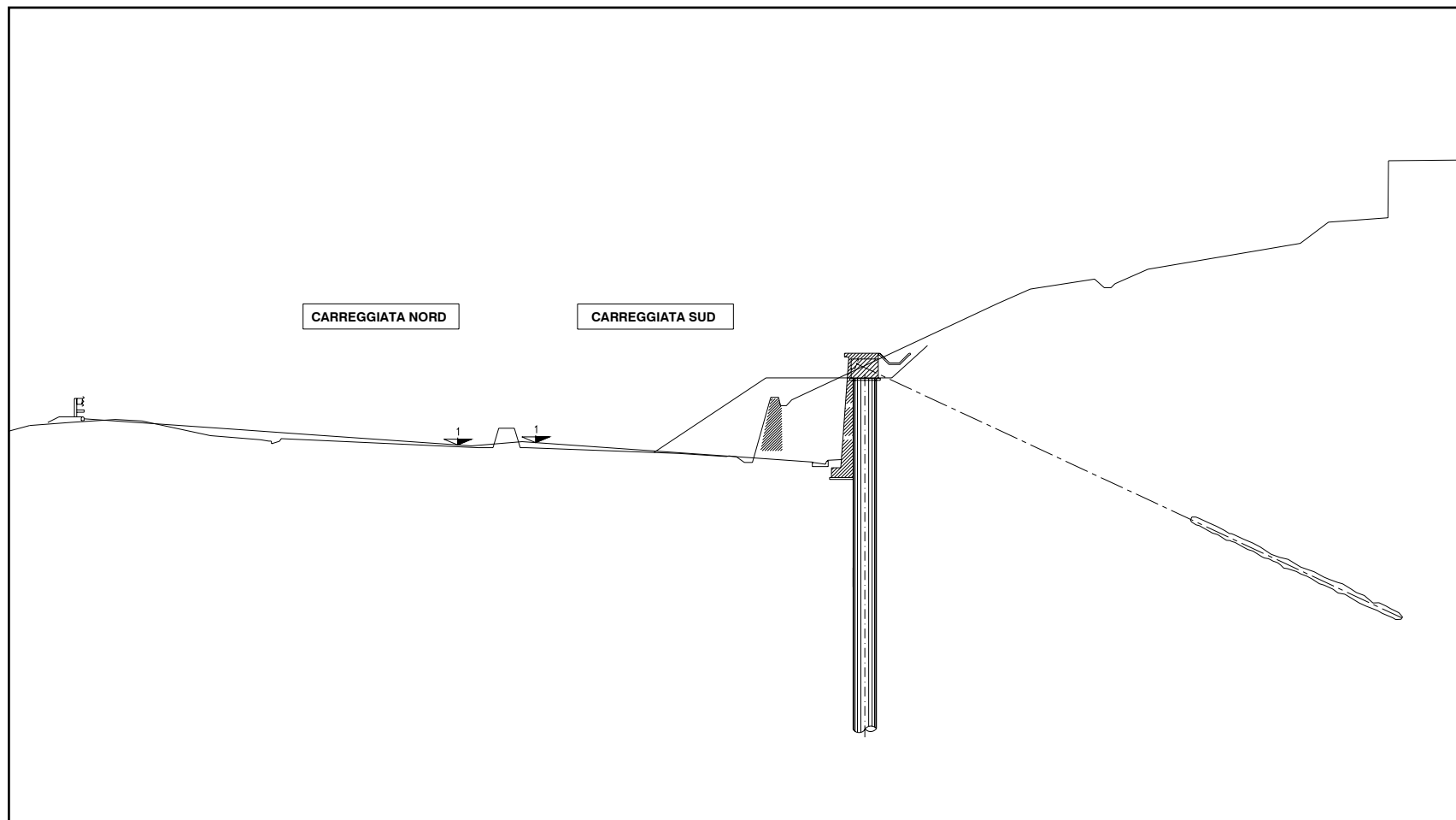
Figura 6.1- Sezione di calcolo
