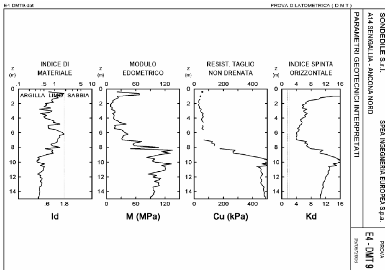
Figura 3.6 – Interpretazione dei parametri geotecnici dalle letture del dilatometro E4-DMT9
