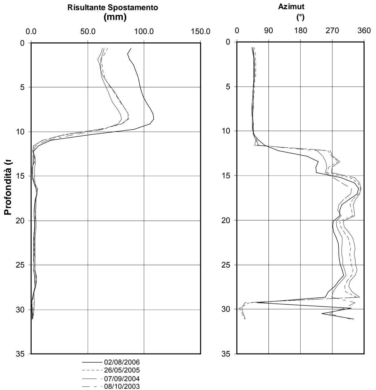
Figura 3.1 Grafici delle letture inclinometro I1
