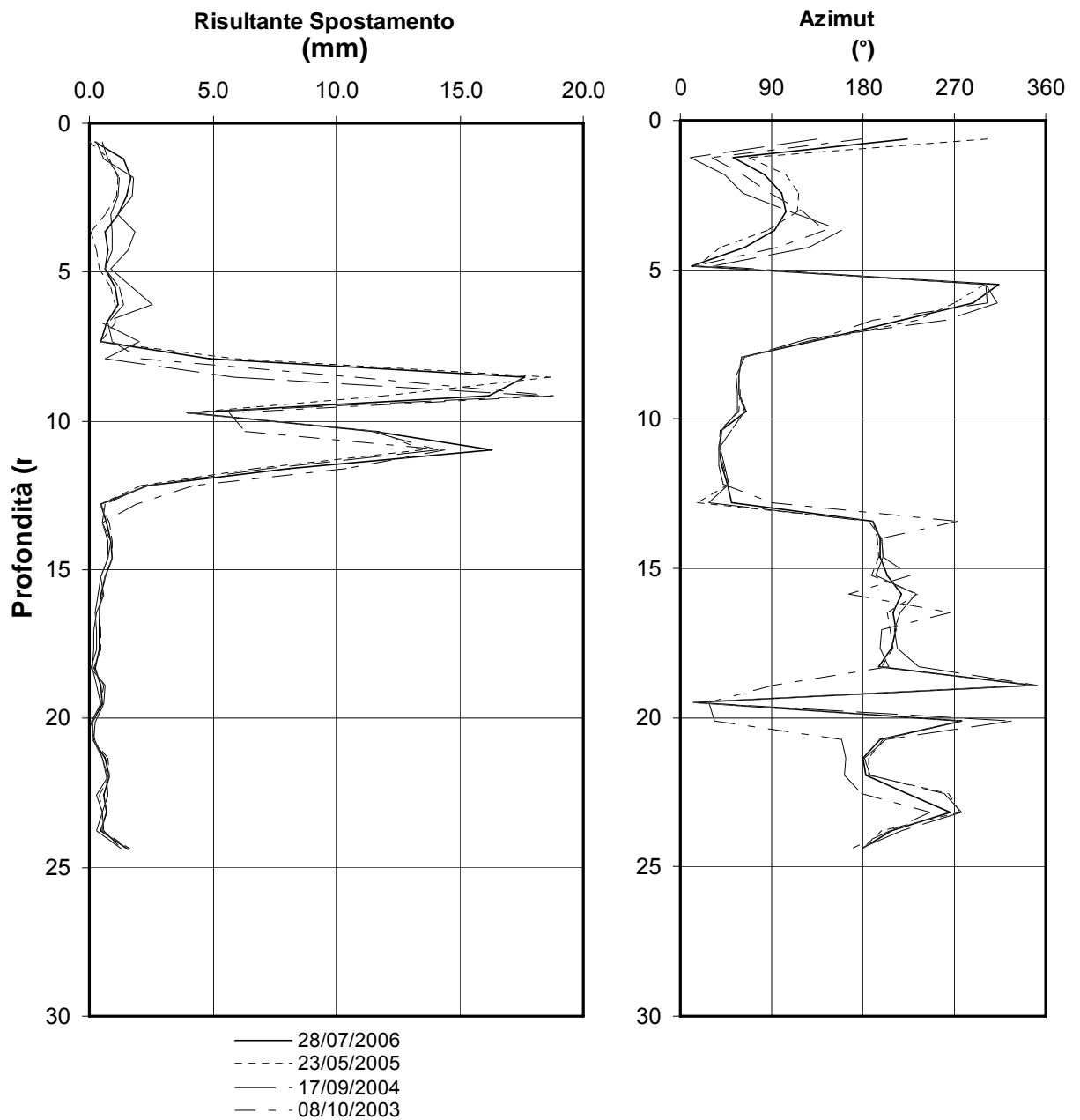
Figura 3.4 Grafici delle letture inclinometro I2
