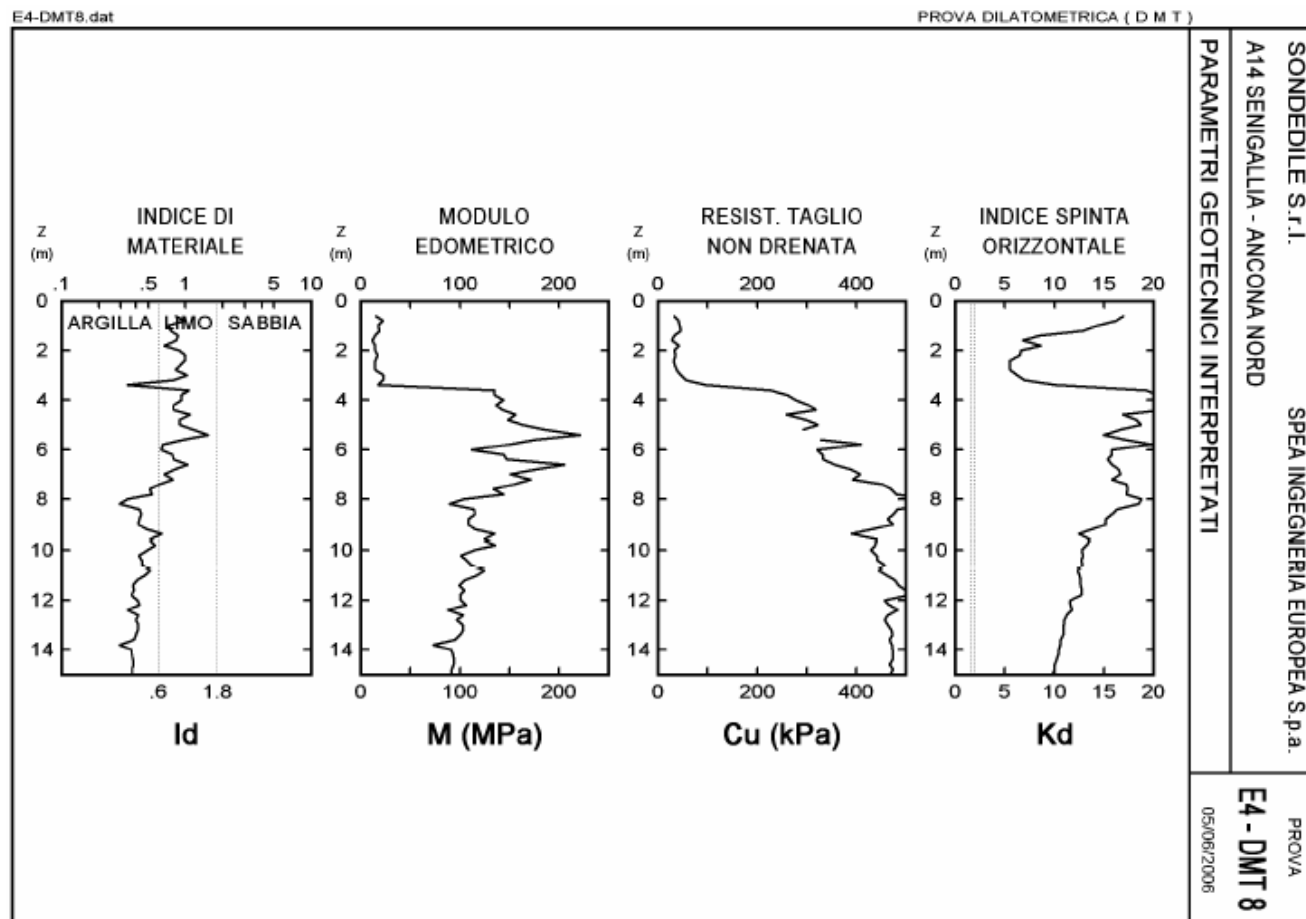
Figura 3.5 – Interpretazione dei parametri geotecnici dalle letture del dilatometro E4-DMT8
