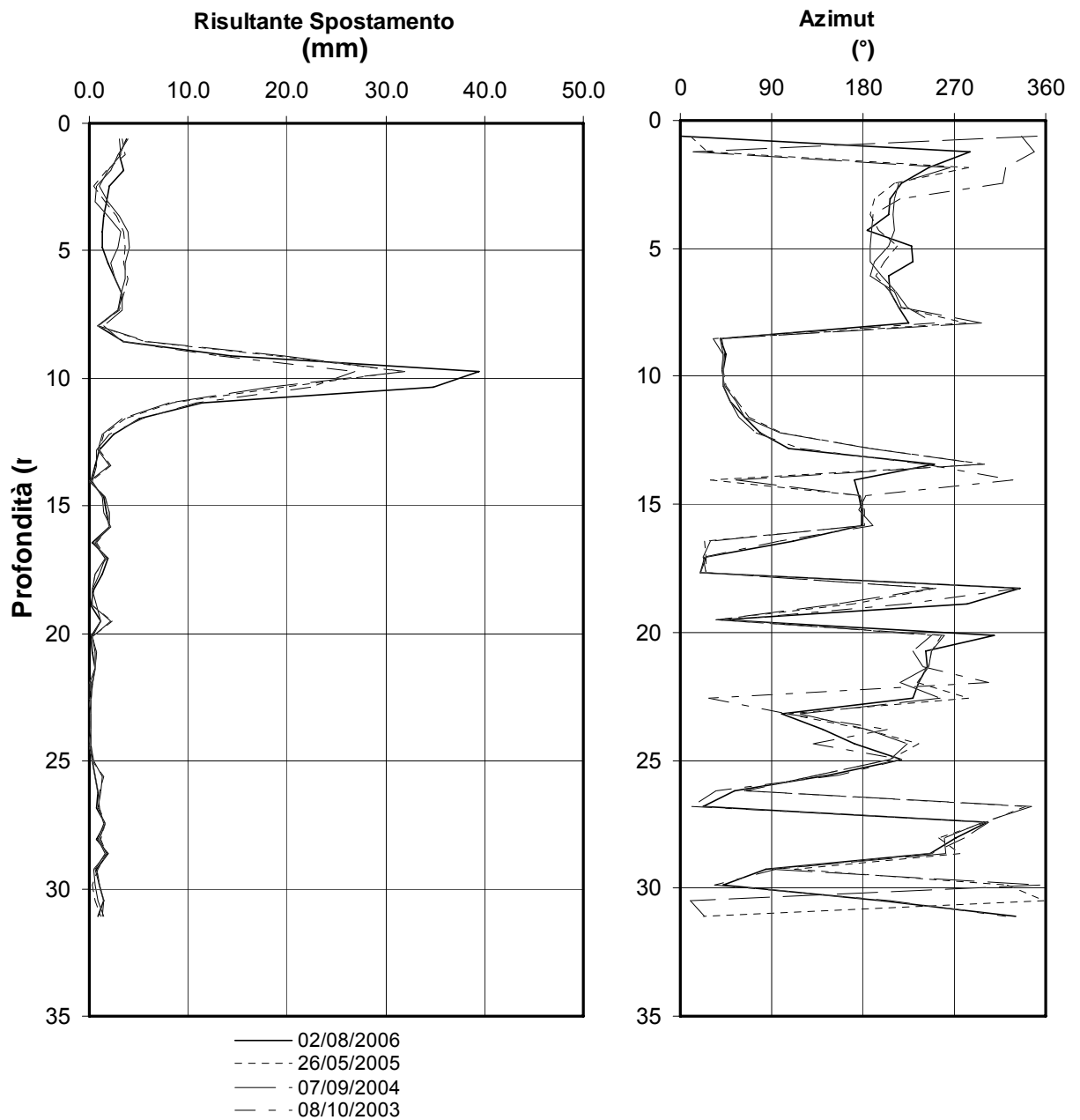
Figura 3.2 Grafici delle letture inclinometro I1
