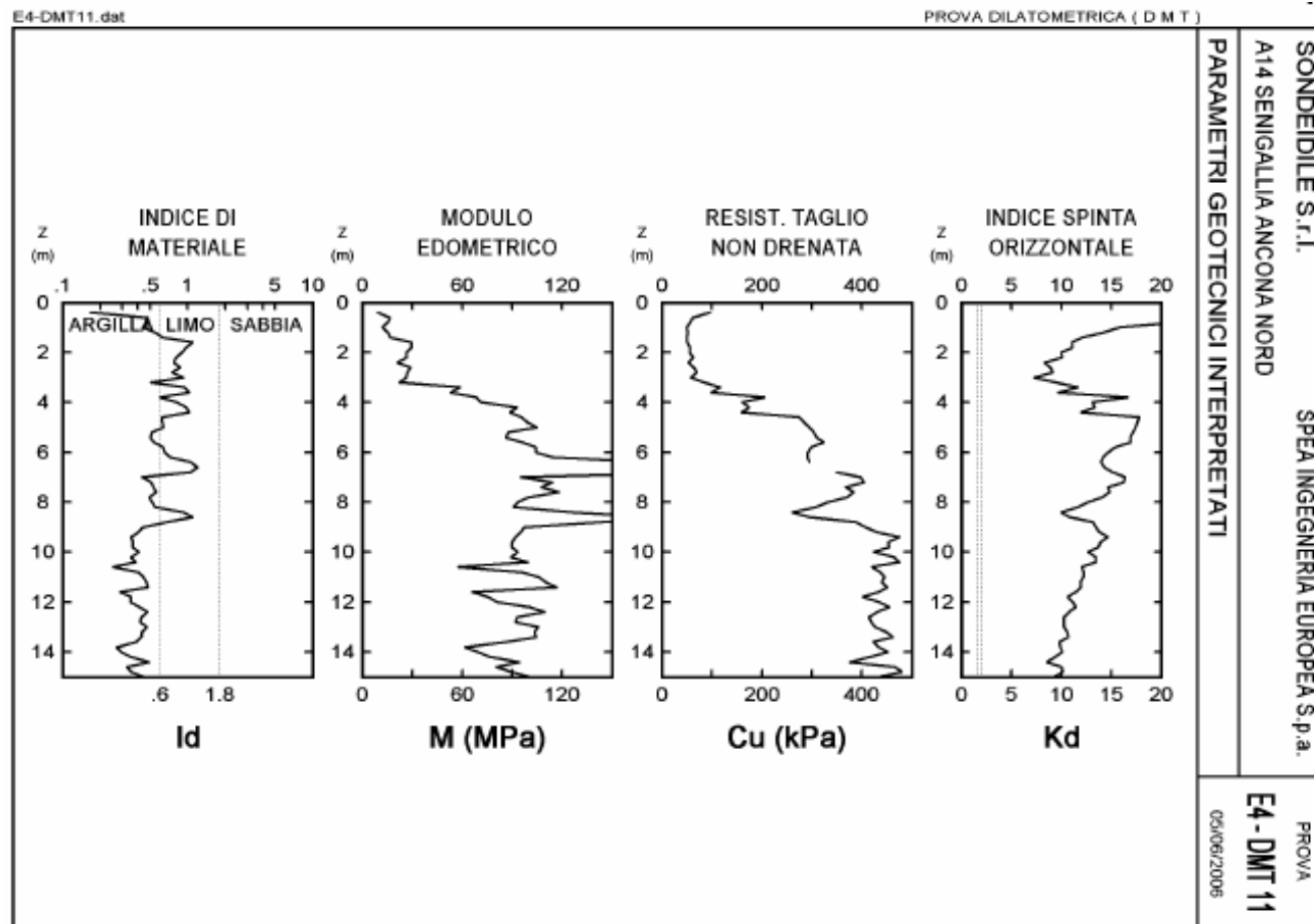
Figura 3.7 – Interpretazione dei parametri geotecnici dalle letture del dilatometro E4-DMT11
