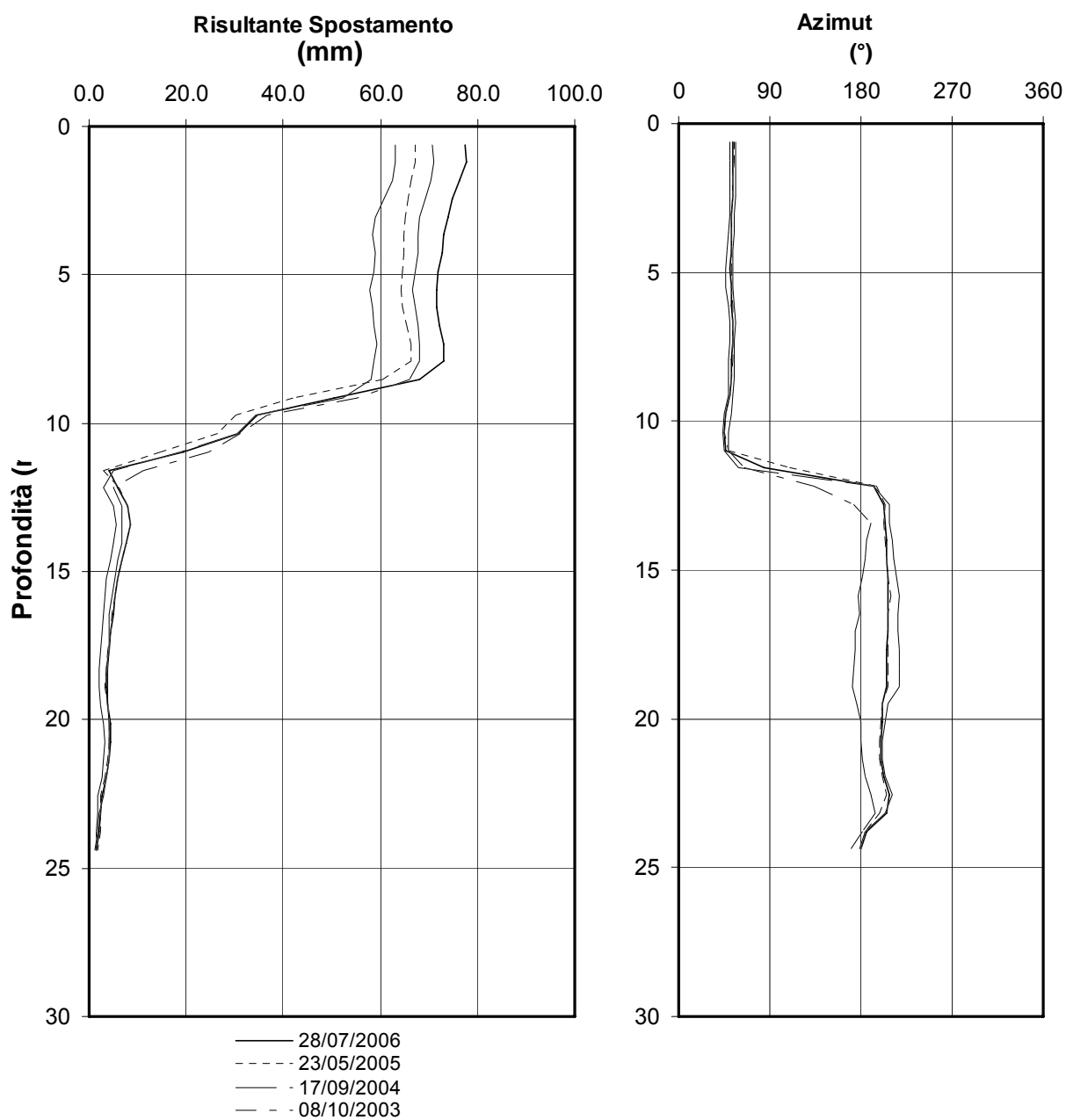
Figura 3.3 Grafici delle letture inclinometro I2
