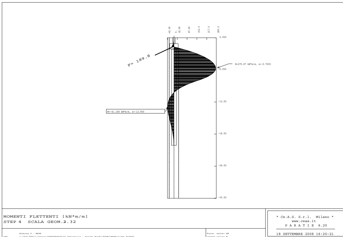
Figura 6.16 - Programma PARATIE – Fase di esercizio – Momento flettente
