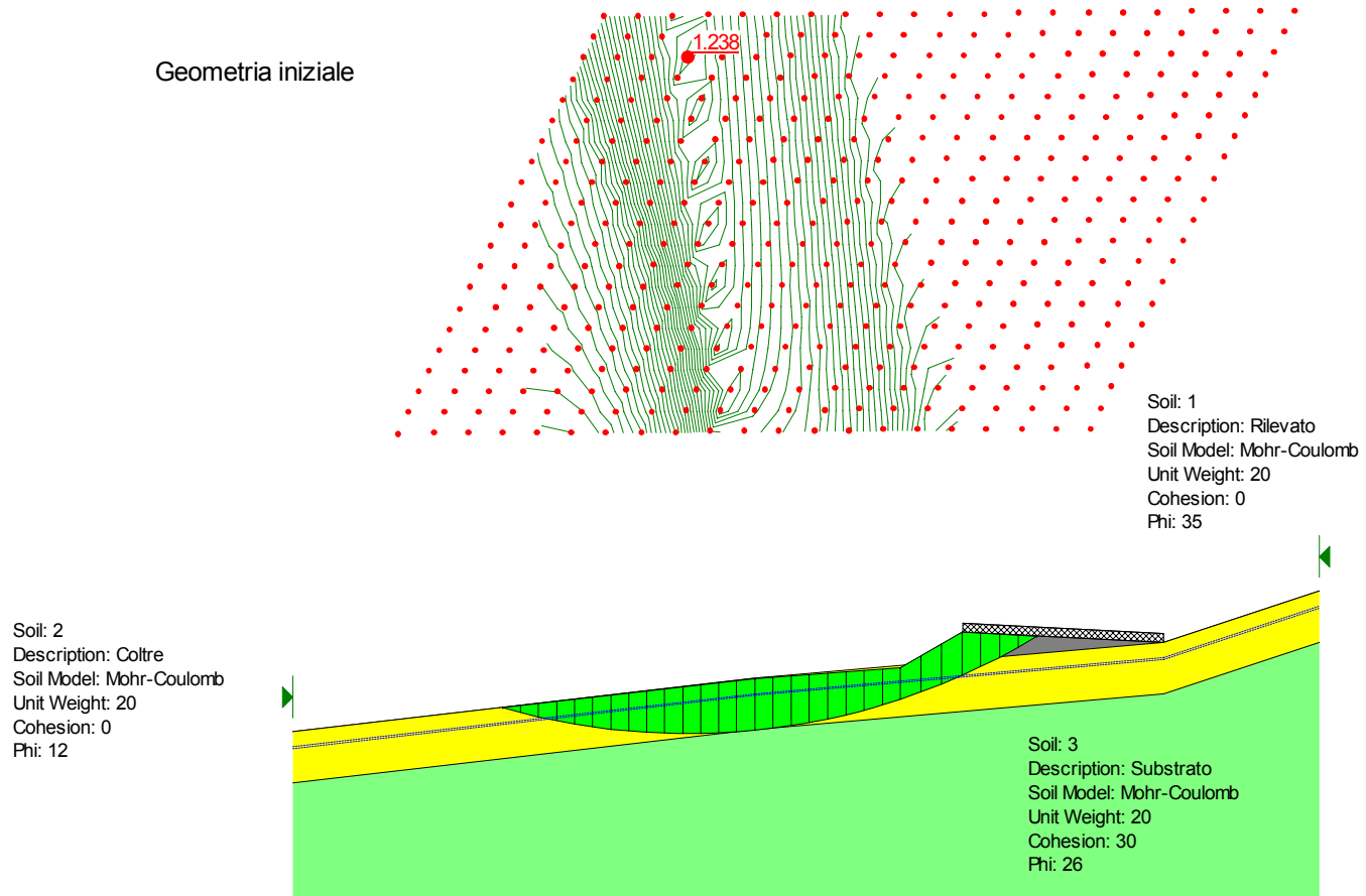
Figura 6.2- Analisi limite nelle condizioni iniziali per la definizione della superficie di rottura critica
