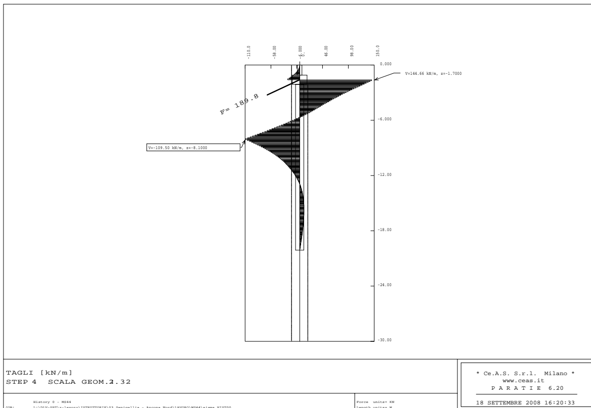
Figura 6.17 - Programma PARATIE – Fase di esercizio - Taglio
