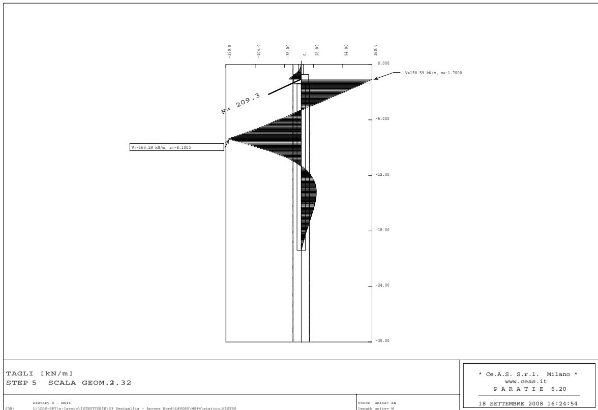
Figura 6.19 - Programma PARATIE – Fase SLU FS NEW – Taglio
