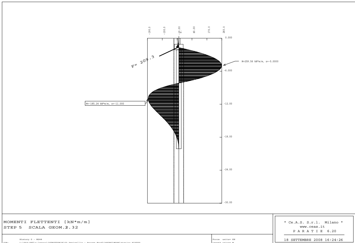
Figura 6.18 - Programma PARATIE – Fase SLU FS NEW – Momento flettente
