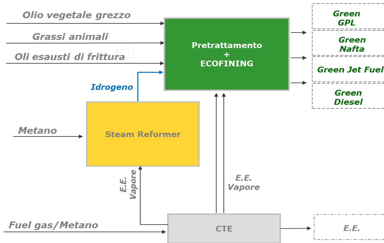
Schema a blocchi del ciclo produttivo "green" post operam
