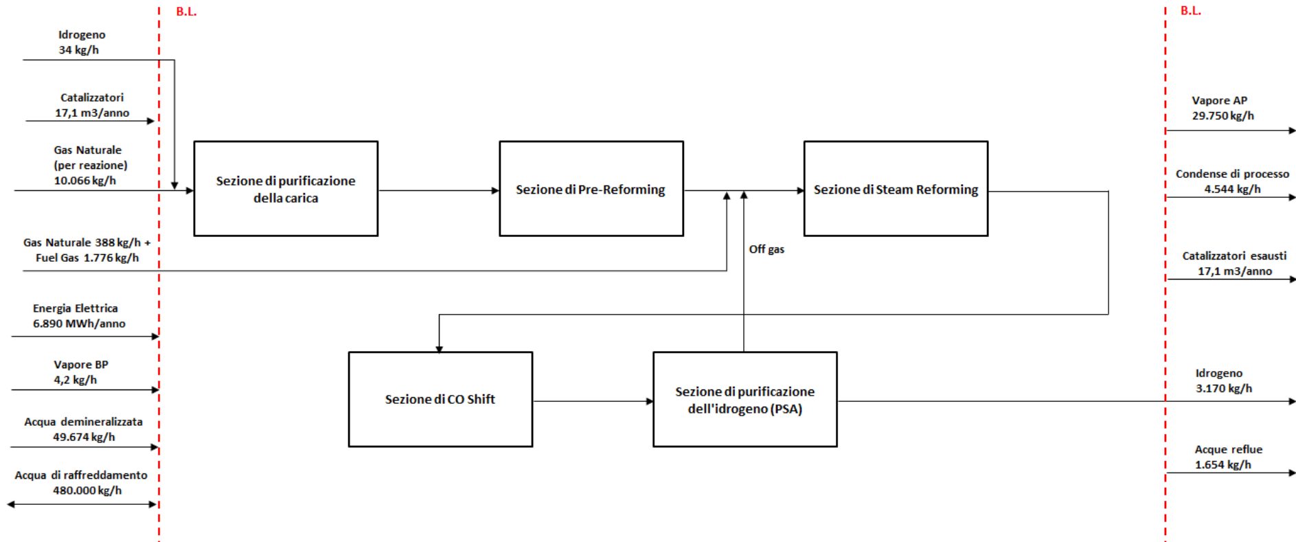
Schema semplificato della nuova unità Steam Reformer con le principali produzioni e consumi dell'impianto
