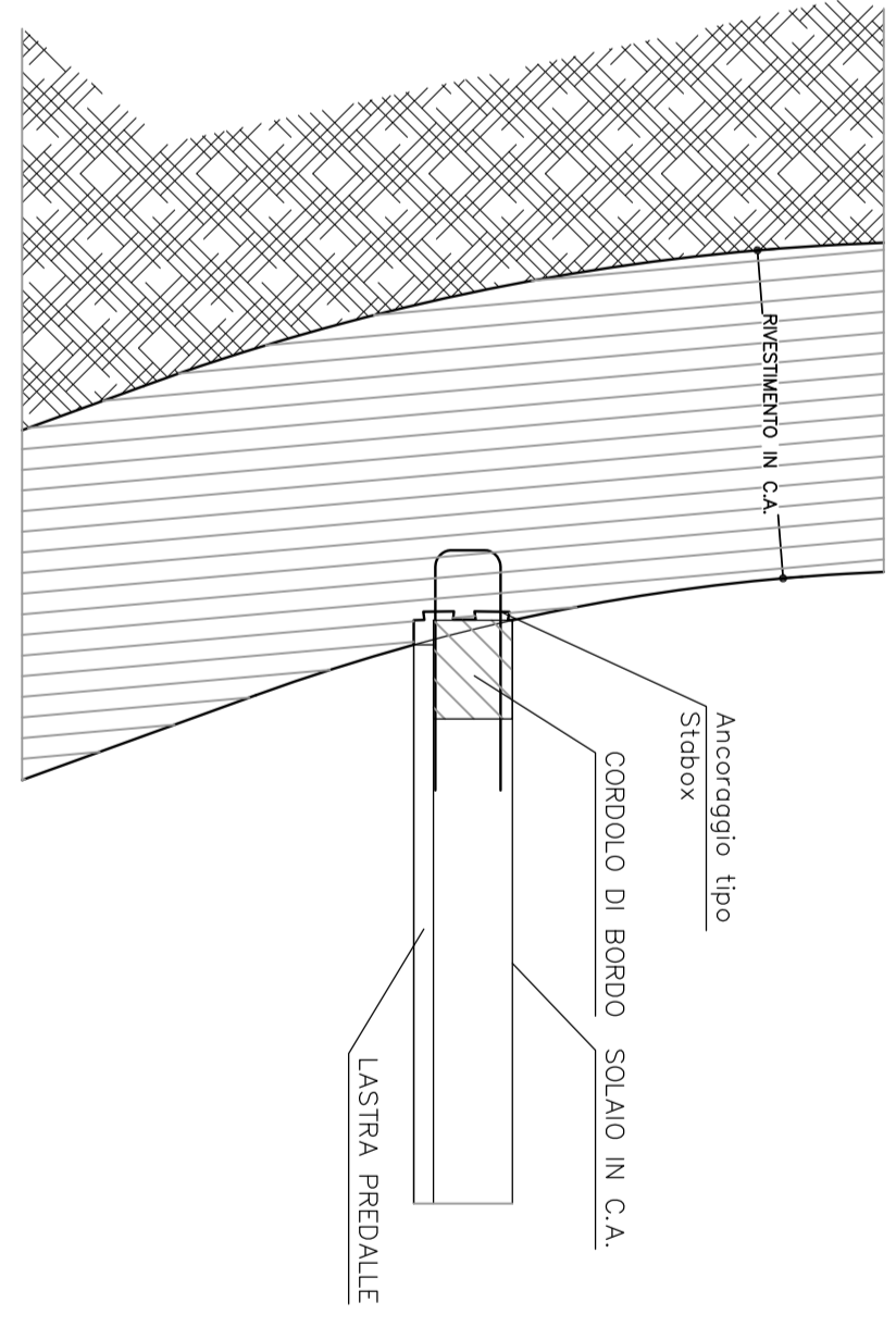
PARTICOLARE A SCALE 1:25
