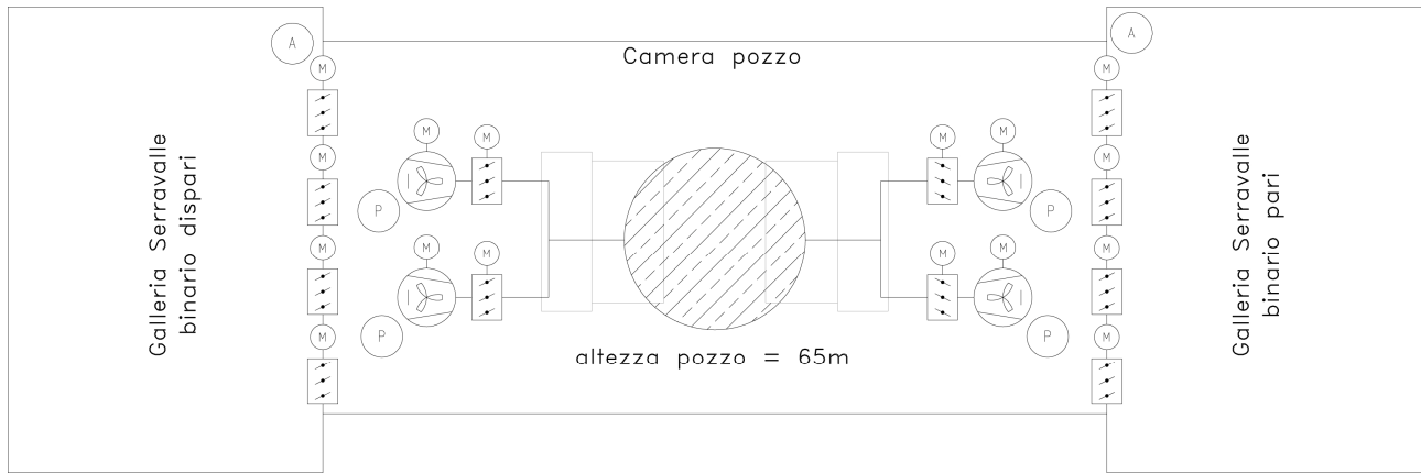
SCHEMA DI PRINCIPIO SCALA - POZZO DI VENTILAZIONE N.6 galleria Serravalle progr. 30+565
