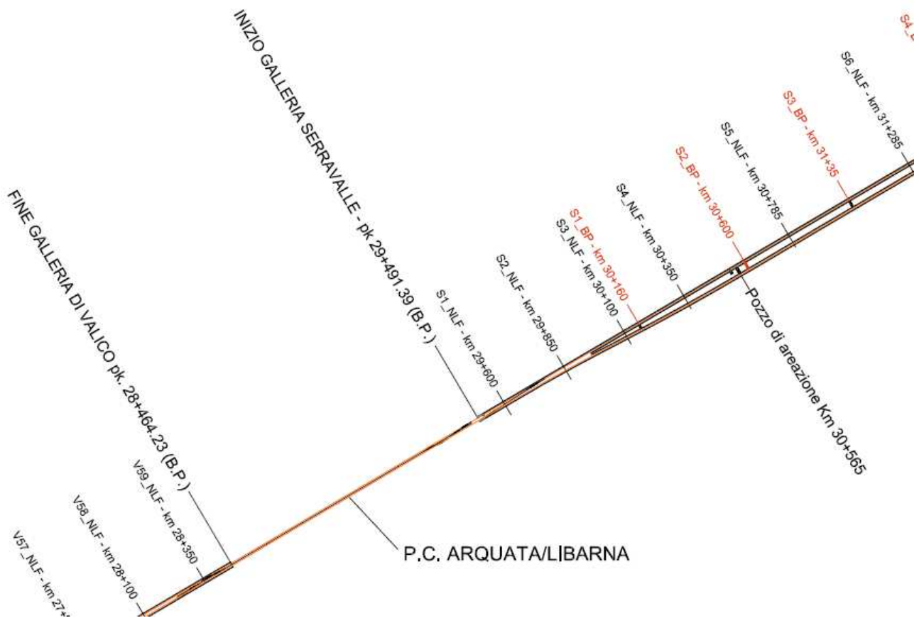
Planimetria localizzazione Pozzo n.6
