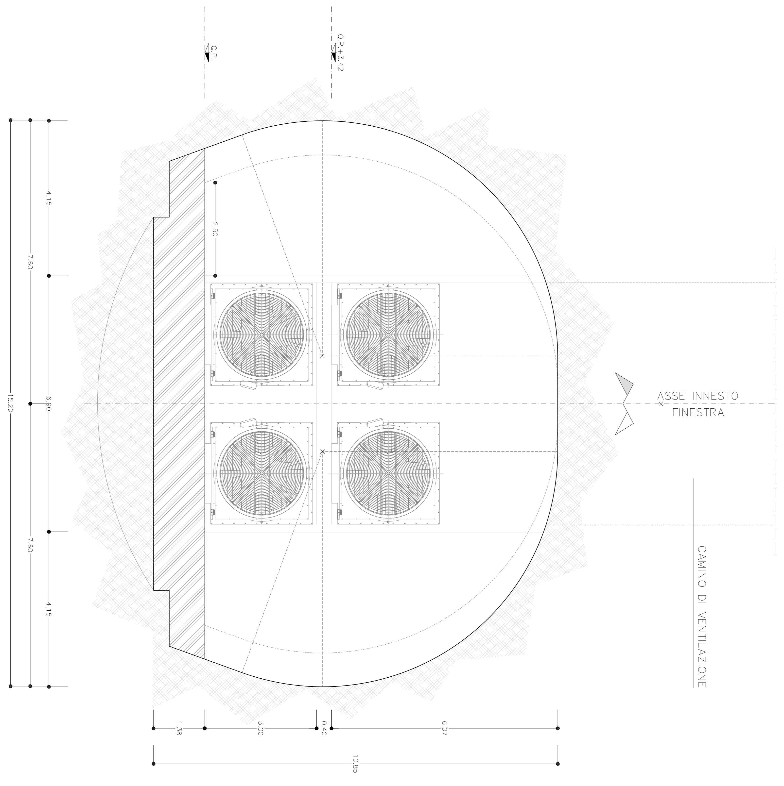
SEZIONE 15 SCALA 1:50 CENTRALE DI VENTILAZIONE SEZIONE IN ALLARGO
