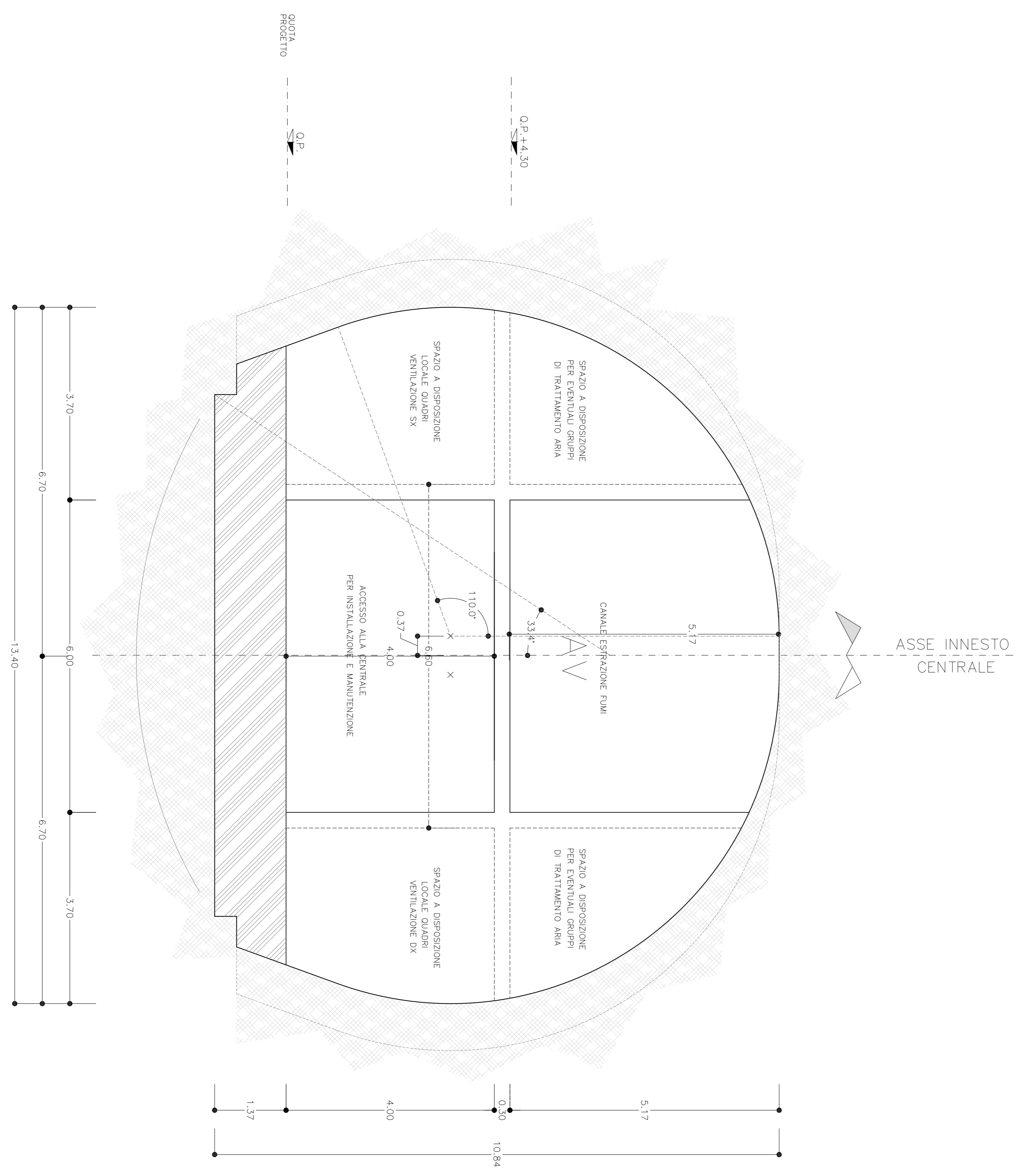
SEZIONE 14 SCALA 1:50 CENTRALE DI VENTILAZIONE SEZIONE TIPO
