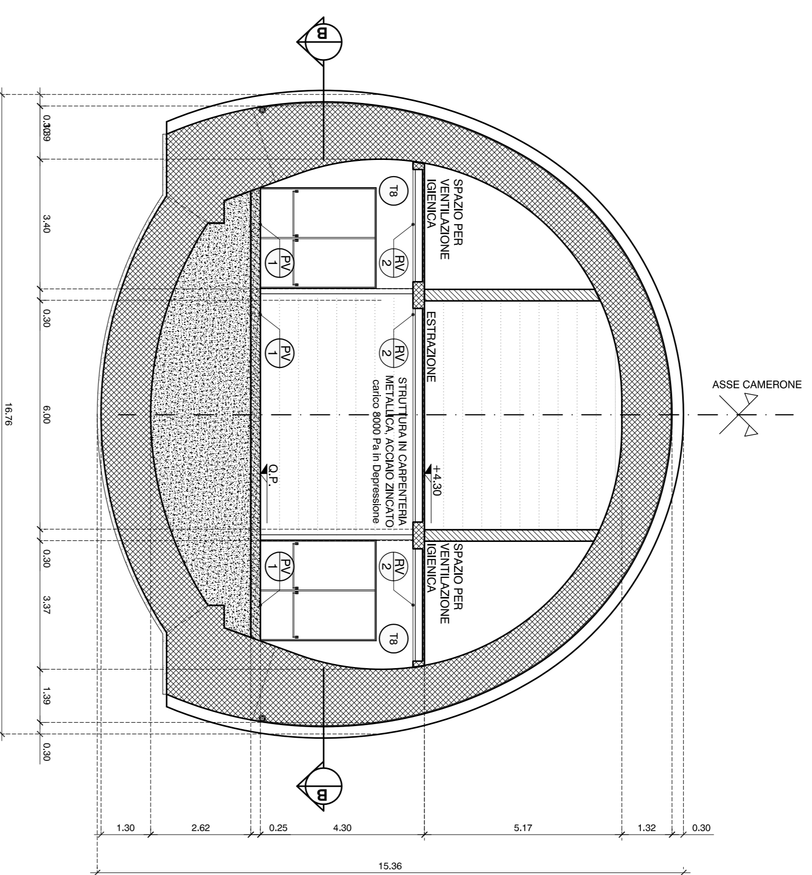
SEZIONE E - E SCALA 1:100
