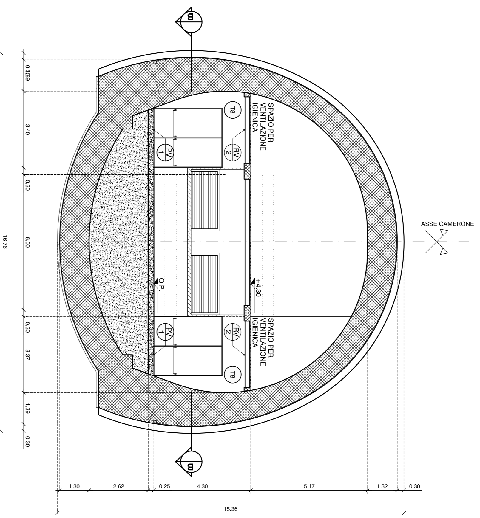
SEZIONE F - F SCALA 1:100
