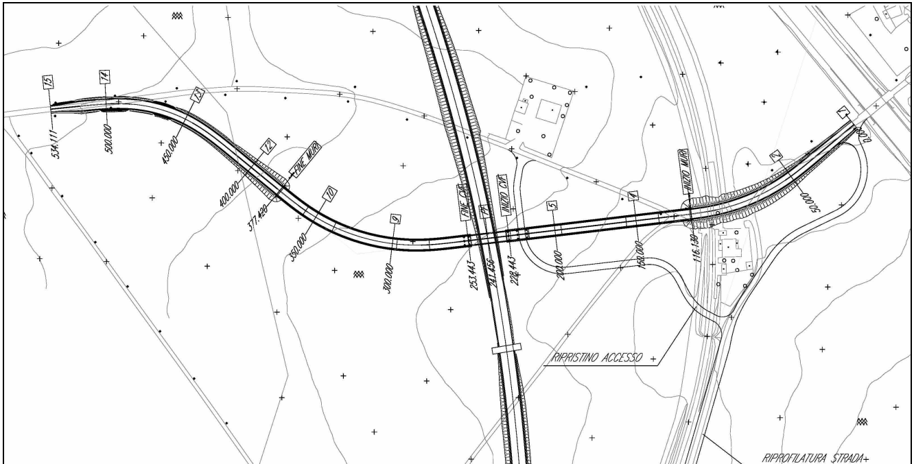
Figura 12 – NV07 – planimetria di progetto
