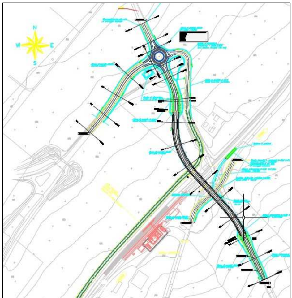
Figura 8 – NV05 – planimetria di progetto
