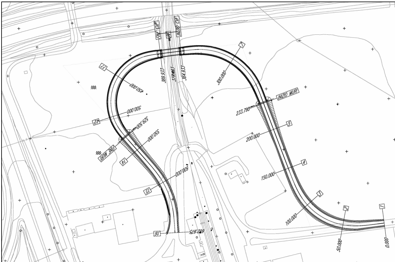
Figura 10 – NV06 – planimetria di progetto
