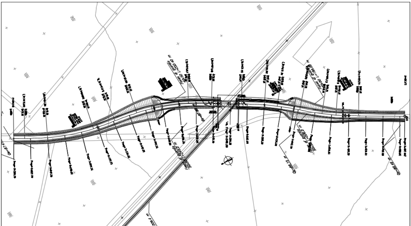
Figura 4 – NV02 – planimetria di progetto
