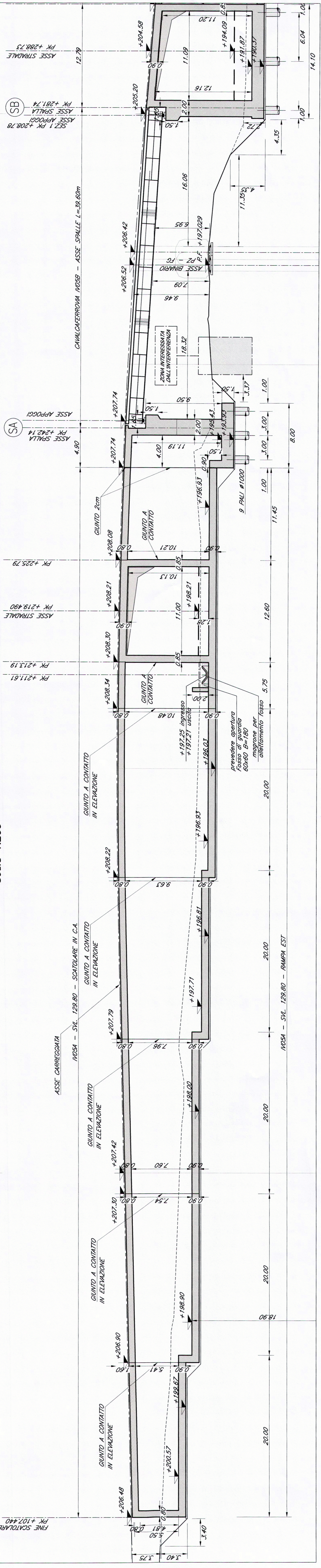
SEZIONE LONGITUDINALE (in asse) Scala 1:200
