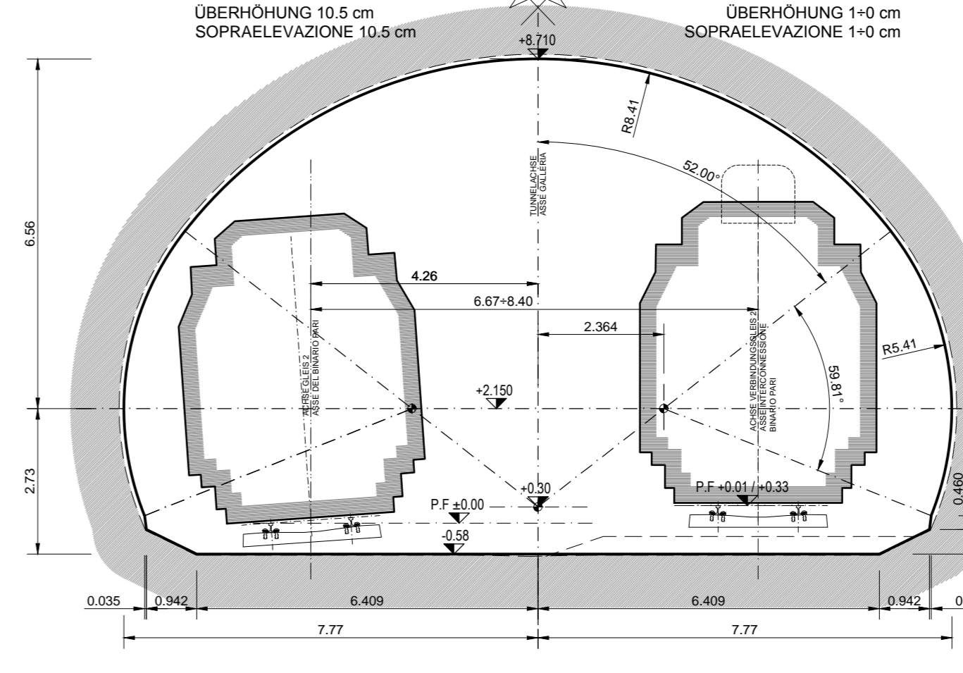
GALLERIA PRINCIPALE A DOPPIO BINARIO INTERASSE BINARI 6,67+8,40m (Tipo "N2 - TP-PC3")
