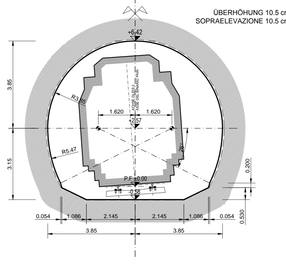
GALLERIA PRINCIPALE A SINGOLO BINARIO (Tipo "S1 - TP - IS")
