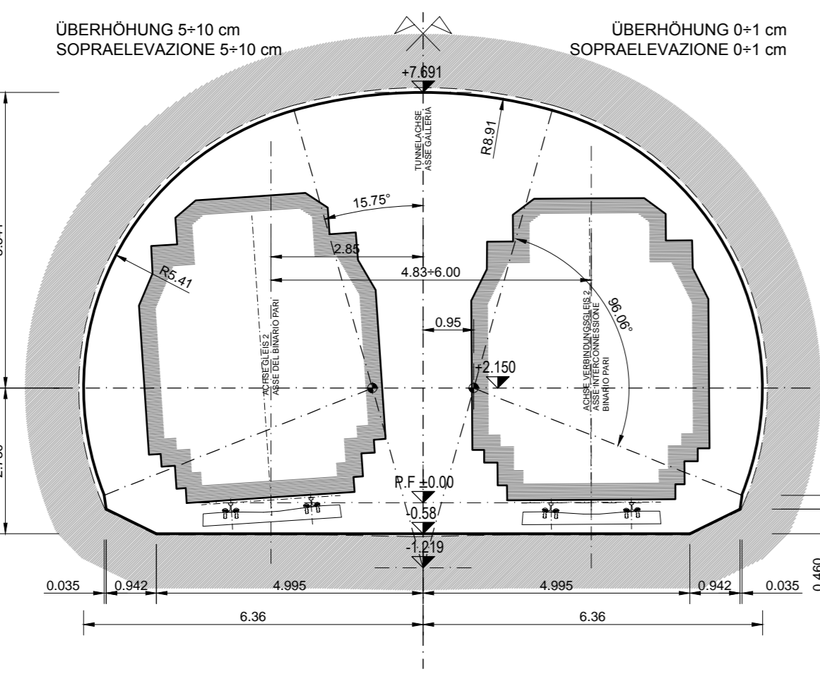
GALLERIA PRINCIPALE A DOPPIO BINARIO INTERASSE BINARI 4,83+6,00m (Tipo "N2-TP-6.0")
