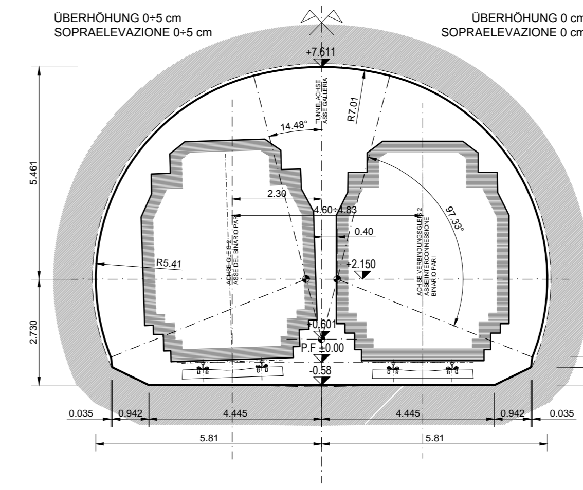
GALLERIA PRINCIPALE A DOPPIO BINARIO INTERASSE BINARI 4,60+4,83m (Tipo "N2-TP-4.9")
