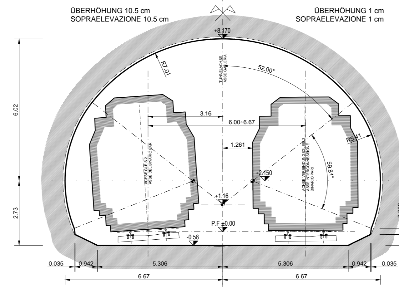
GALLERIA PRINCIPALE A DOPPIO BINARIO INTERASSE BINARI 6,00+6,67m (Tipo "N2 - TP-PC2")
