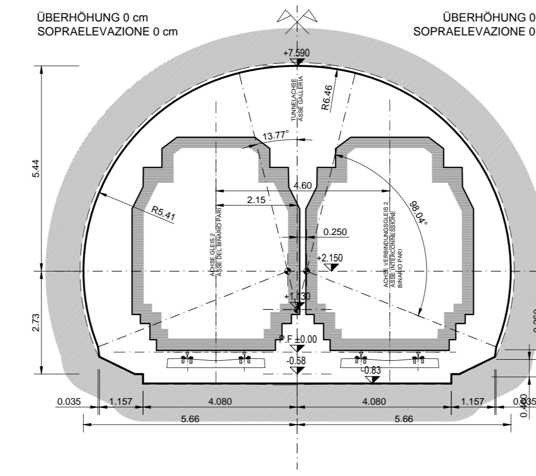
GALLERIA PRINCIPALE A DOPPIO BINARIO INTERASSE BINARI 4,60m SISTEMA A MASSE FLOTTANTI (Tipo "N2-TP-SMF-4.6")
