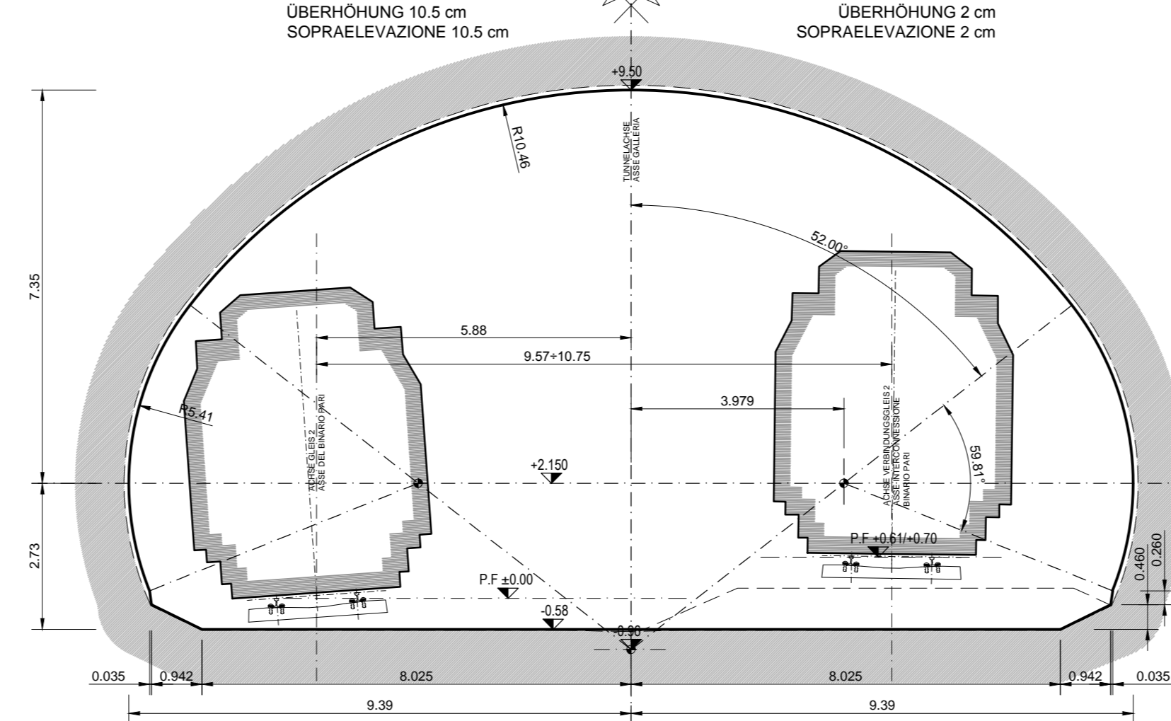
GALLERIA PRINCIPALE A DOPPIO BINARIO INTERASSE BINARI 9,57+10,75m (Tipo "N2 - TP-PC5")
