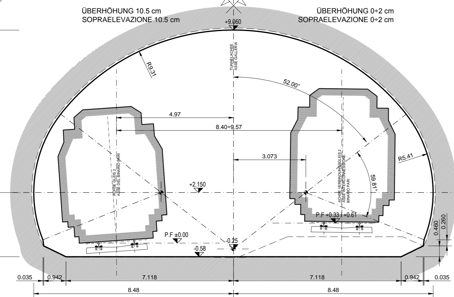
GALLERIA PRINCIPALE A DOPPIO BINARIO INTERASSE BINARI 8,40+9,57m (Tipo "N2 - TP-PC4")
