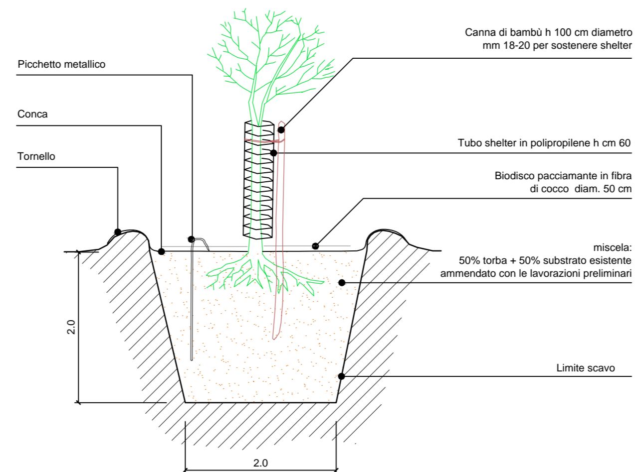
Modalità di impianto specie arboree e arbustive in fitocelle anni 2 scala 1:50
