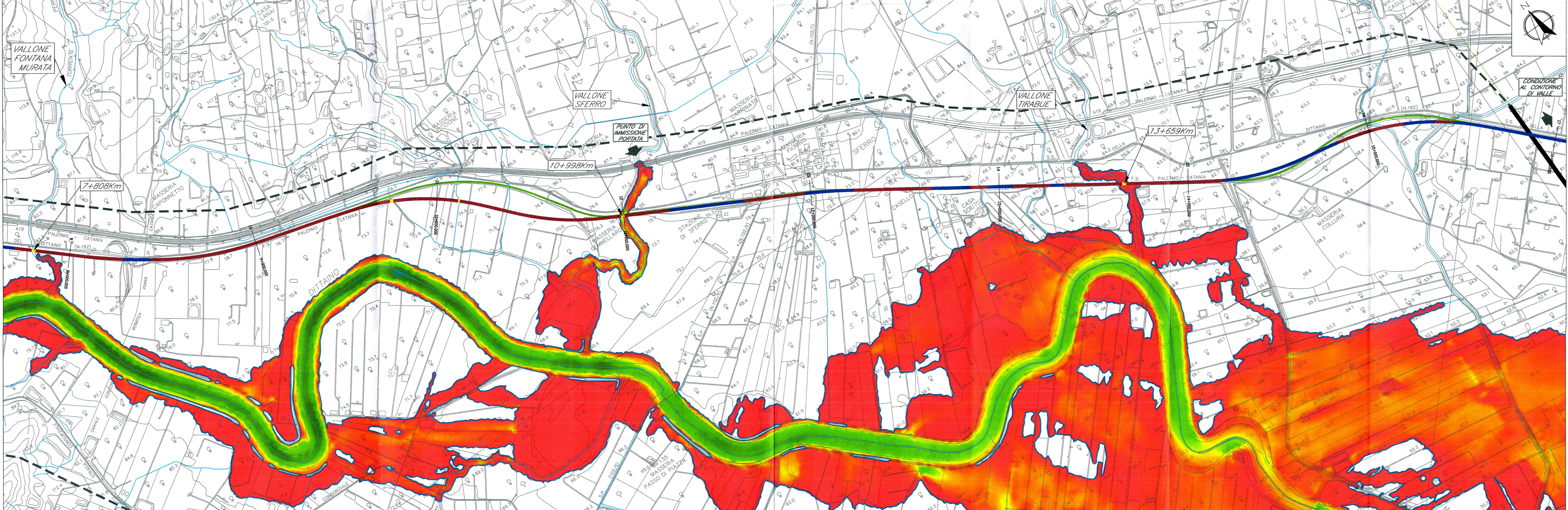
Riquadro 05 - Planimetria degli allagamenti e velocità - TR 50 anni - scala 1:10'000
