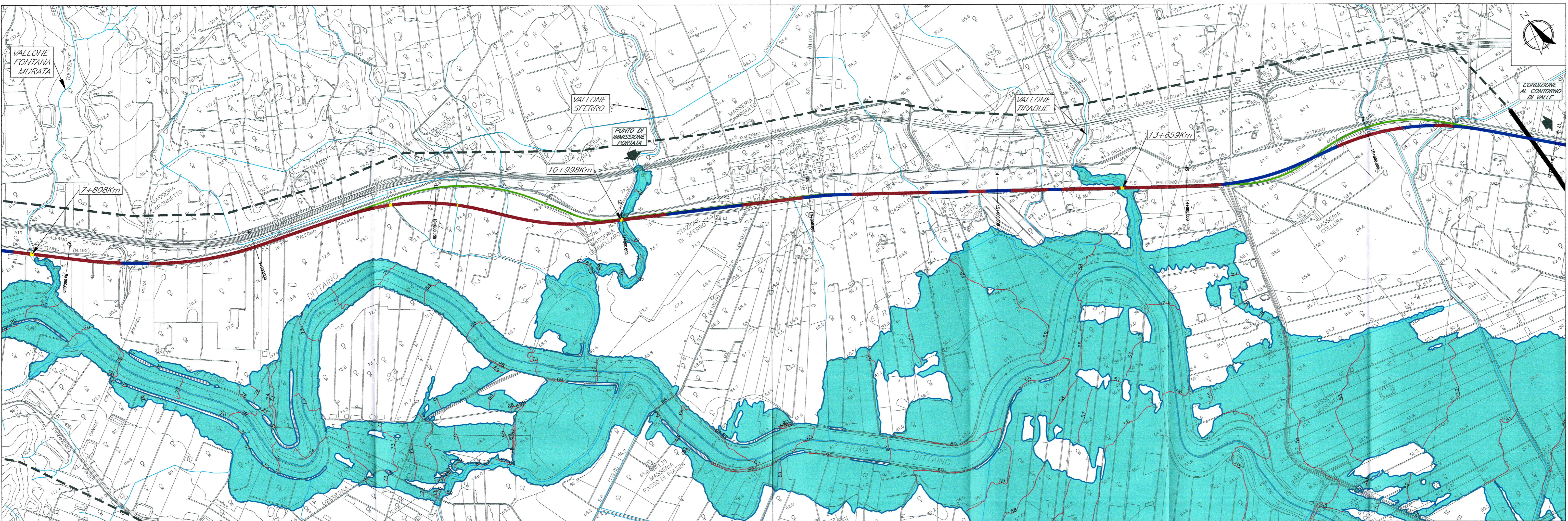
Riquadro 05 - Planimetria degli allagamenti e livelli idrici - TR 50 anni - scala 1:10'000
