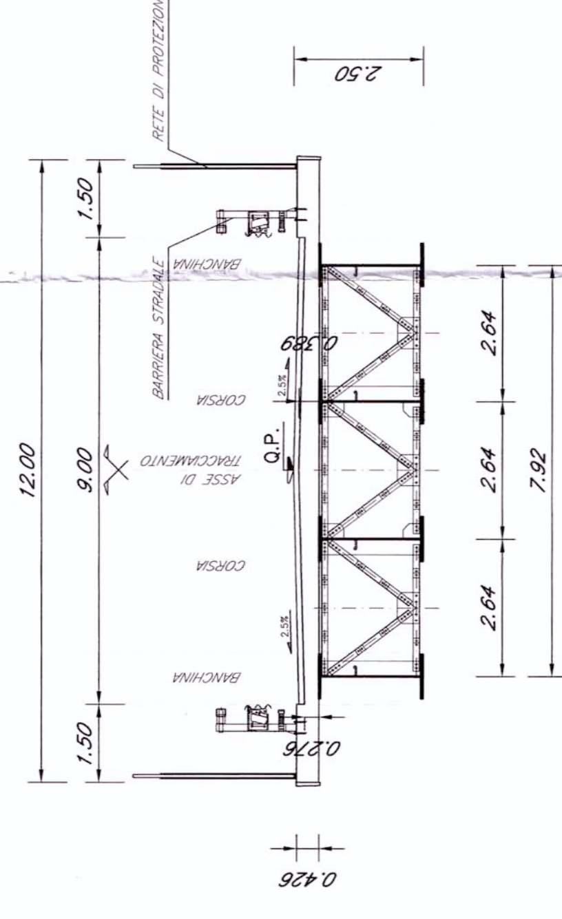
Sezione strada tipo F1 Comparto L=55+35 m
