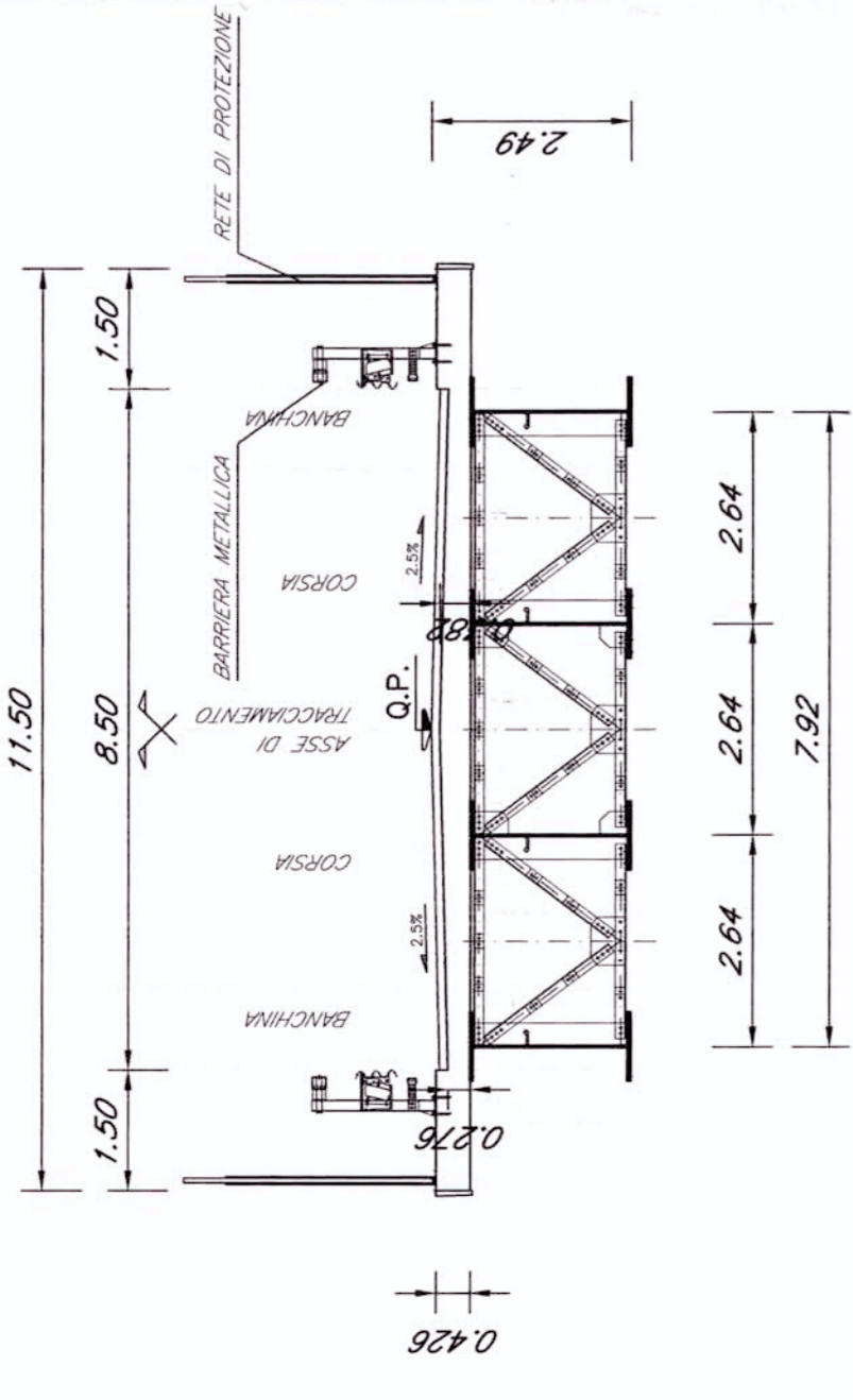
Sezione strada tipo F2 Compatta L= 26 m
