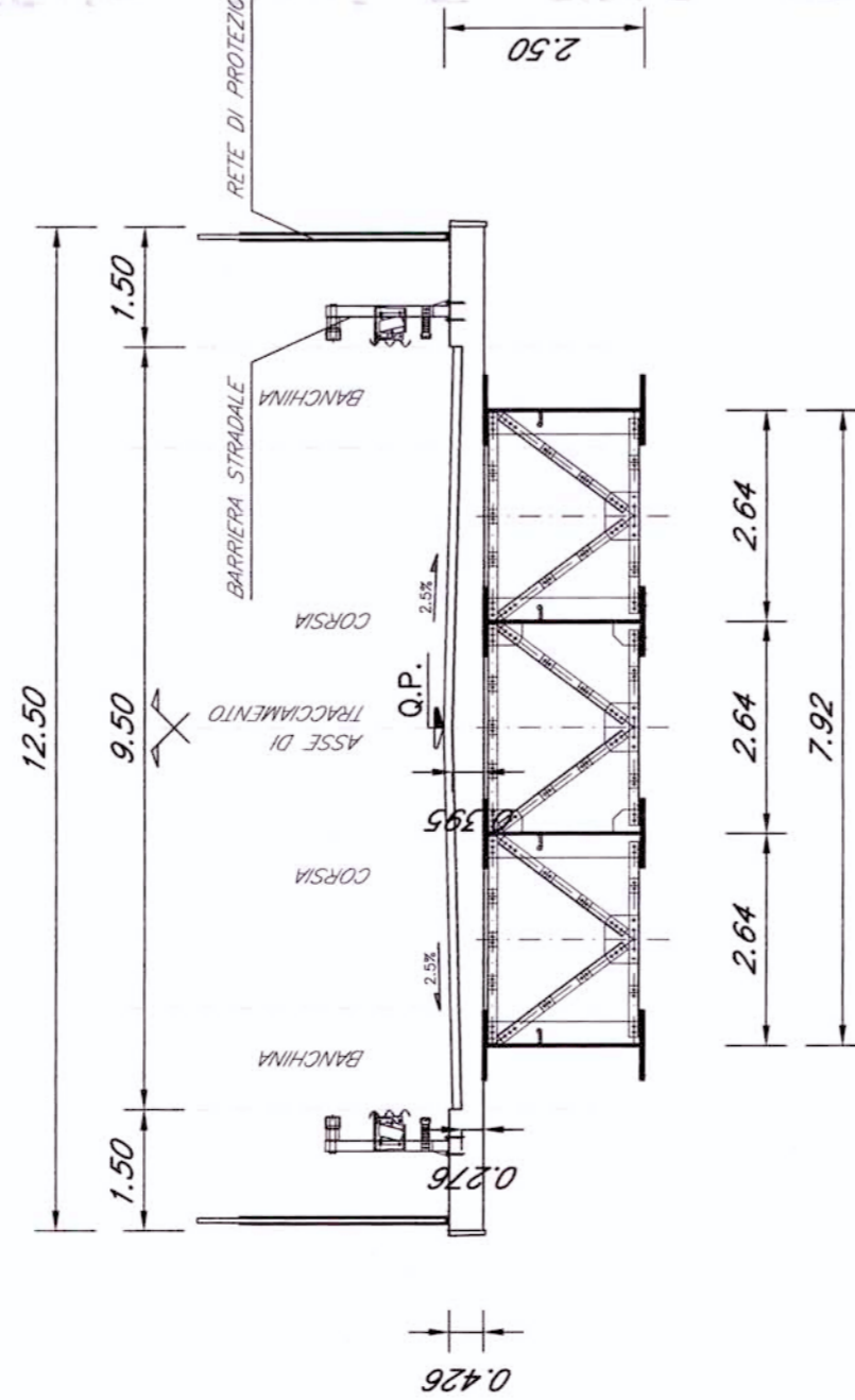
Sezione strada tipo C2 Compatta L= 26 m
