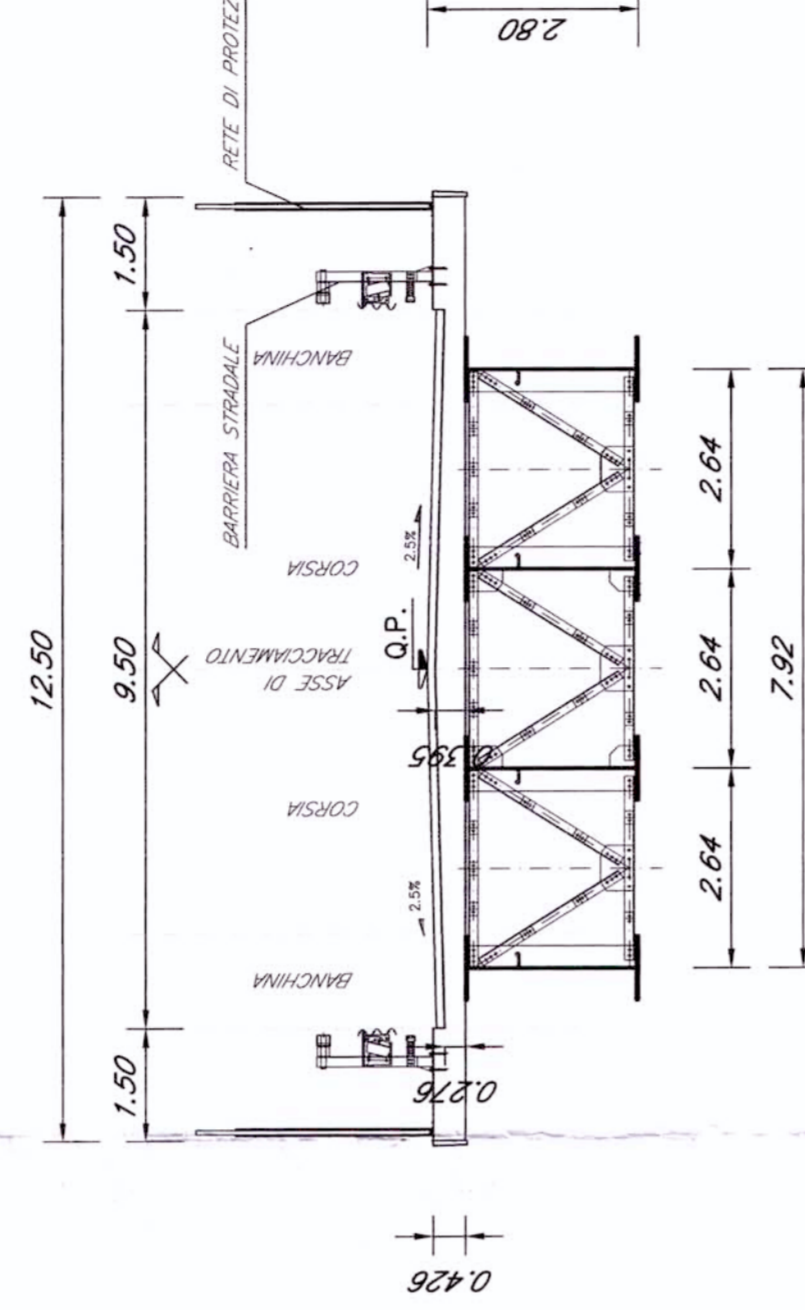
Sezione strada tipo C2 Compatta L= 40 m
