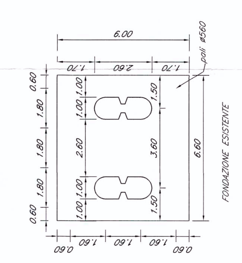
PIANTA FONDAZIONE STATO ATTUALE - Scala 1:100
