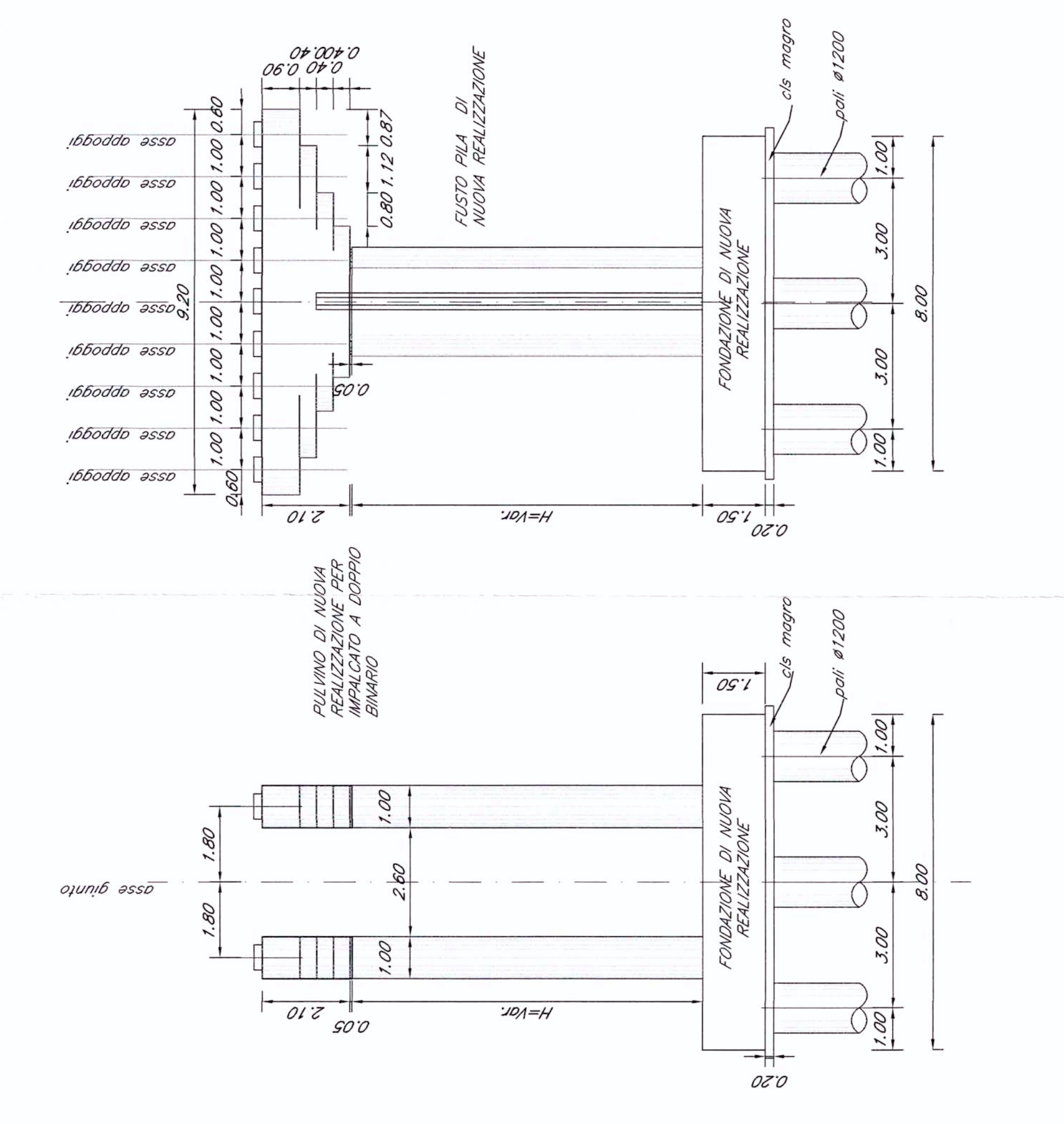
PROSPETTI NUOVE PILE - Scala 1:100
