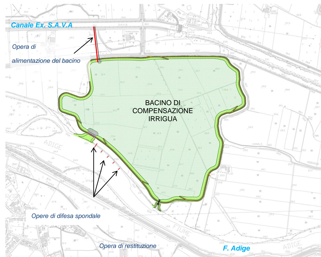
Fig. 5-1: Planimetria delle opere in progetto.
