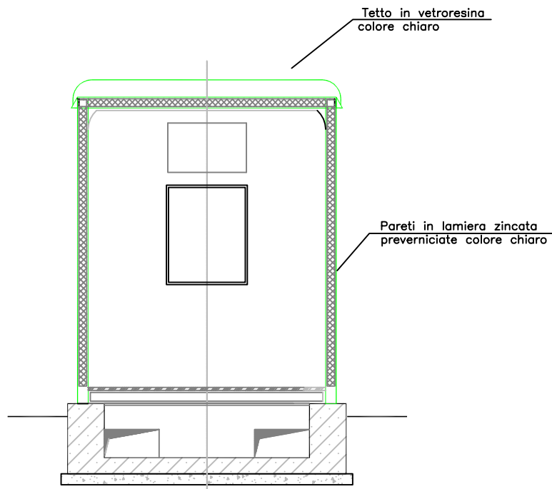
SEZIONE W-W
