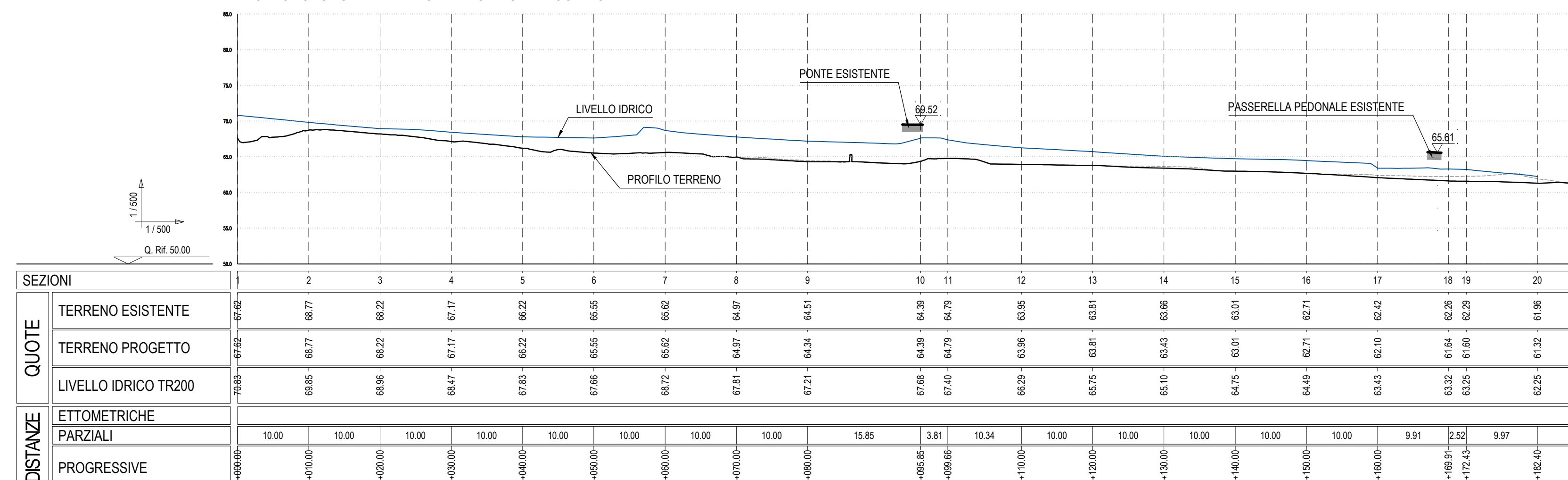
PROFLO LONGITUDINALE BIANCHETTA STATO DI PROGETTO
