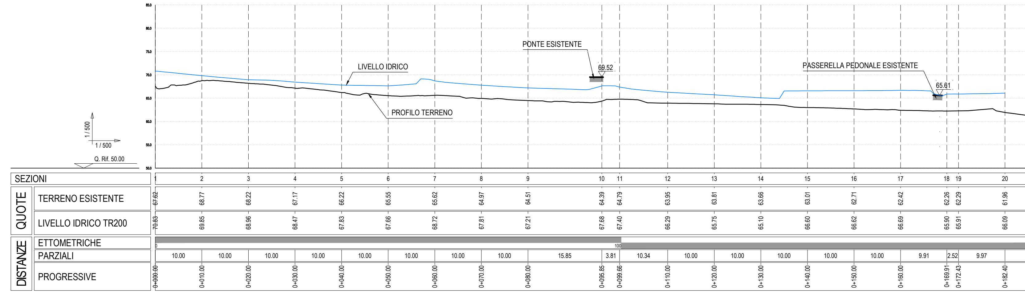
PROFLO LONGITUDINALE BIANCHETTA STATO DI FATTO
