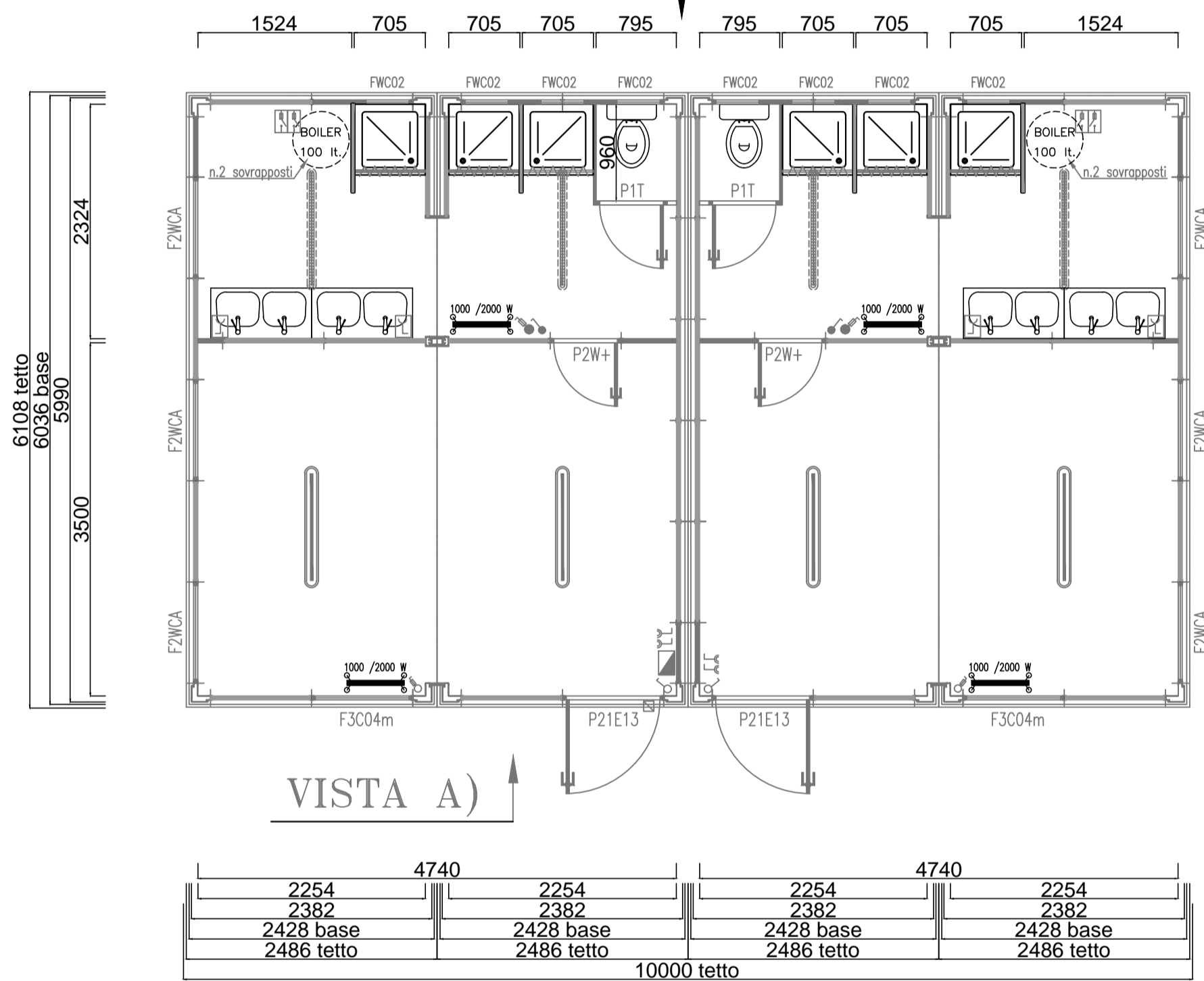
PIANTA
