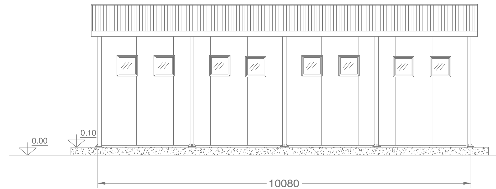
VISTA C)
