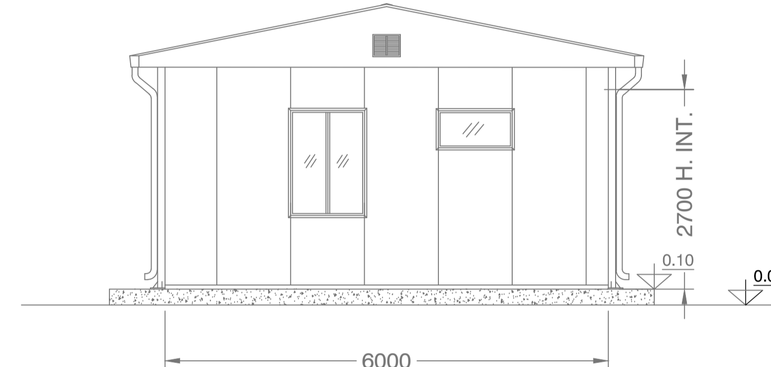
VISTA B)
