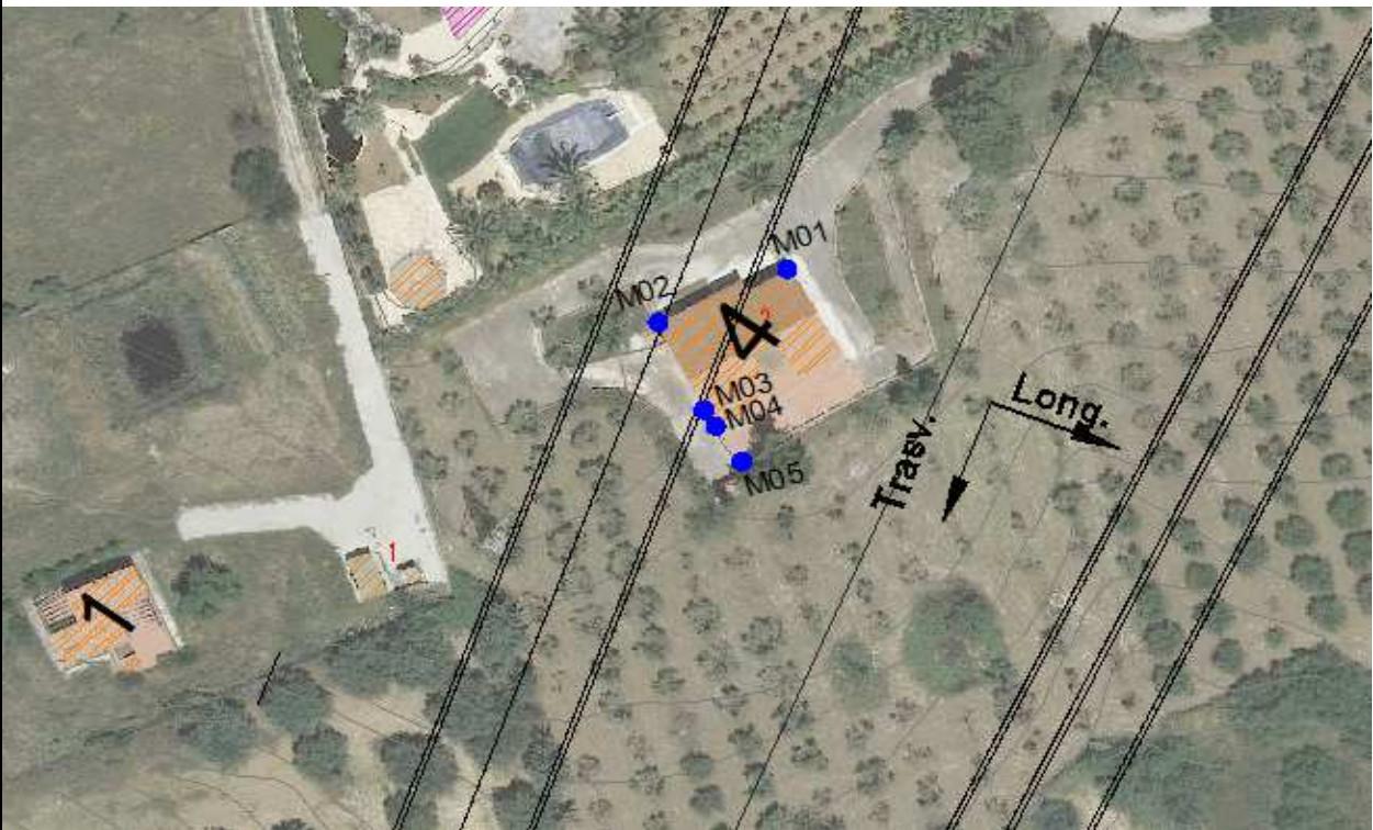
STRALCIO PLANIMETRICO CON INDICAZIONE STRUMENTAZIONE MONITORATA
