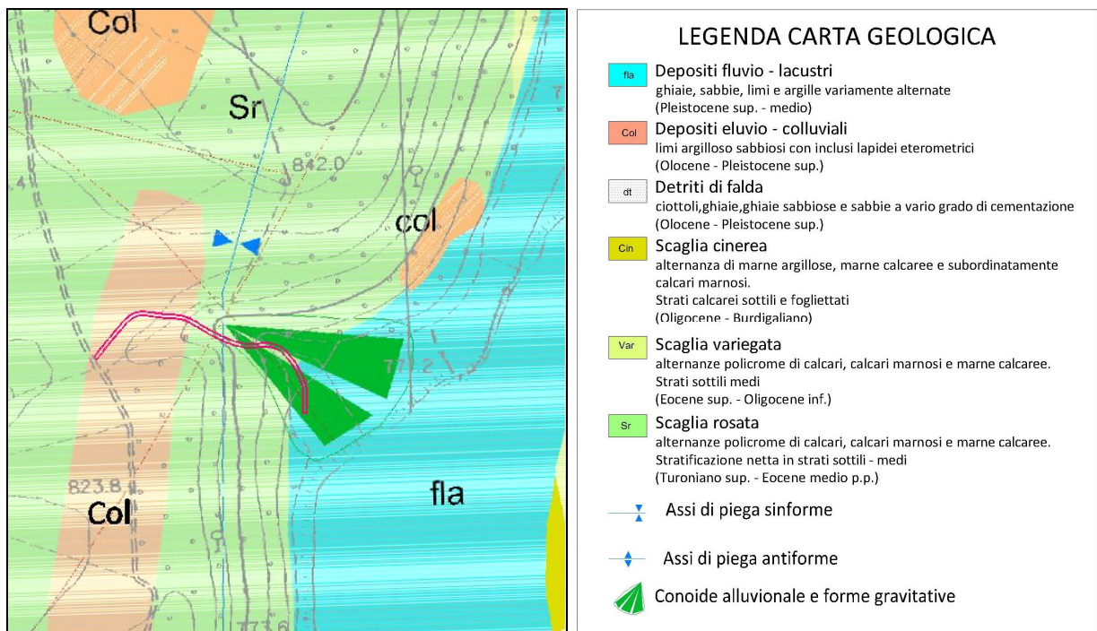
Figura 5 – Stralcio della Carta geologica della strada di cantiere.
