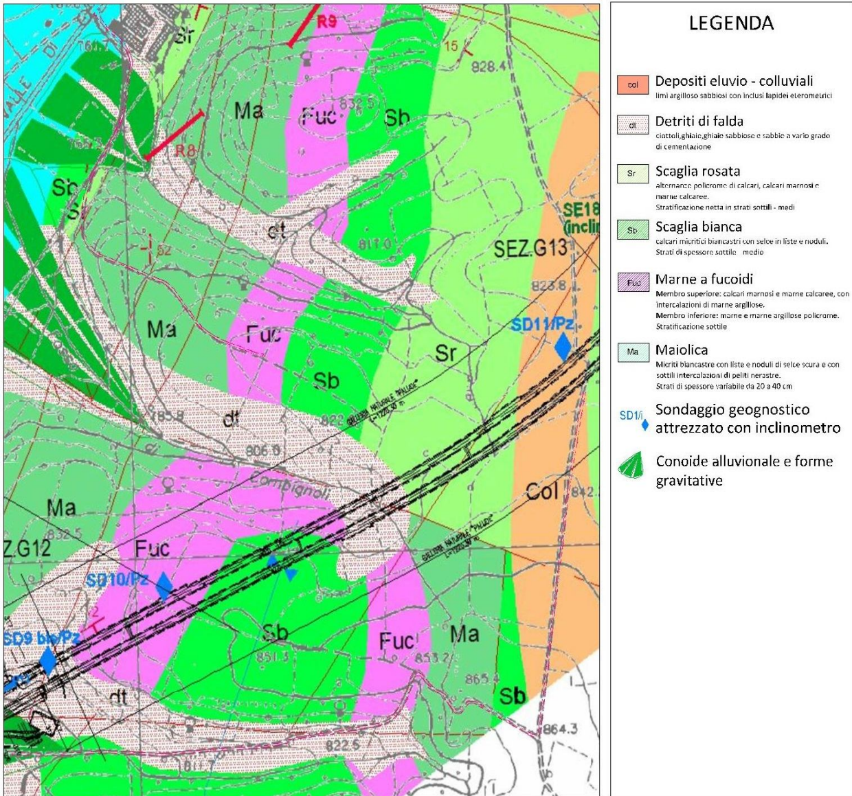
Figura 5 – Stralcio della Carta geologica della strada di cantiere.
