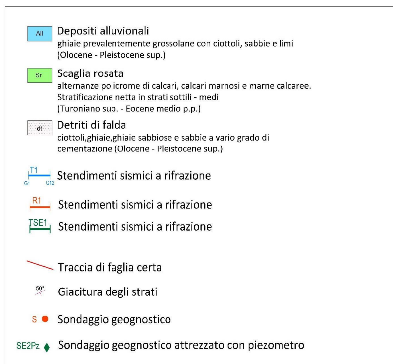
Figura 5 – Stralcio della Carta geologica della strada di cantiere.
