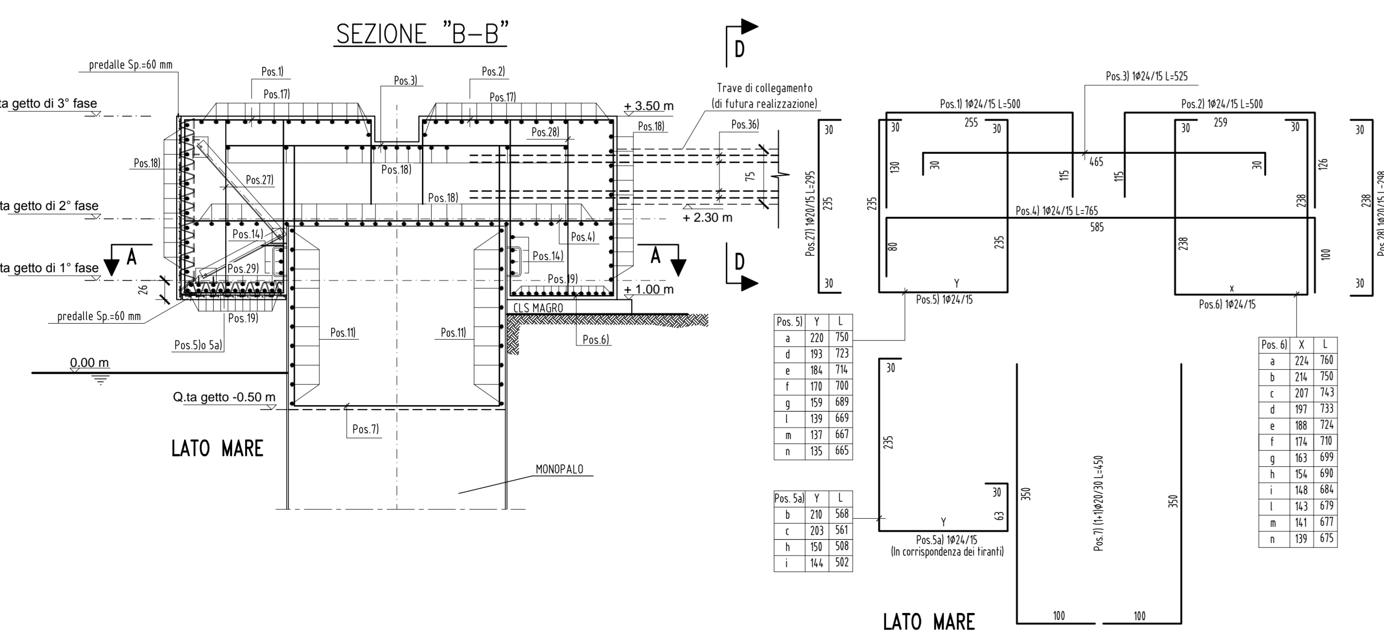
SEZIONE SUI MONOPALI scala 1:50
