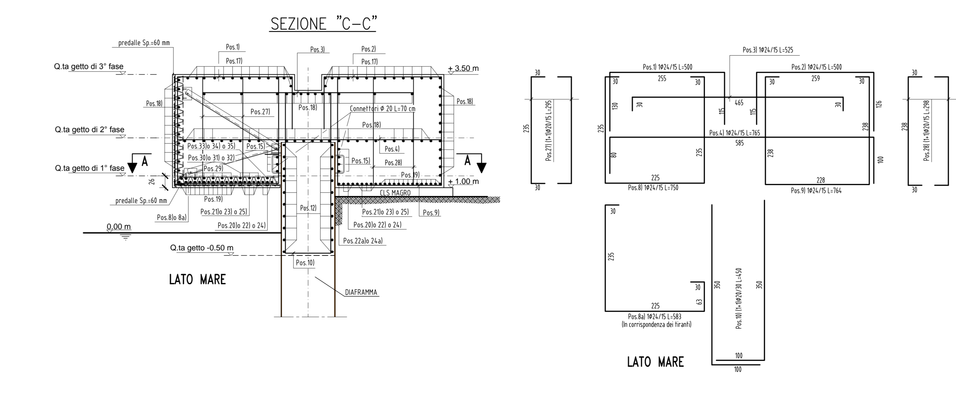
SEZIONE SUL DIAFRAMMA scala 1:50
