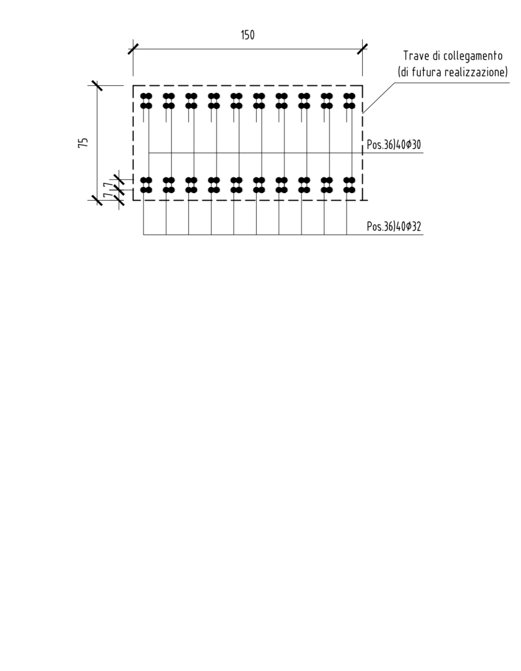
SEZIONE "D-D" scala 1:25
