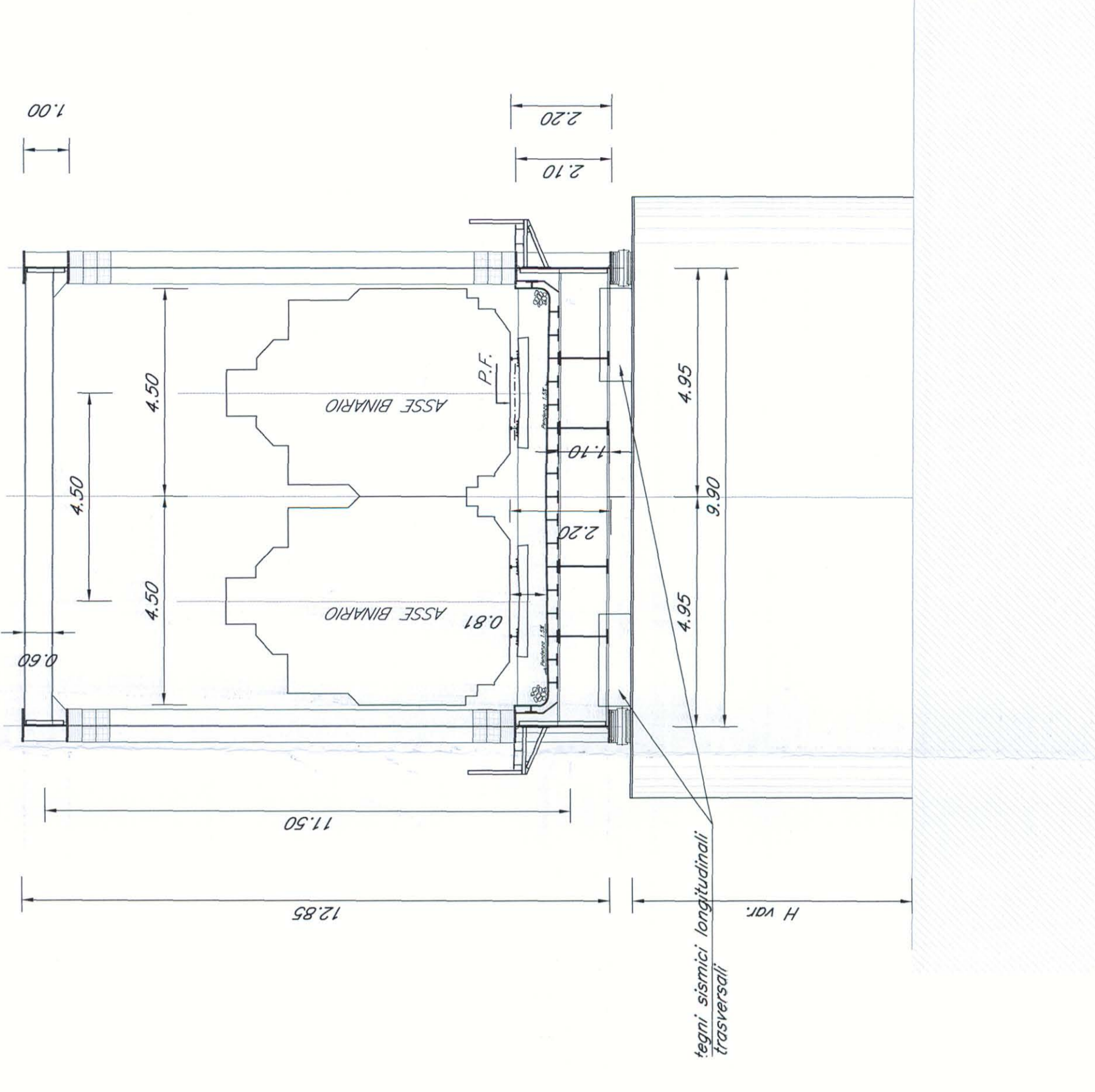
SEZIONE TRASVERSALE scala 1:100
