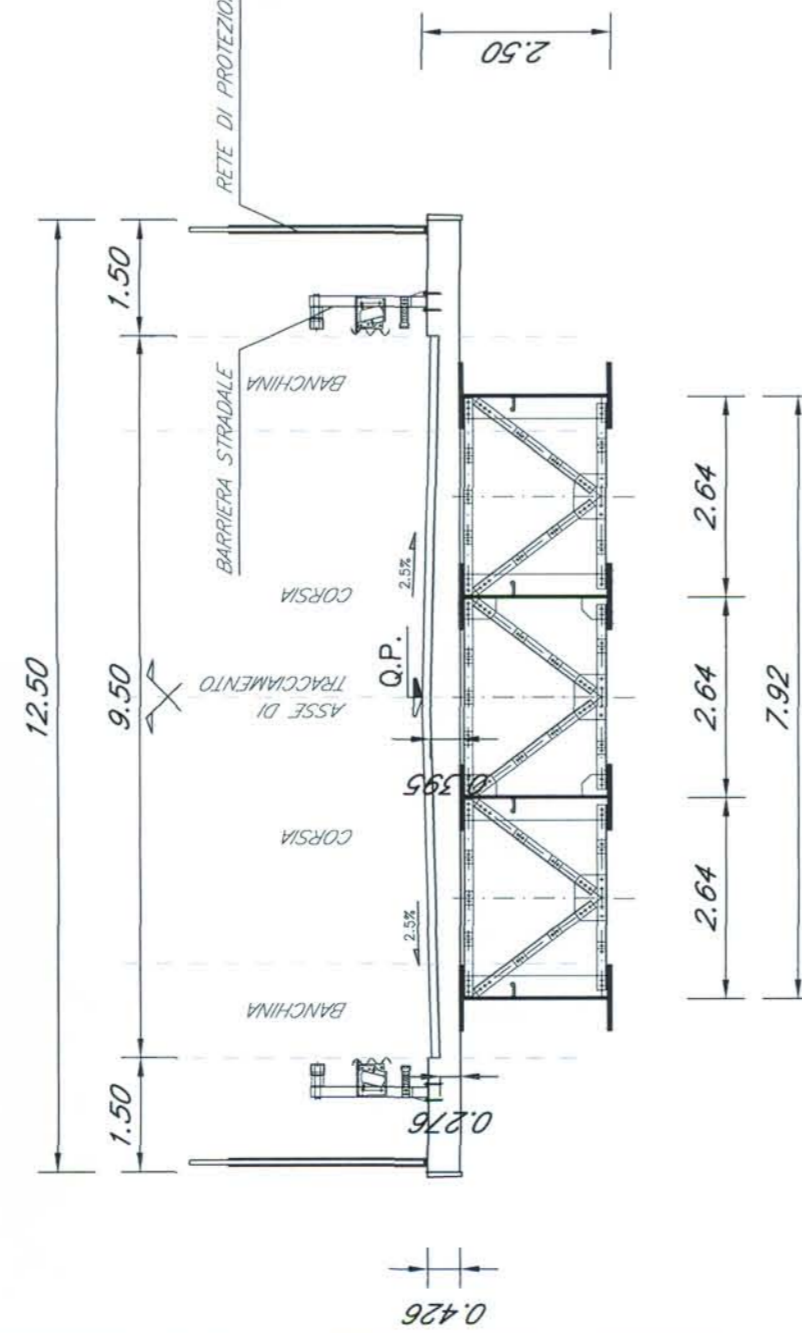
Sezione strada tipo C2 Compata L= 26 m
