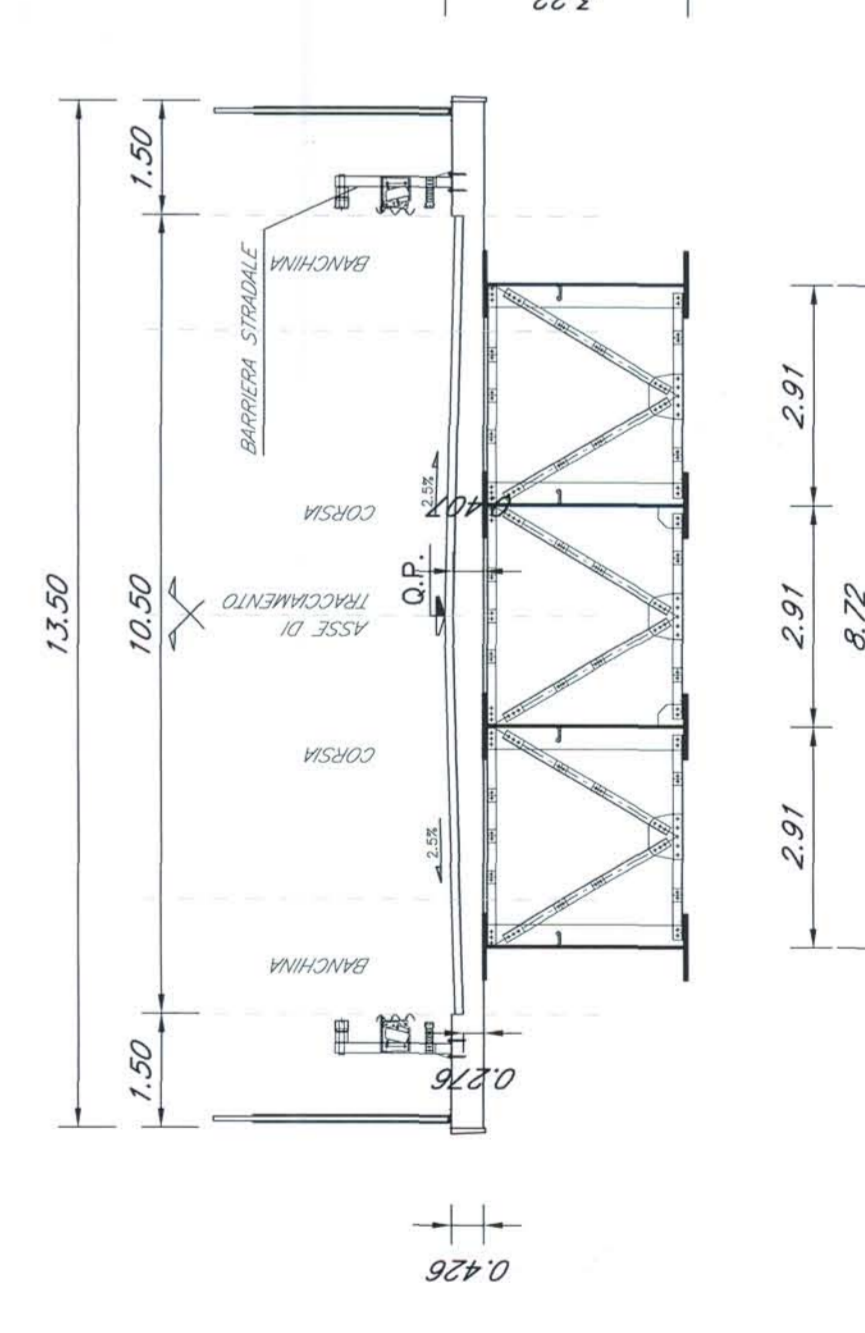
Sezione strada tipo C1 Compata L=50 m
