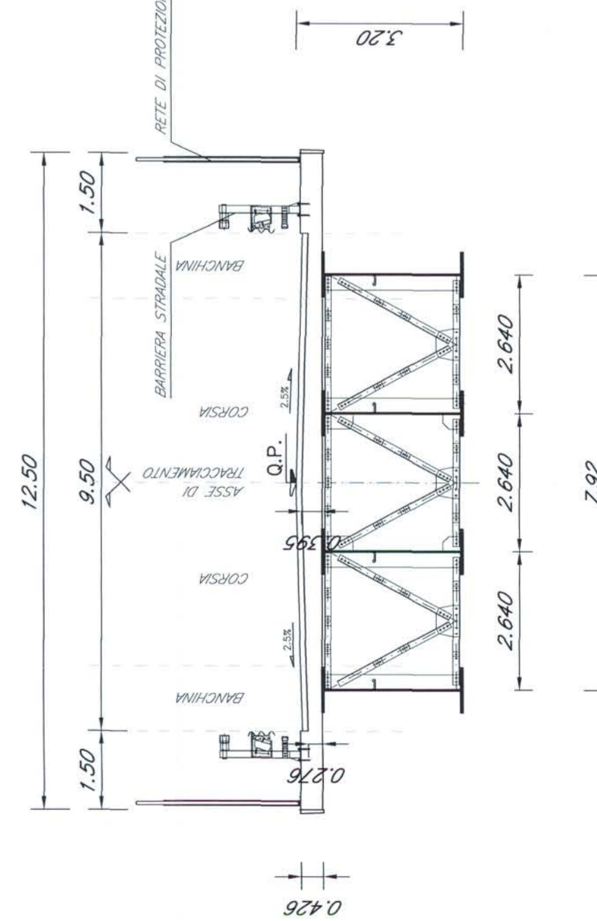
Sezione strada tipo C2 Compata L=50 m
