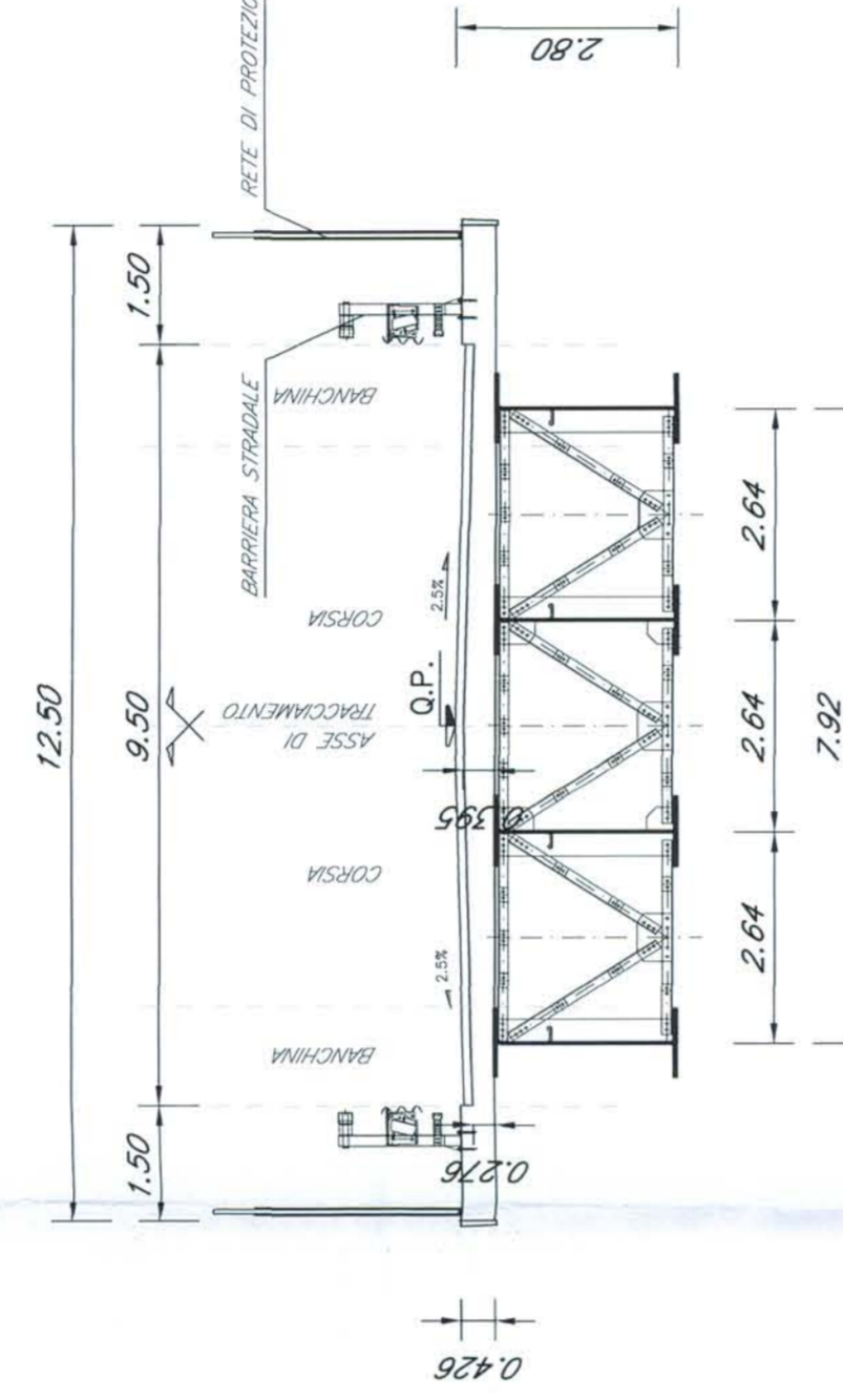
Sezione strada tipo C2 Compata L= 40 m
