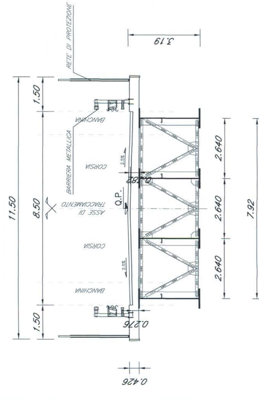
Sezione strada tipo F2 Compata L=50 m
