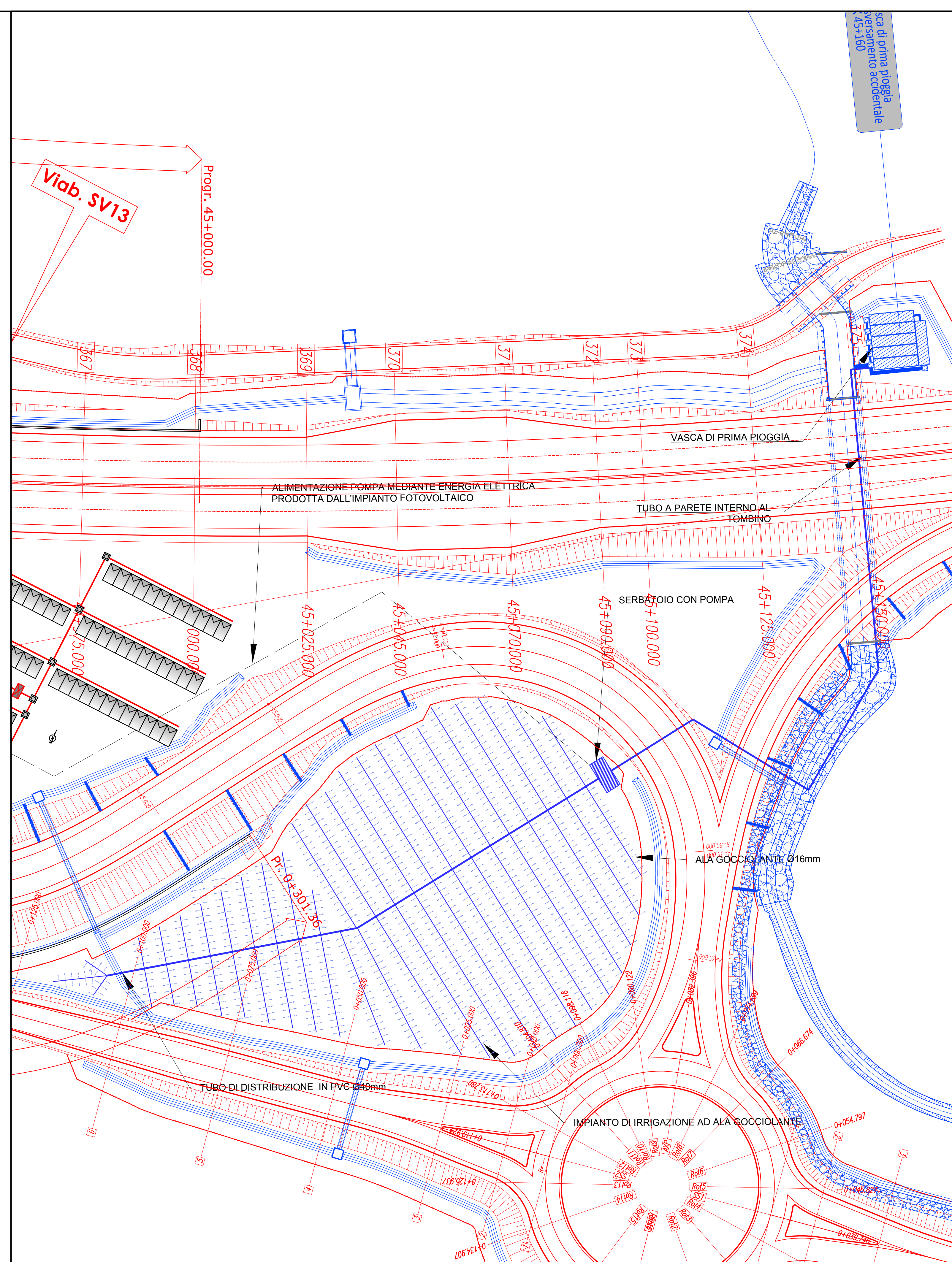
SCHEMA IMPIANTO DI IRRIGAZIONE - SVINCOLO DI BERCHIDDA
