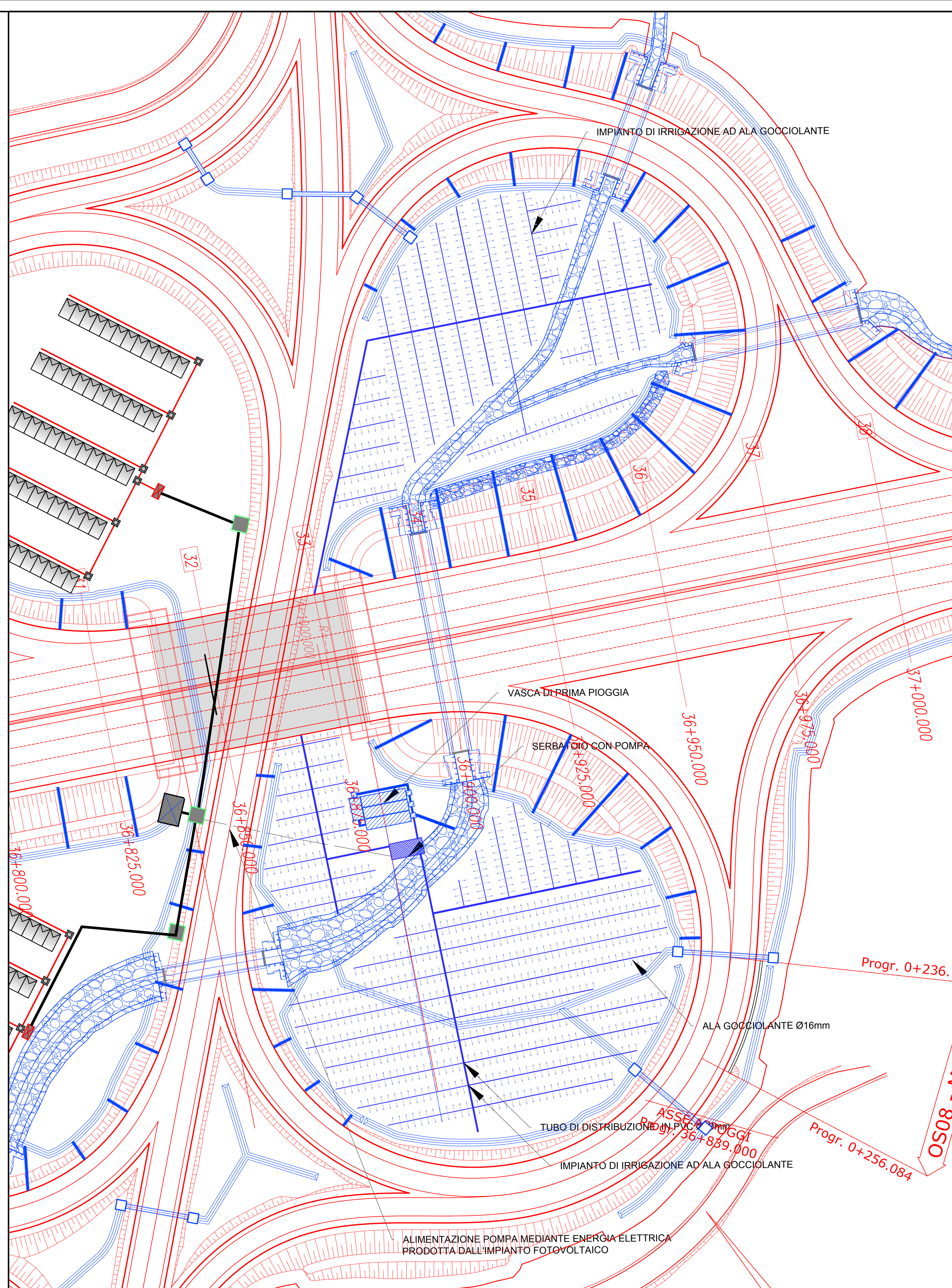
SCHEMA IMPIANTO DI IRRIGAZIONE - SVINCOLO DI OSCHIRI
