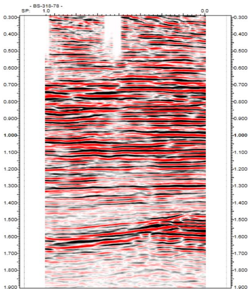
Figura 2.8 Linea sismica BS-317-81 attraverso la struttura e ubicazione del pozzo
