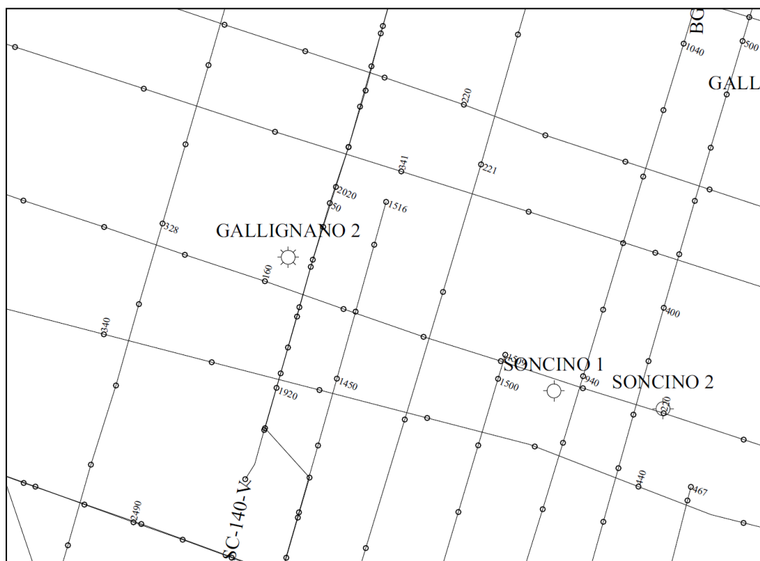
Figura 2.7 Isocrono del Top della Formazione Sabbie di Caviaga
