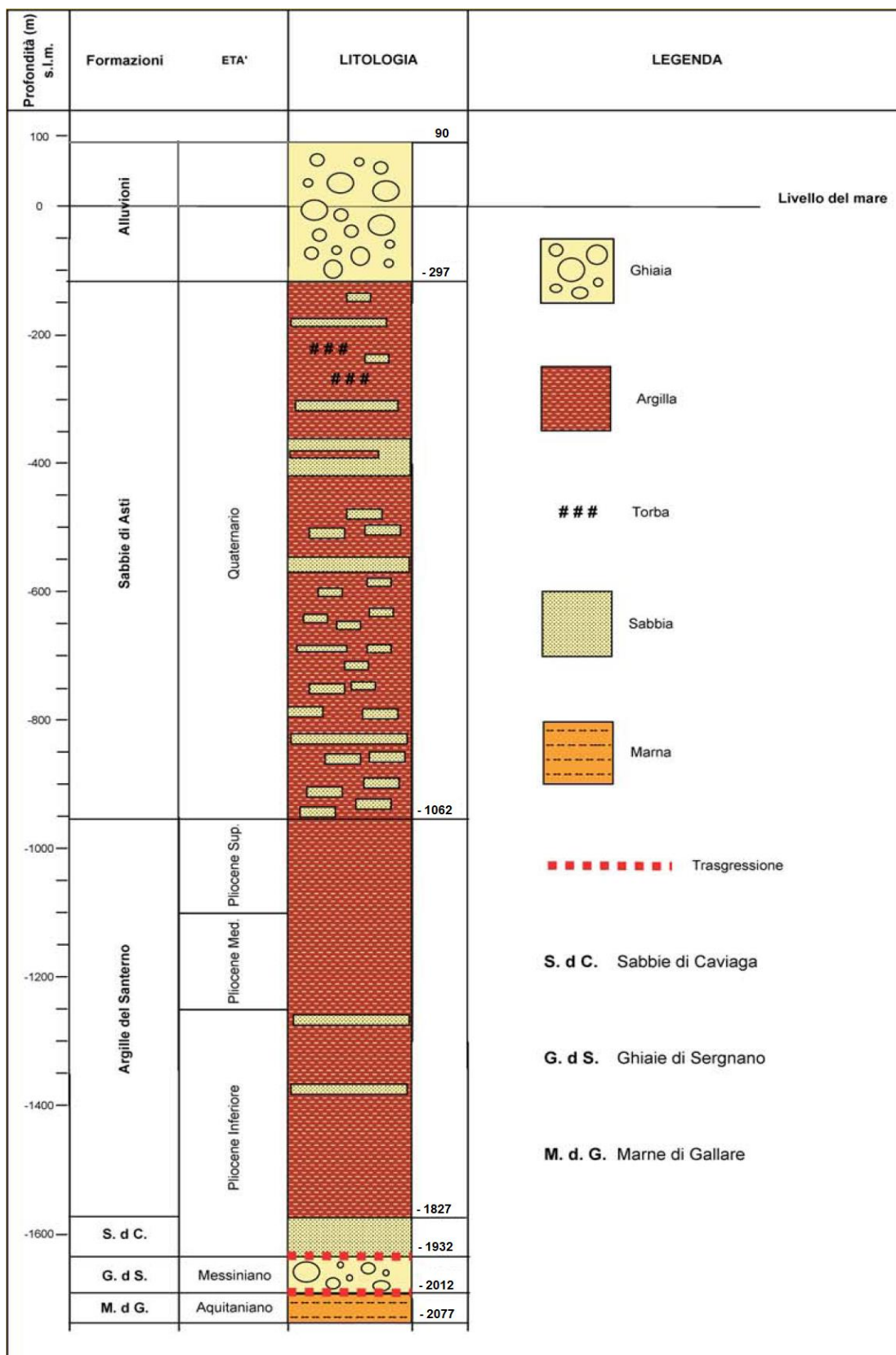
Figura 2.6 Stratigrafia terziaria-quadernaria del sondaggio Gallignano 02
