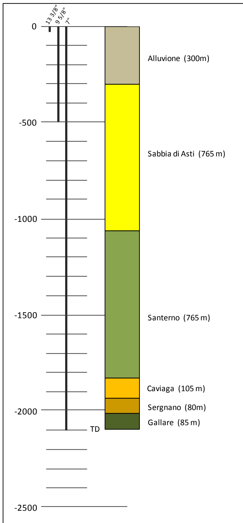
Figura 2.9. Profilo litostratigrafico previsto
