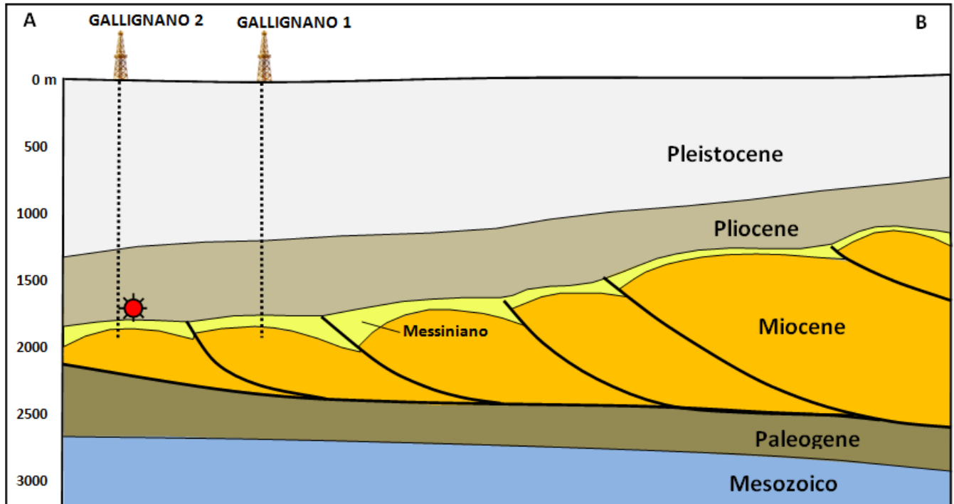
Figura 2.4 Sezione geologica schematica attraverso l'area del Permesso
