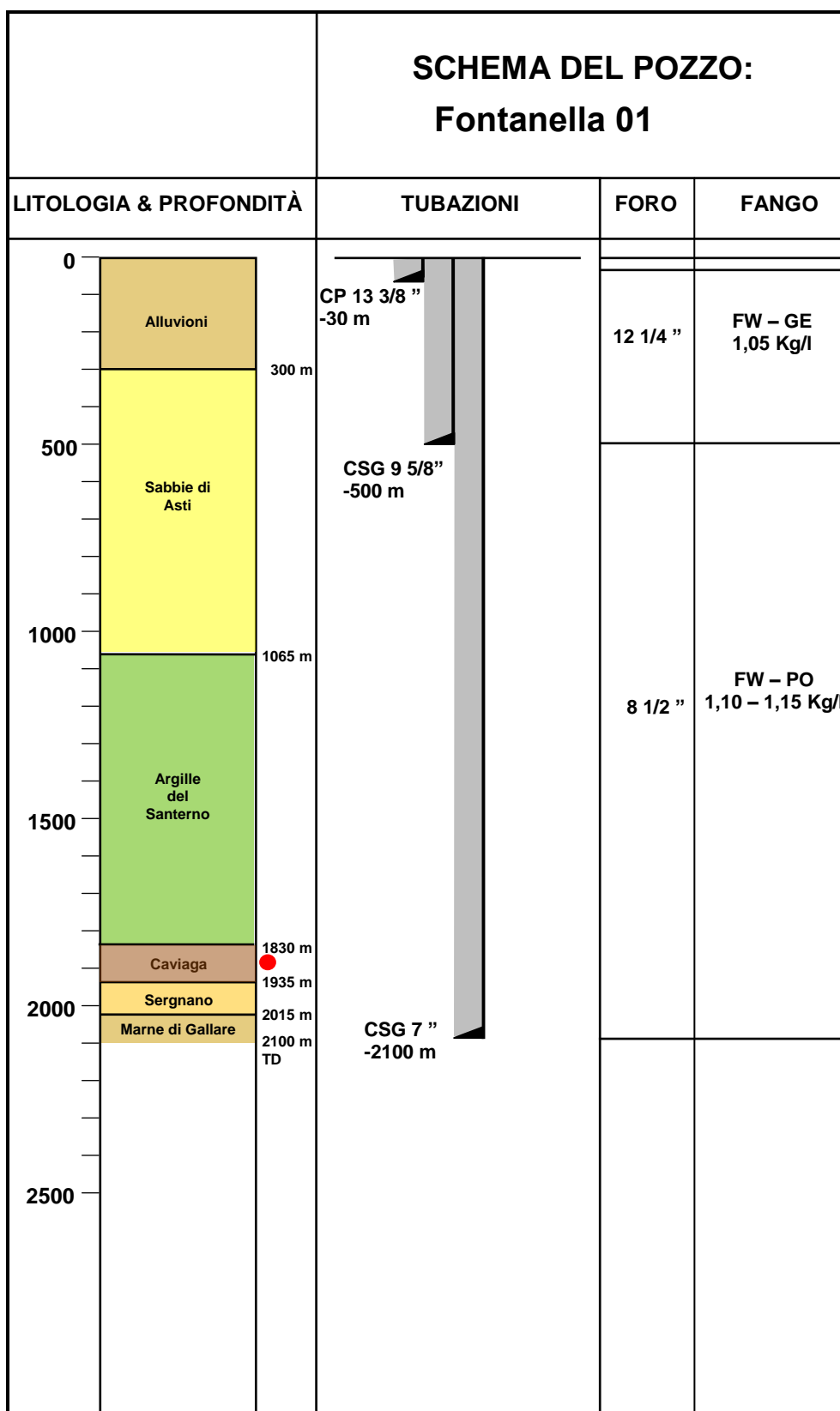
Figura 2.16 Schema del Pozzo
