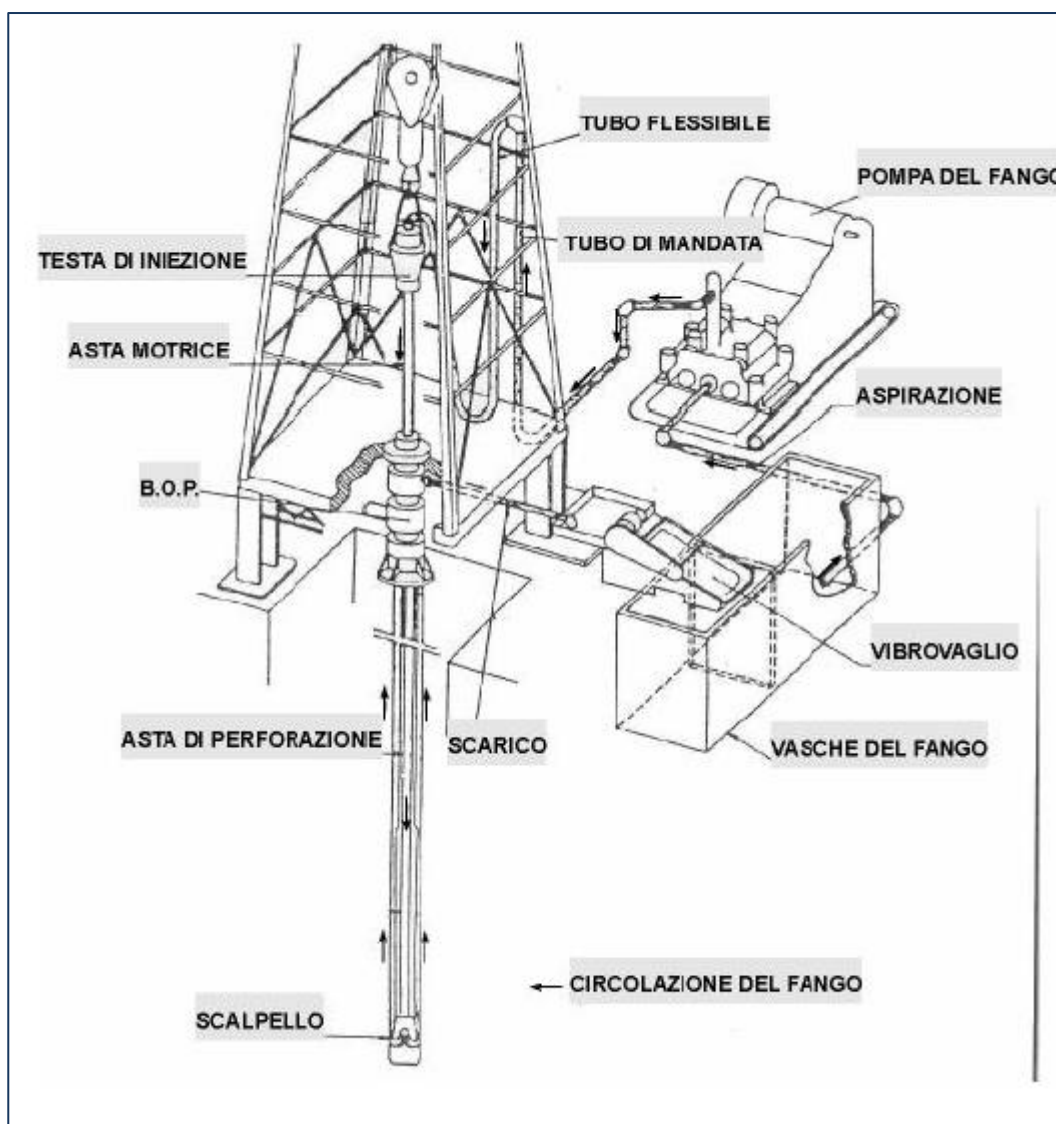
Fig. 2.13 Schema del circuito del fango
