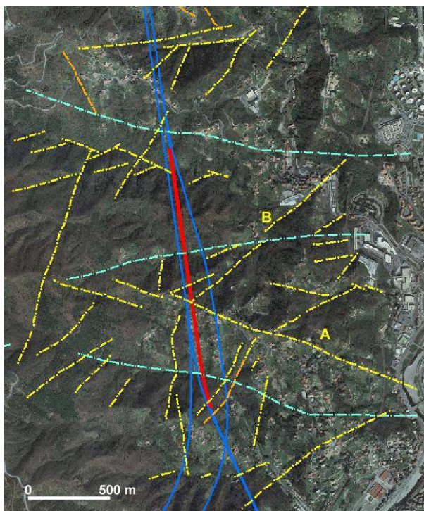
Figura 7 – Principali elementi strutturali lineari dell’area di studio; sulla destra il fondovalle del T. Polcevera.
