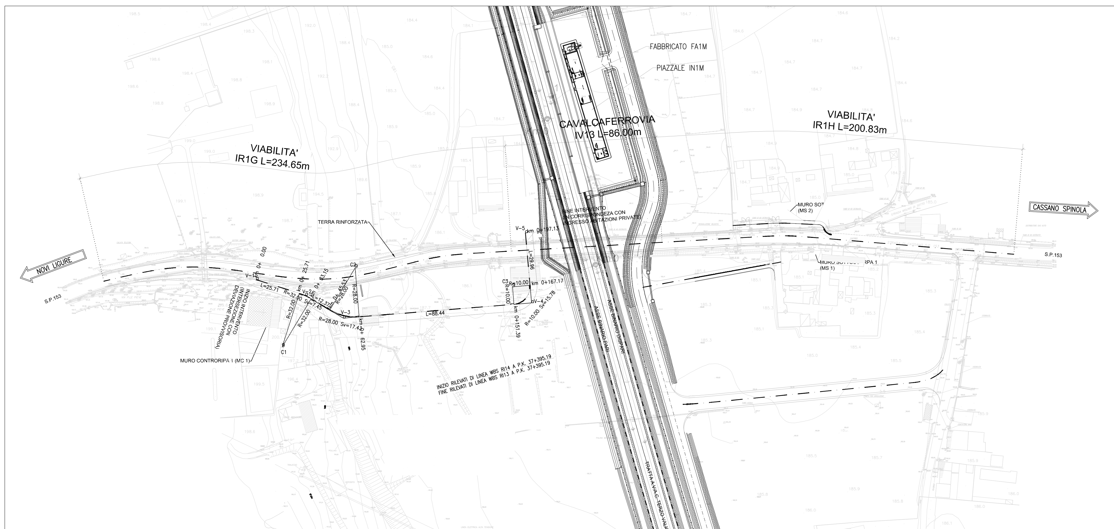
PLANIMETRIA DI TRACCIAMENTO STRADA ACCESSO ALLA 0+425 scala 1:1000
