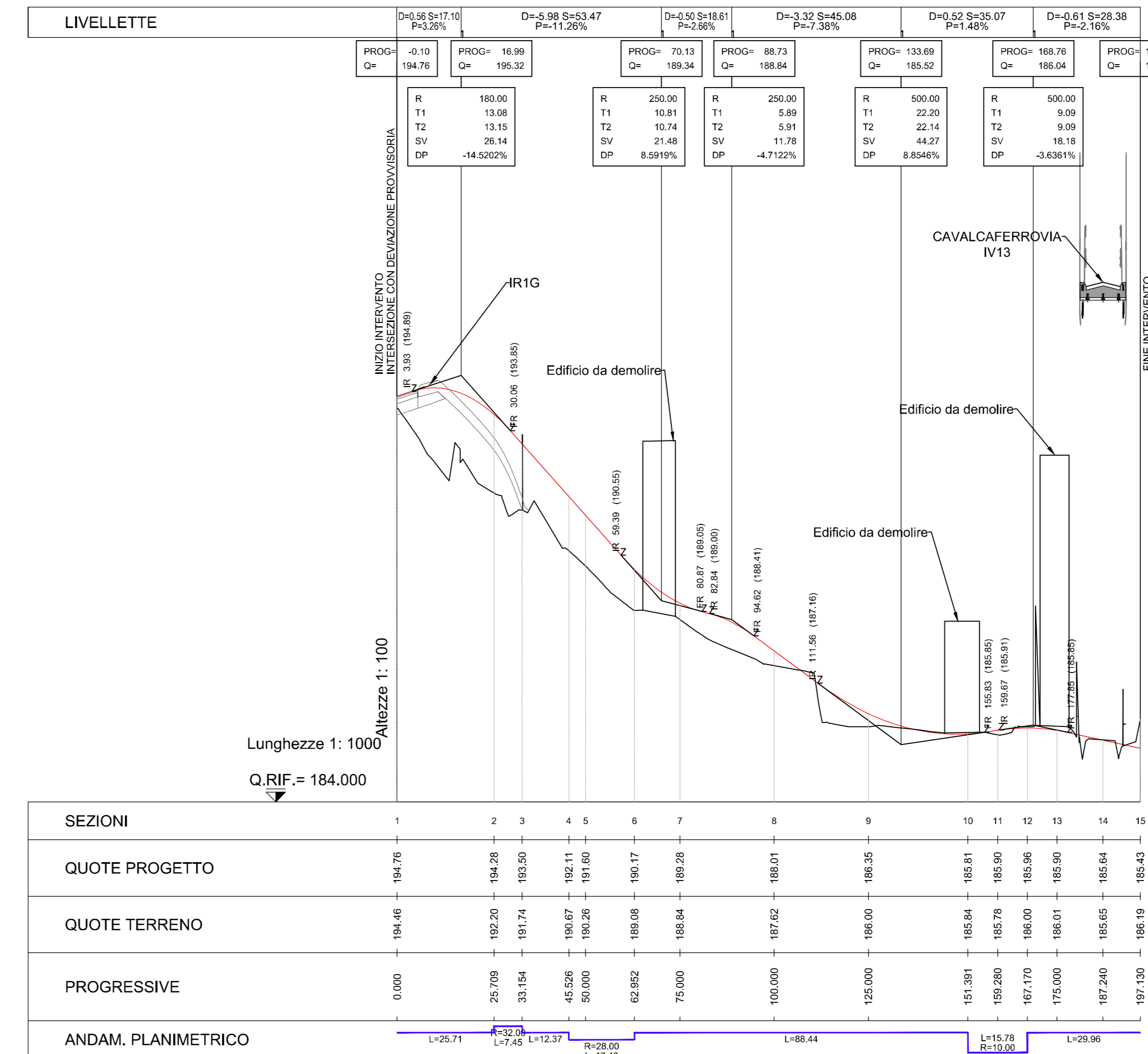
PROFLO LONGITUDINALE DI PROGETTO STRADA ACCESSO ALLA 0+425 scala 1:1000
