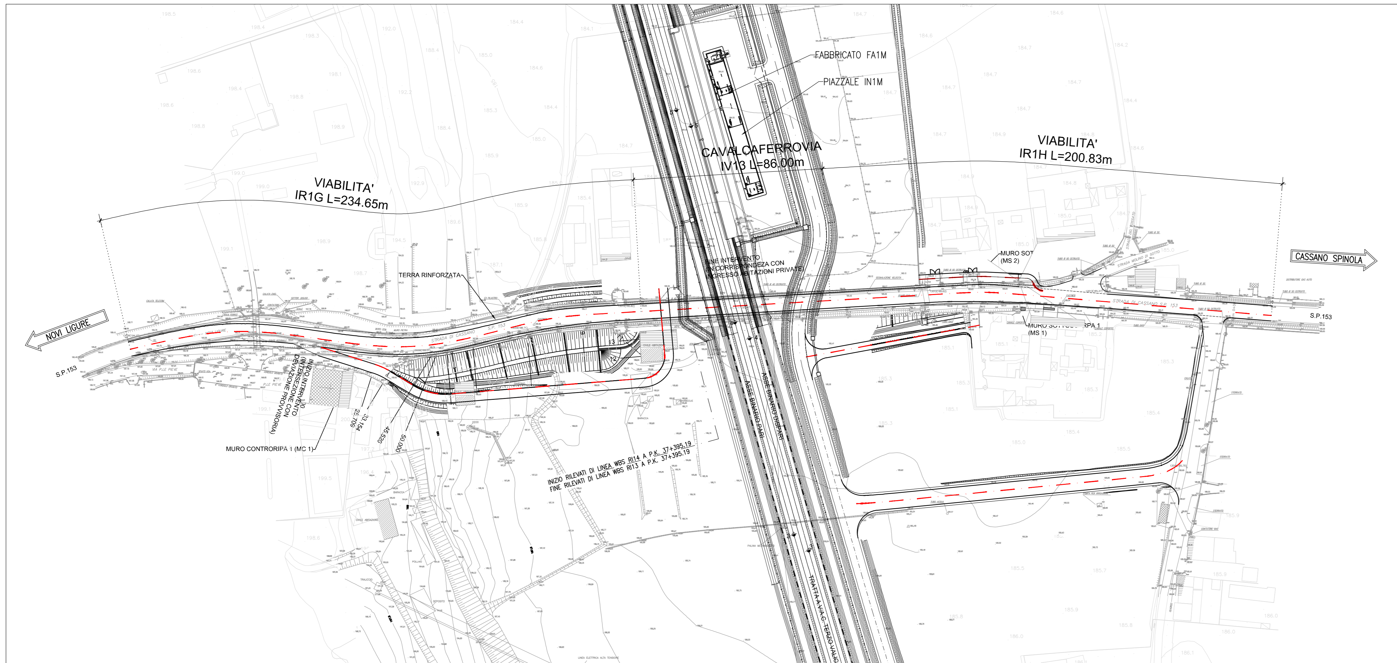
PLANIMETRIA DI PROGETTO STRADA ACCESSO ALLA 0+425 scala 1:1000
