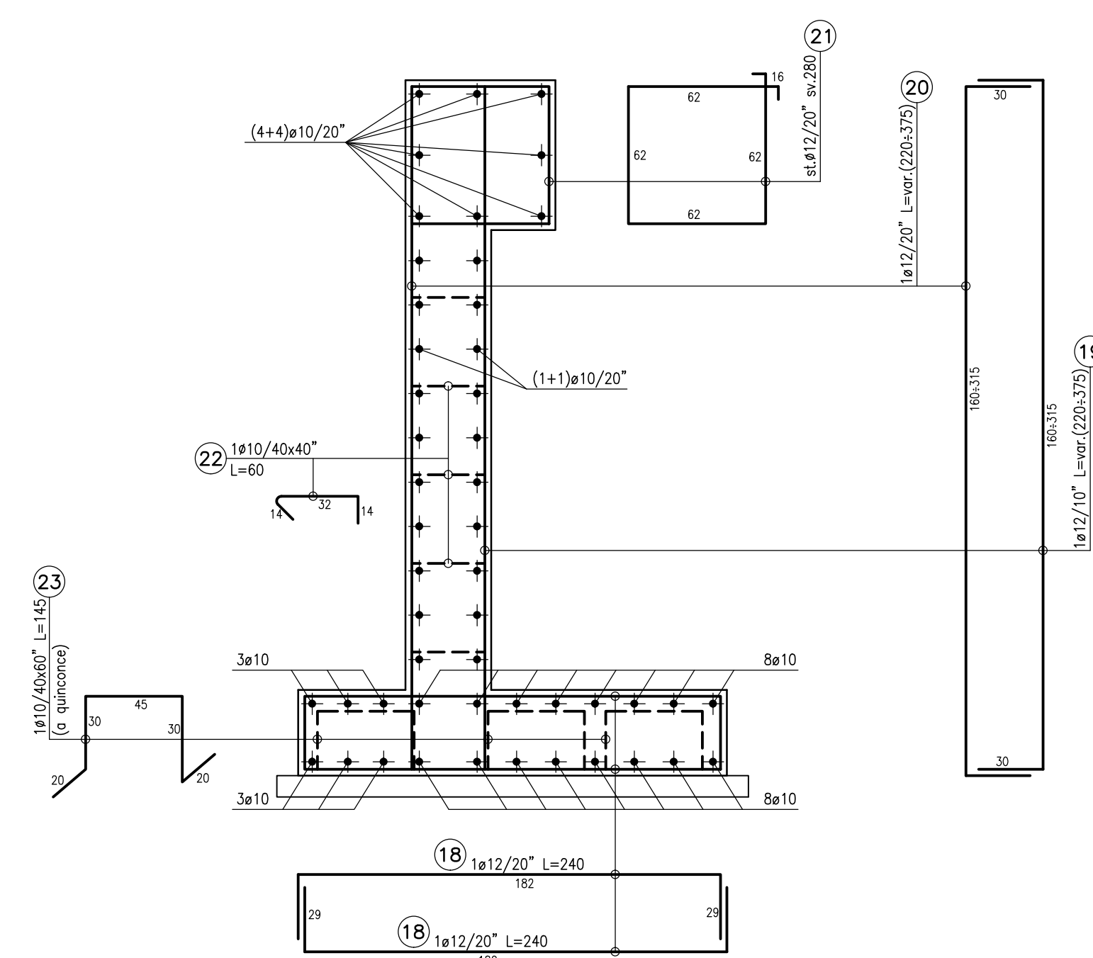
SEZIONE A-A scala 1:25
