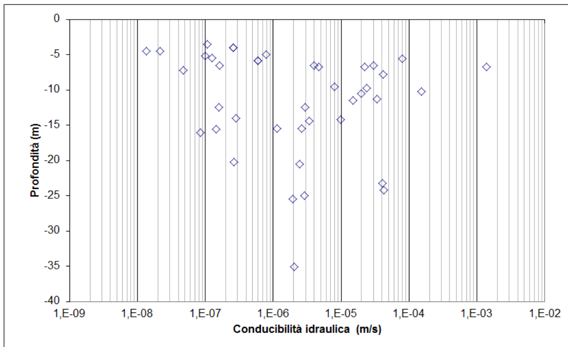
Figura 10. Grafico delle conducibilità idrauliche per i depositi alluvionali medi (fl2).
