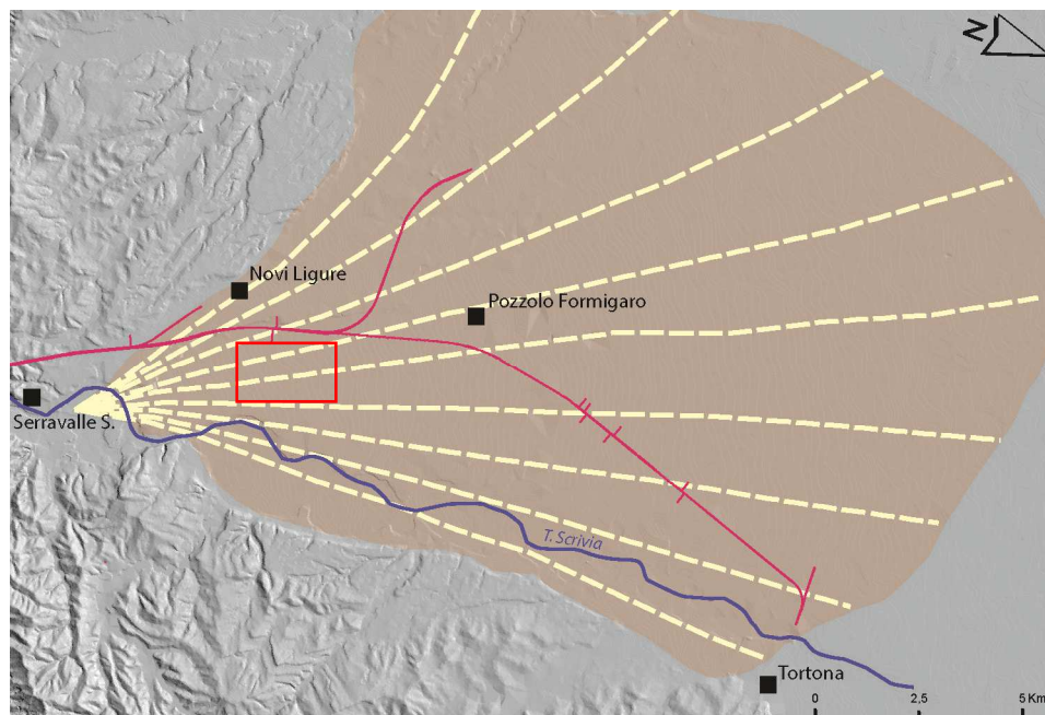
Figura 8 - Rappresentazione schematica dell'estensione areale del conoide del T. Scivia, dei vari ordini di terrazzi da cui esso è disseccato. Il quadrato rosso indica la posizione dell'opera in progetto.
